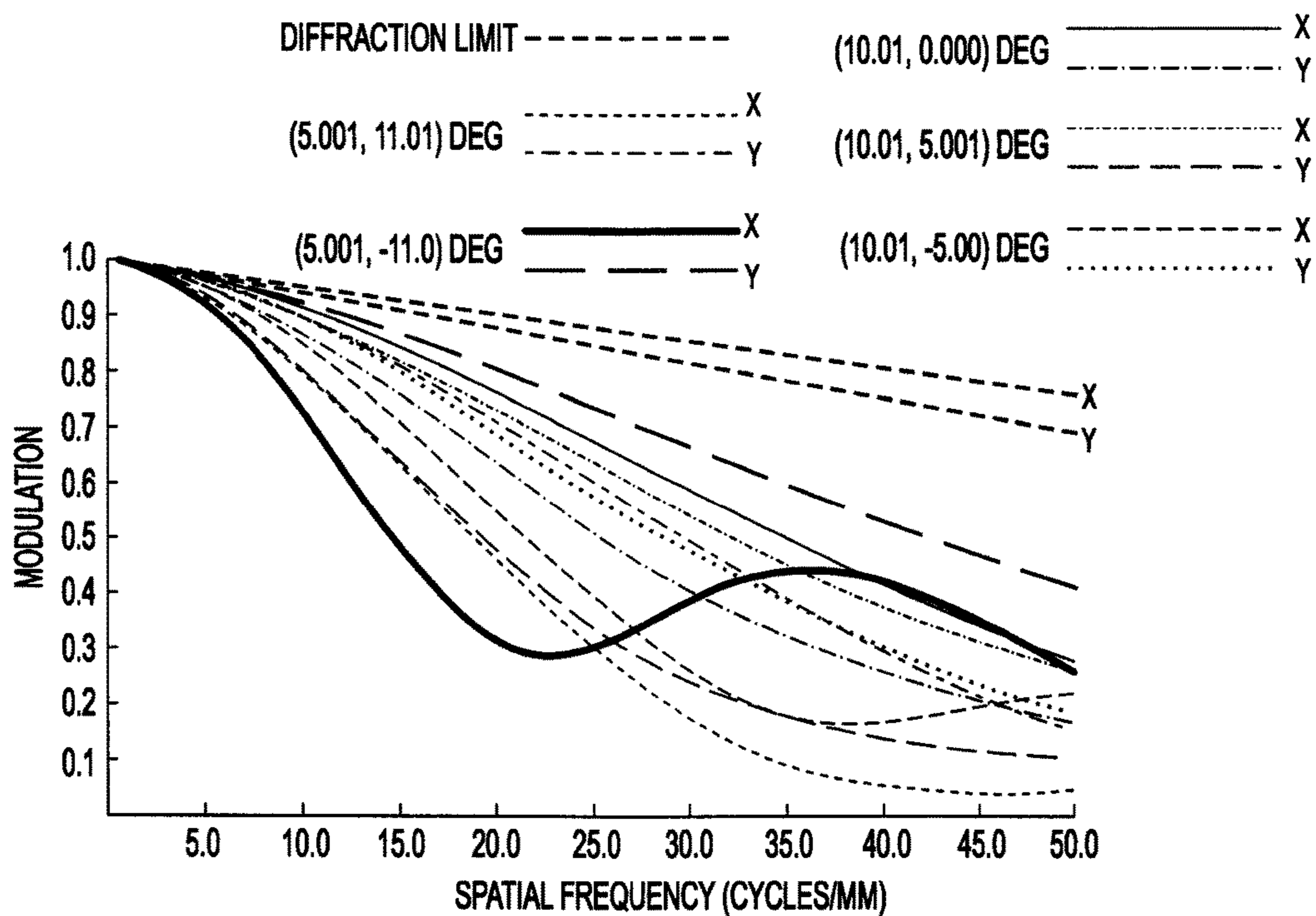
FIG. 9B
