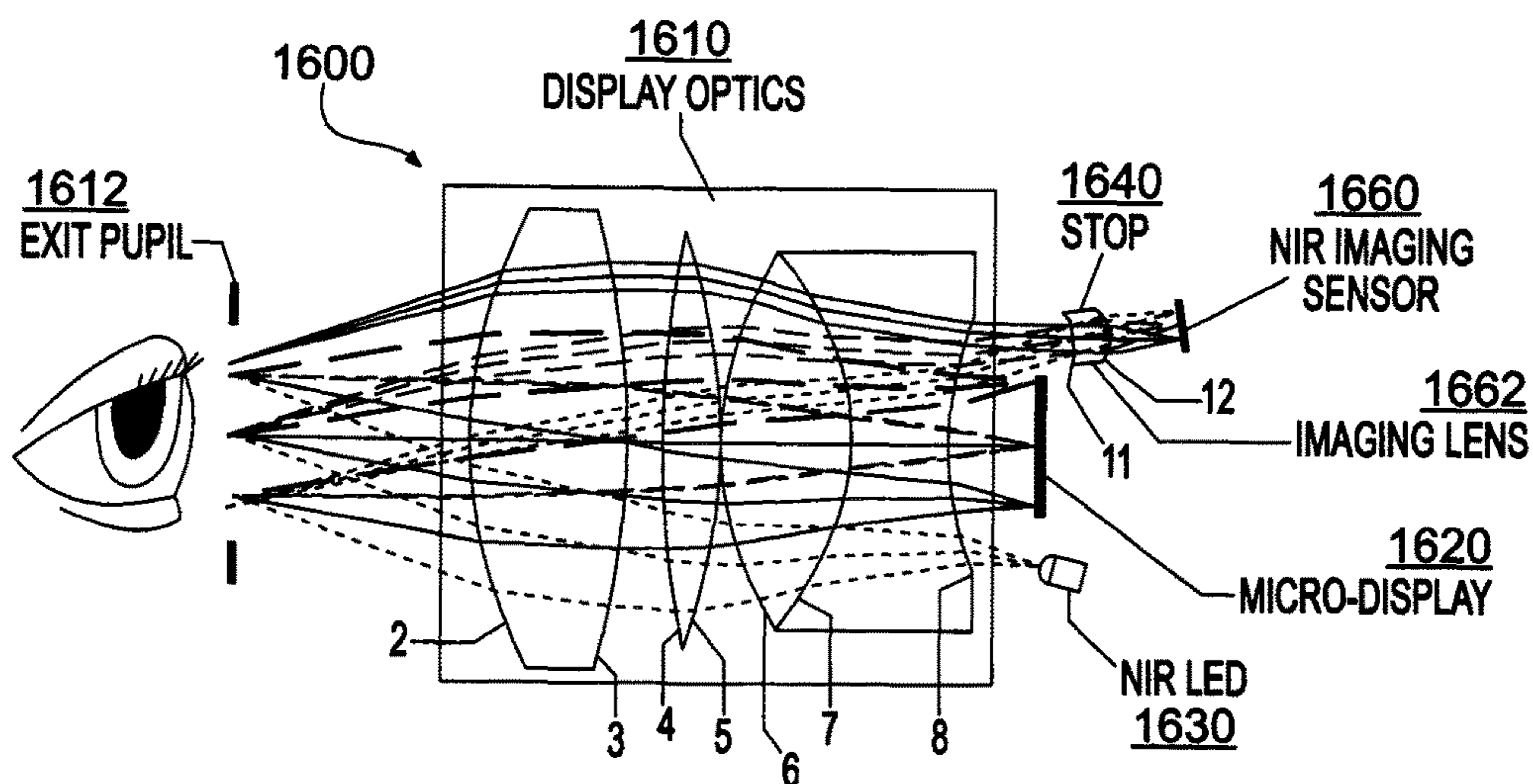
FIG. 16
