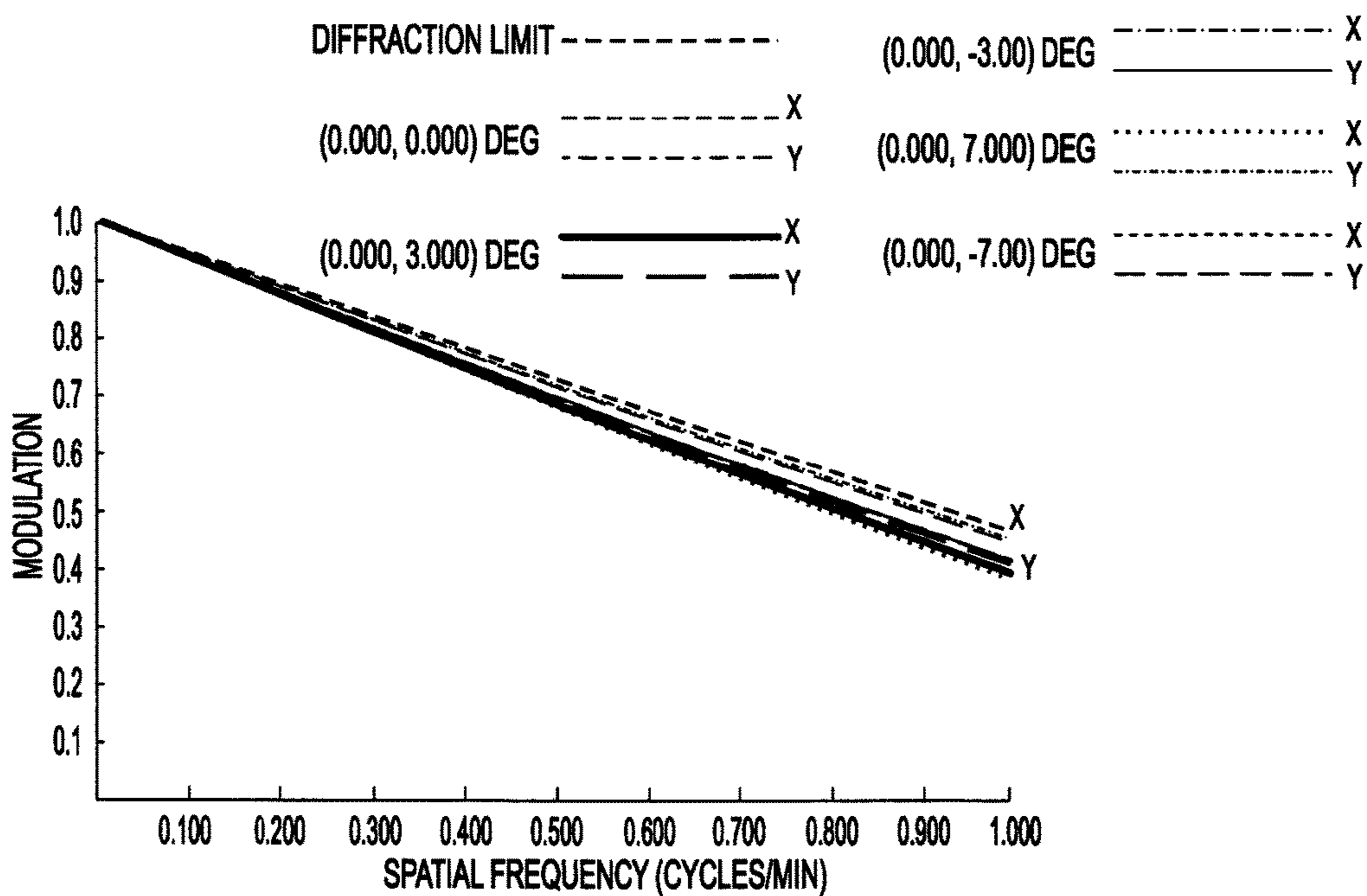
FIG. 13A
