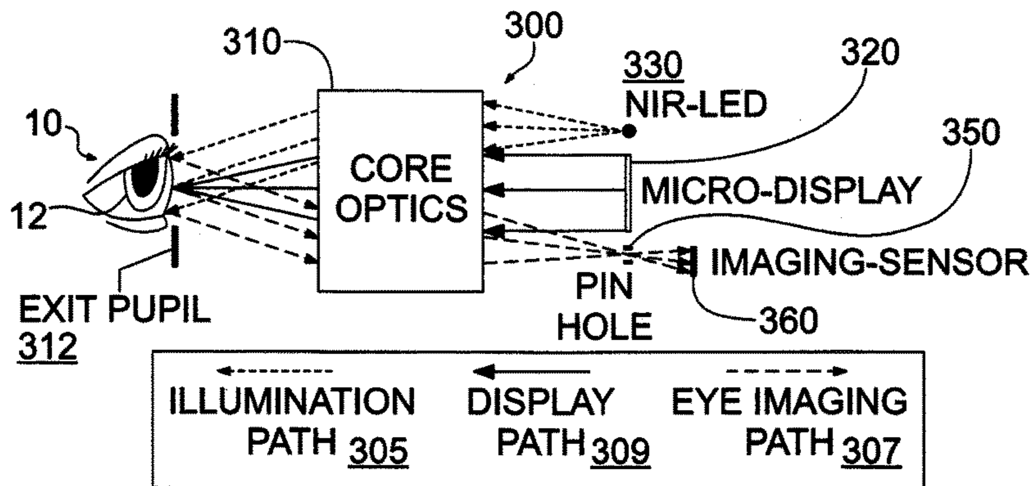
FIG. 3A
