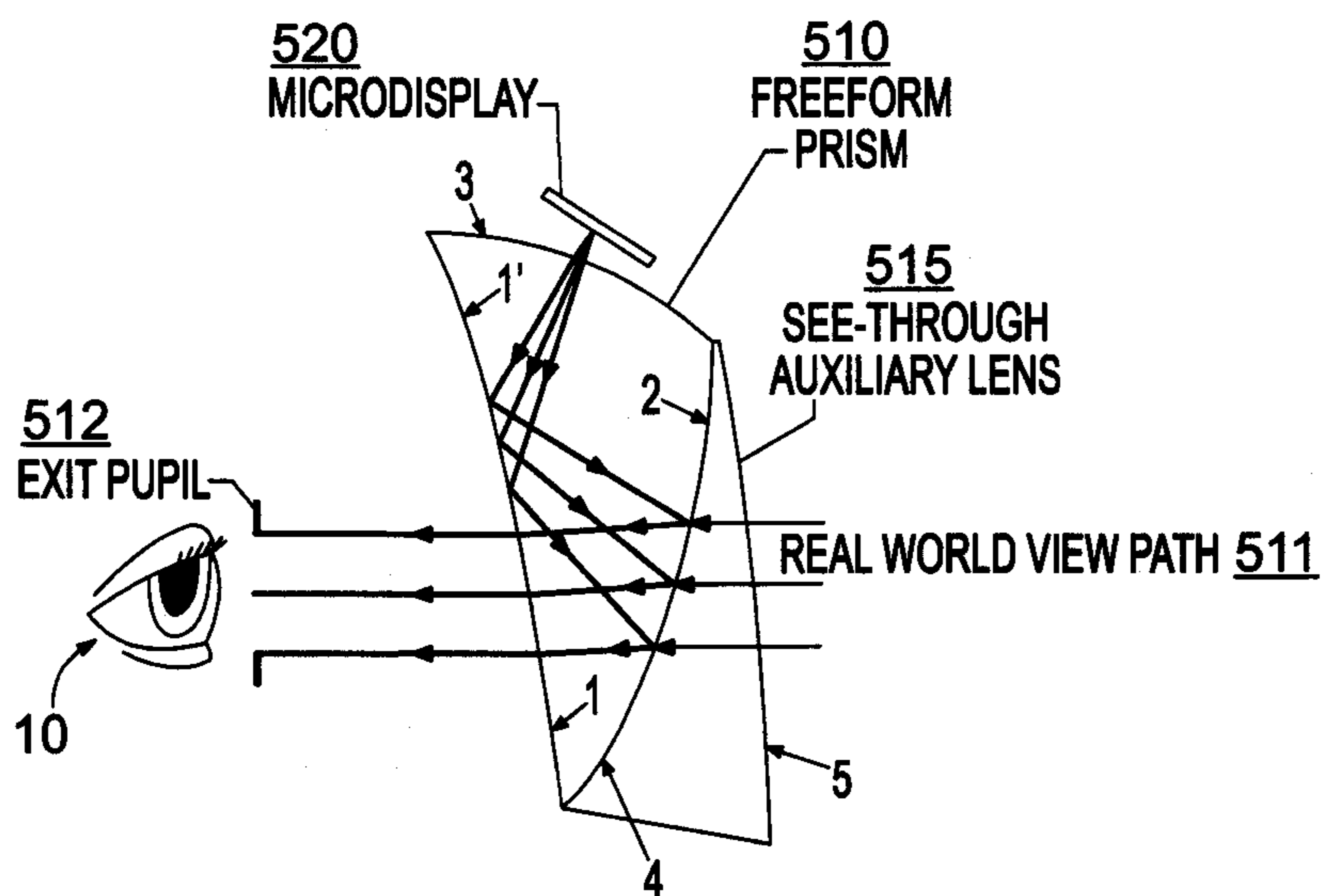
FIG. 5D
