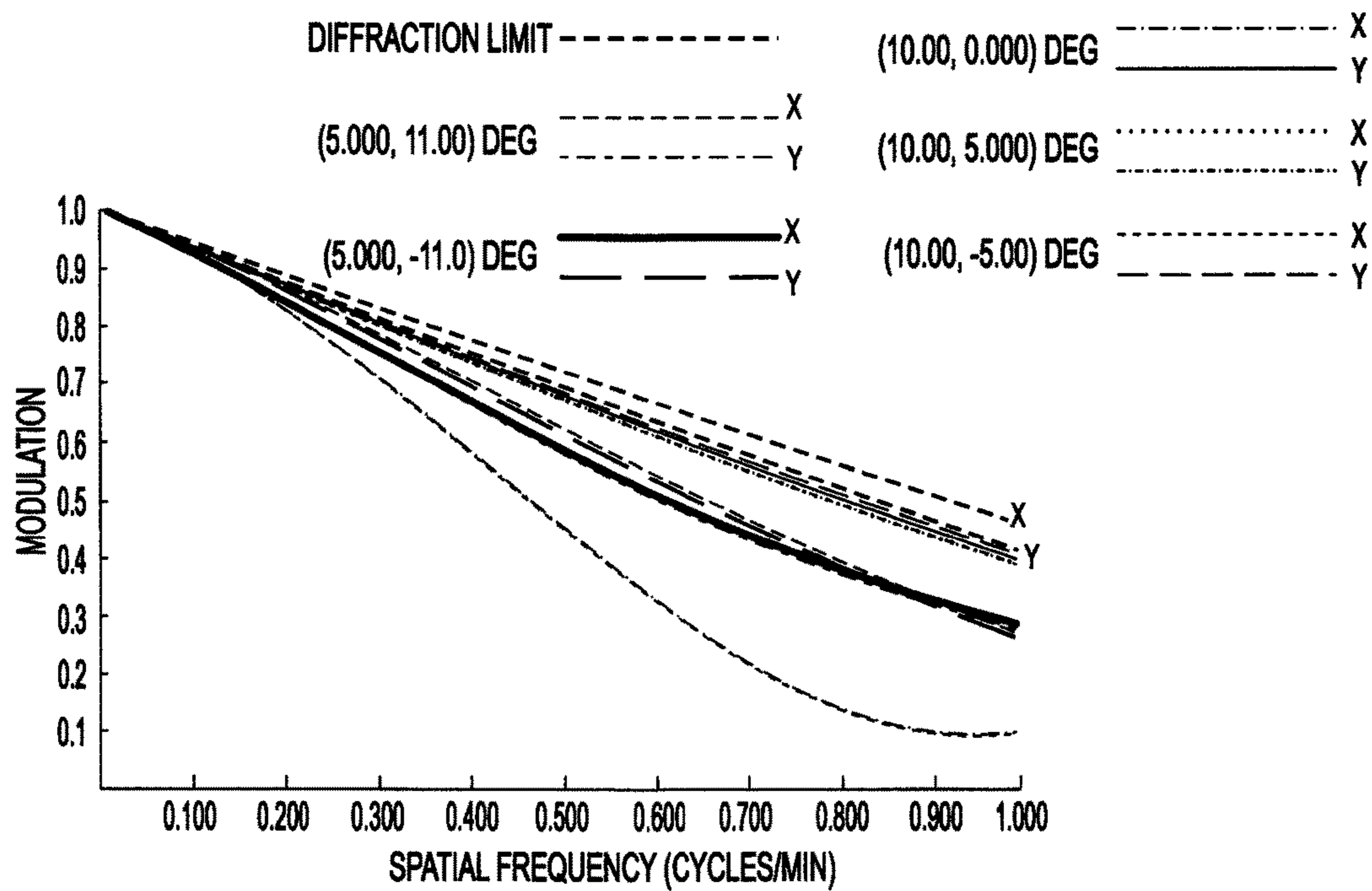
FIG. 13C
