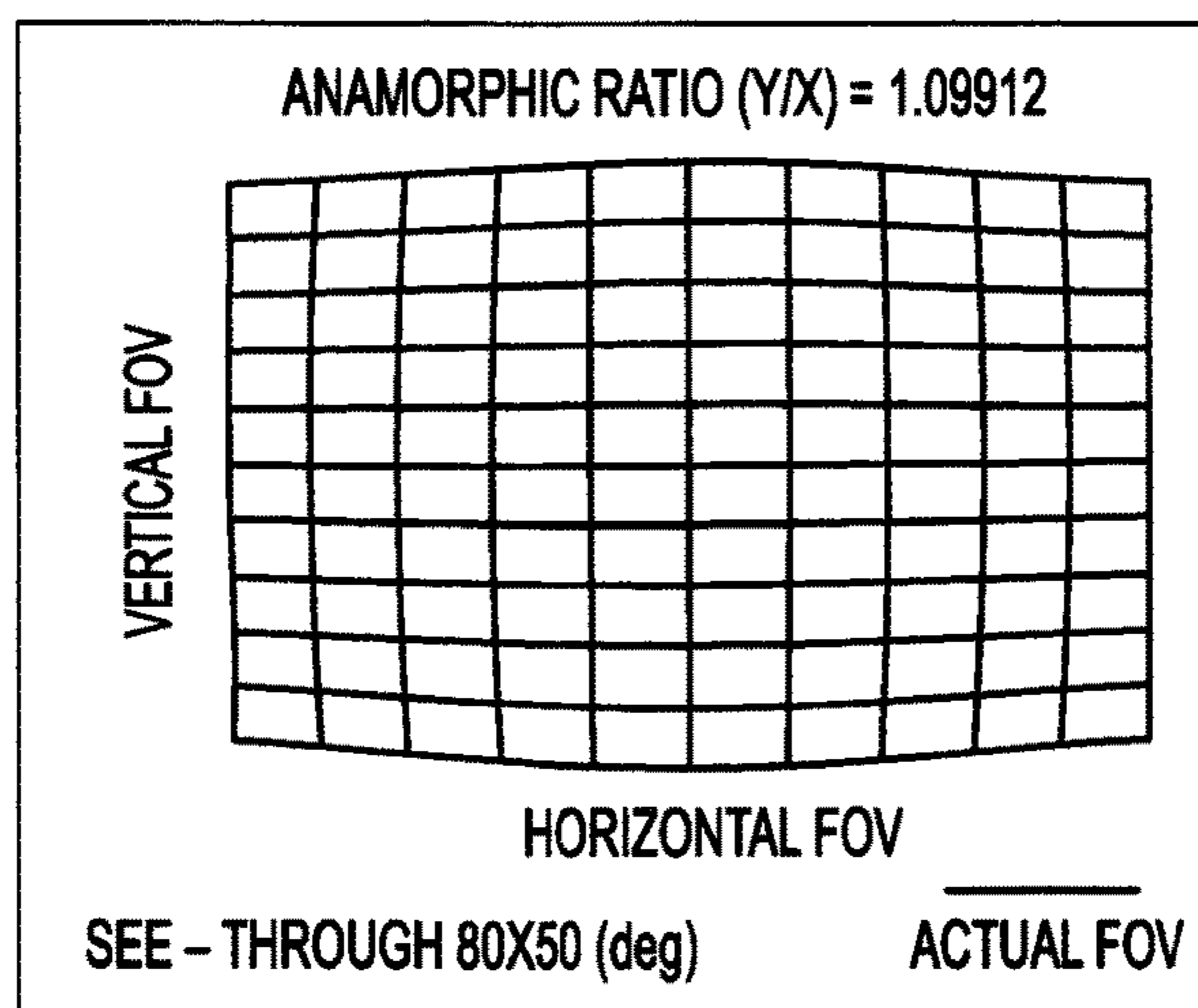
FIG. 14
