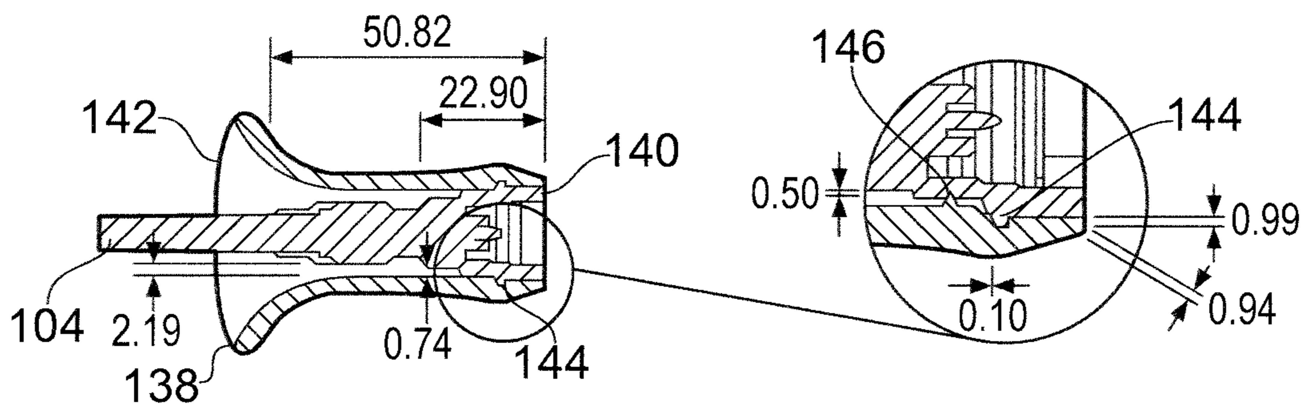
SECTION A-A FIG. 3C
