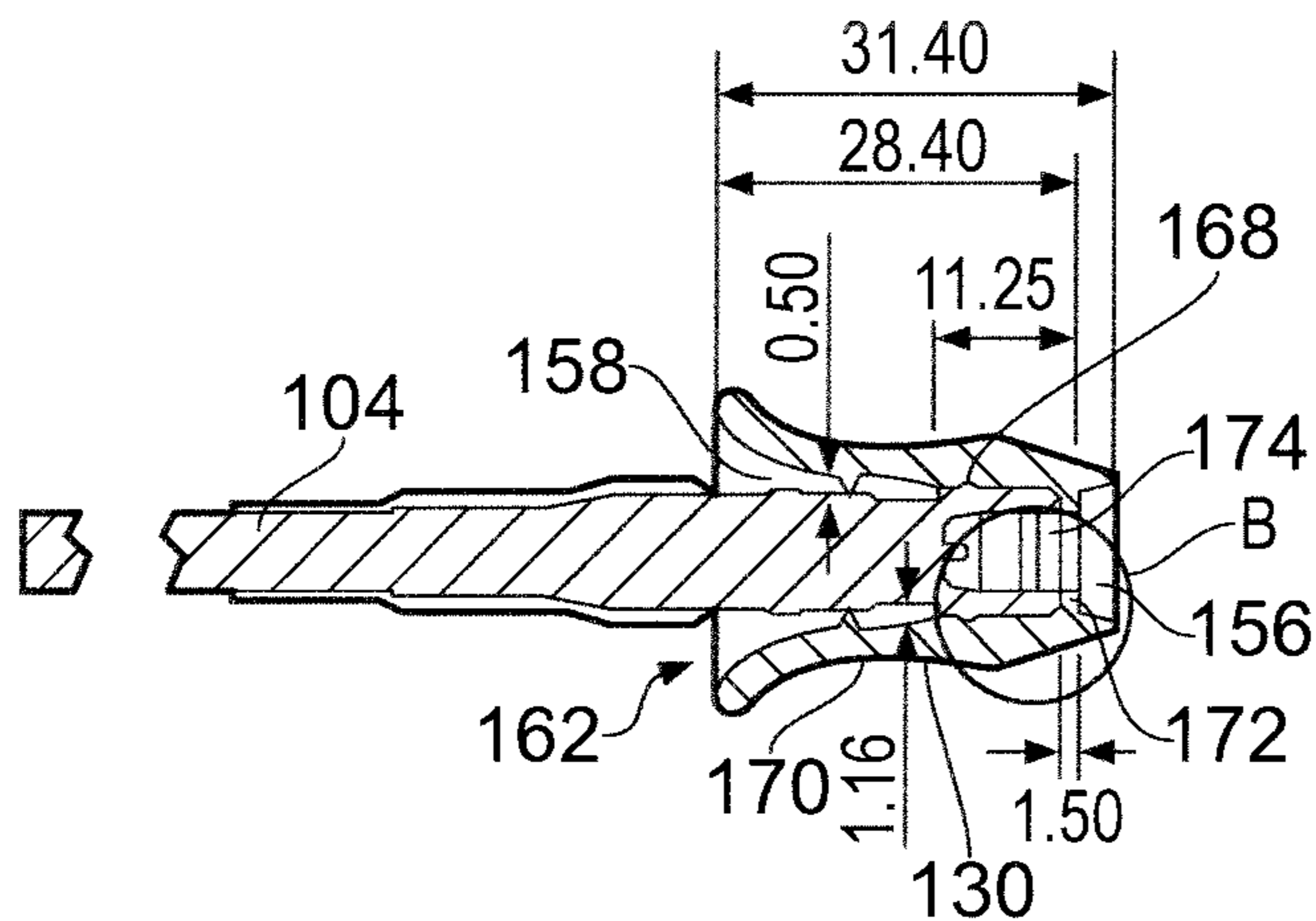
SECTION A-A
