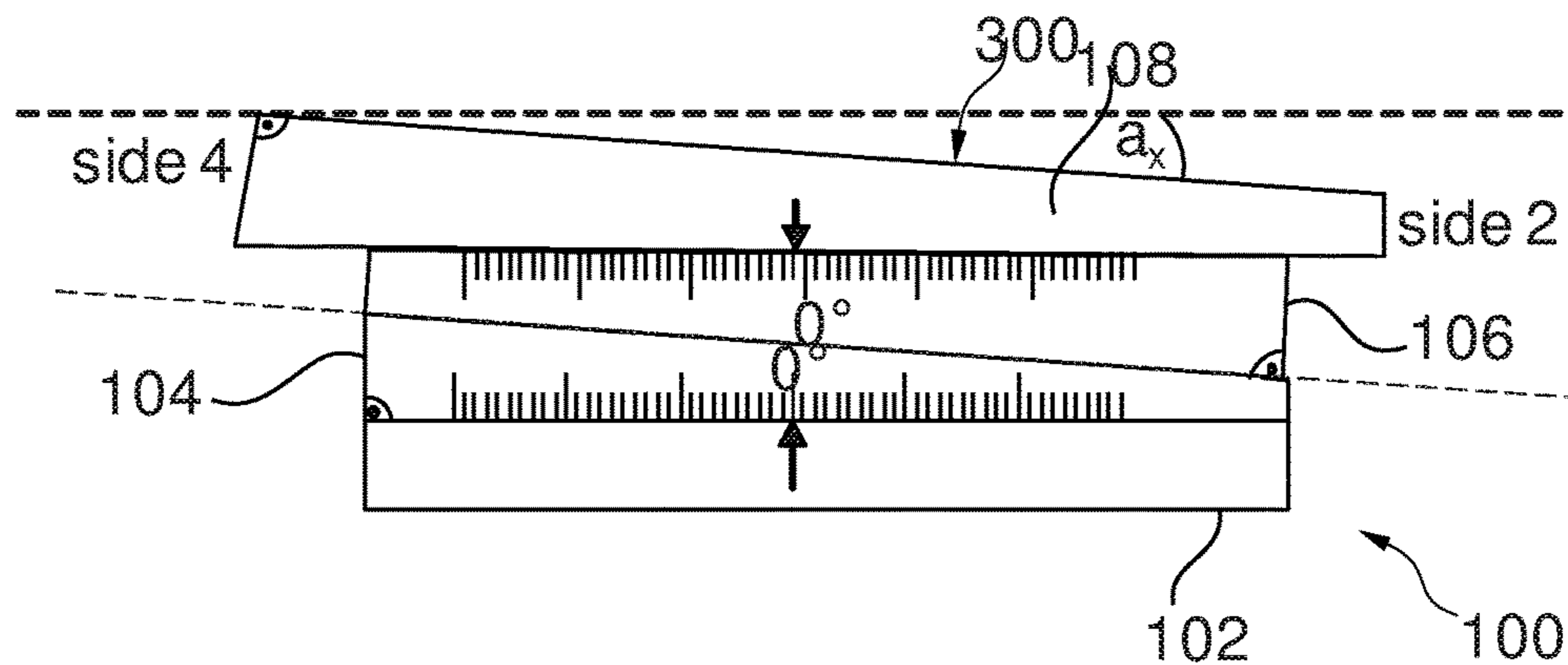
Fig. 7A
