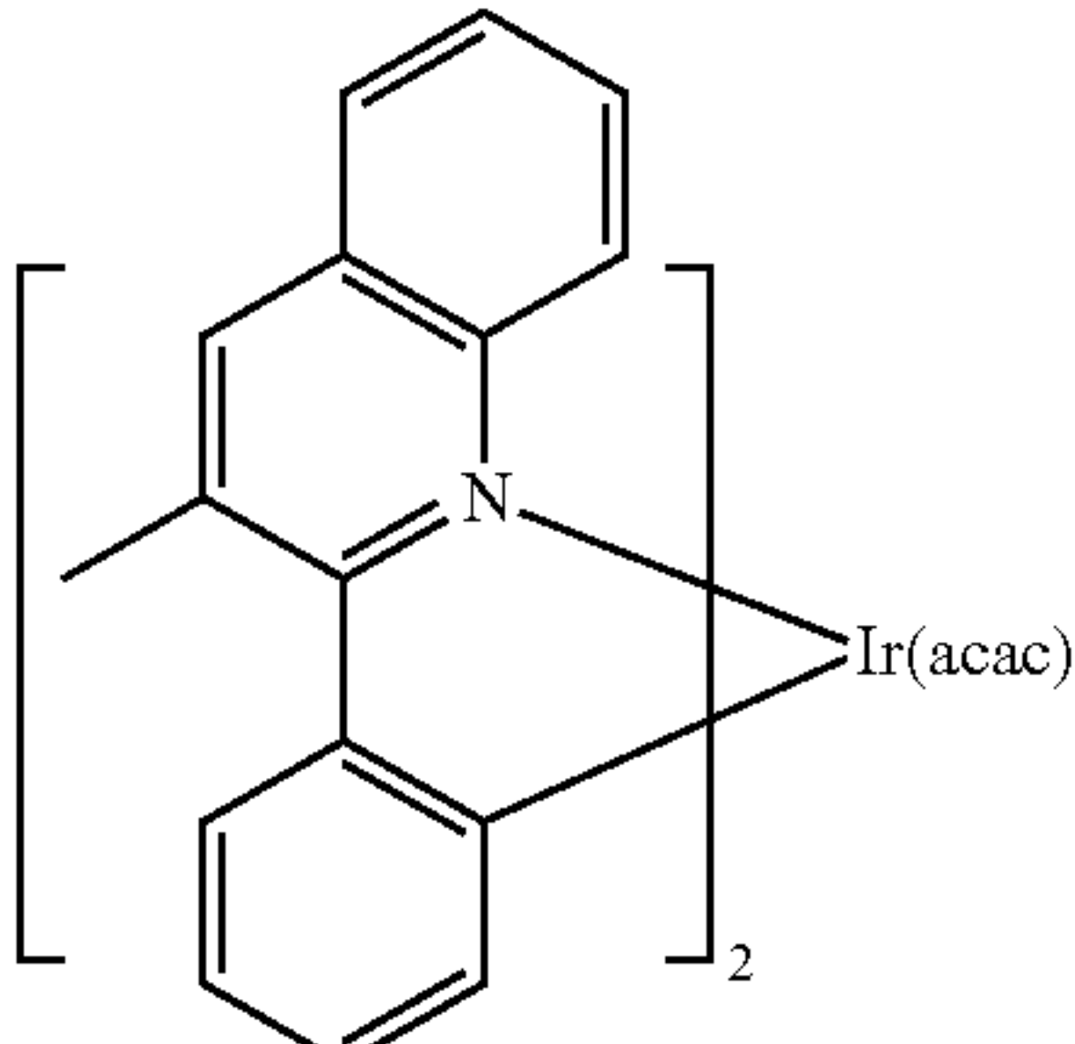
Ir(3-Mepq) 2 (acac)
