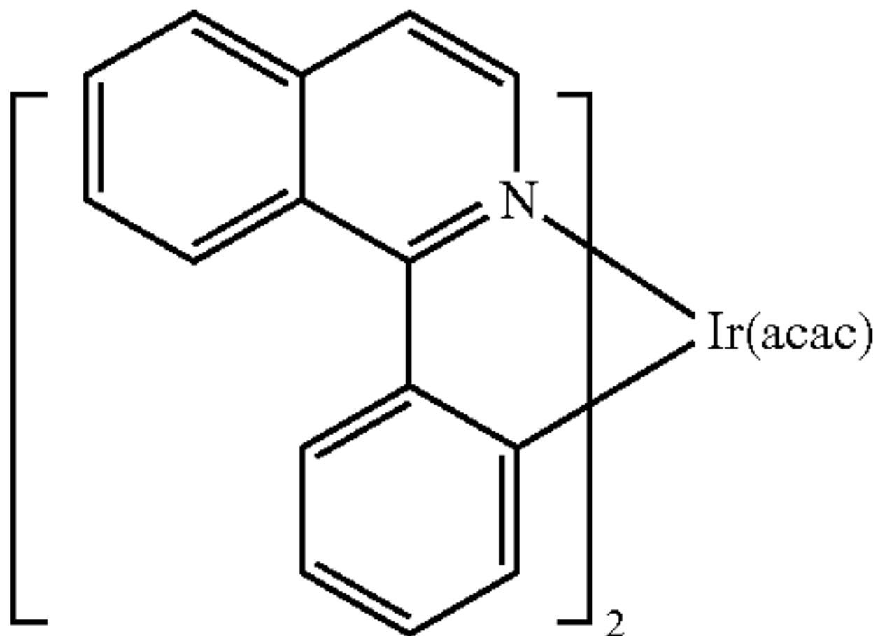
Ir(piq) 2 (acac)
