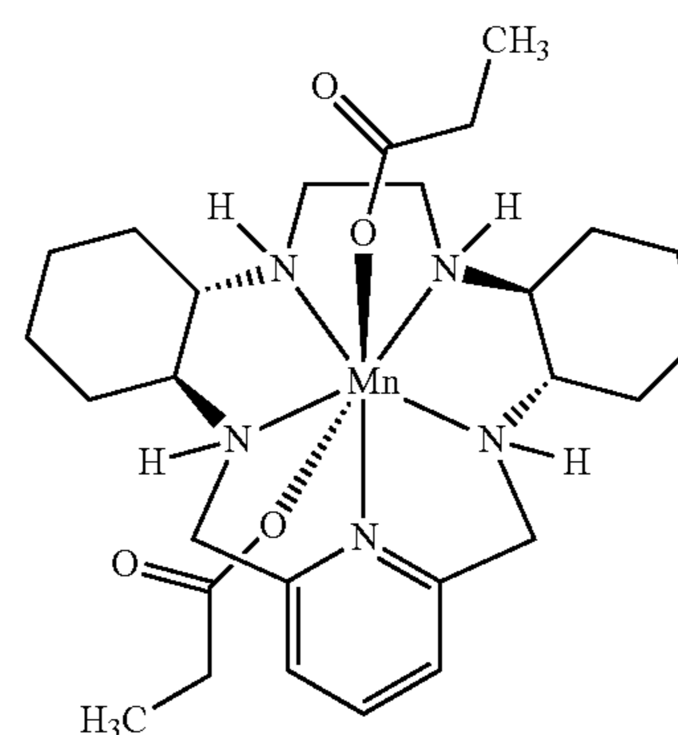
[Bis-Propionato(GC4419)] C_{27}H_{45}MnN_5O_4 MW 558.63
