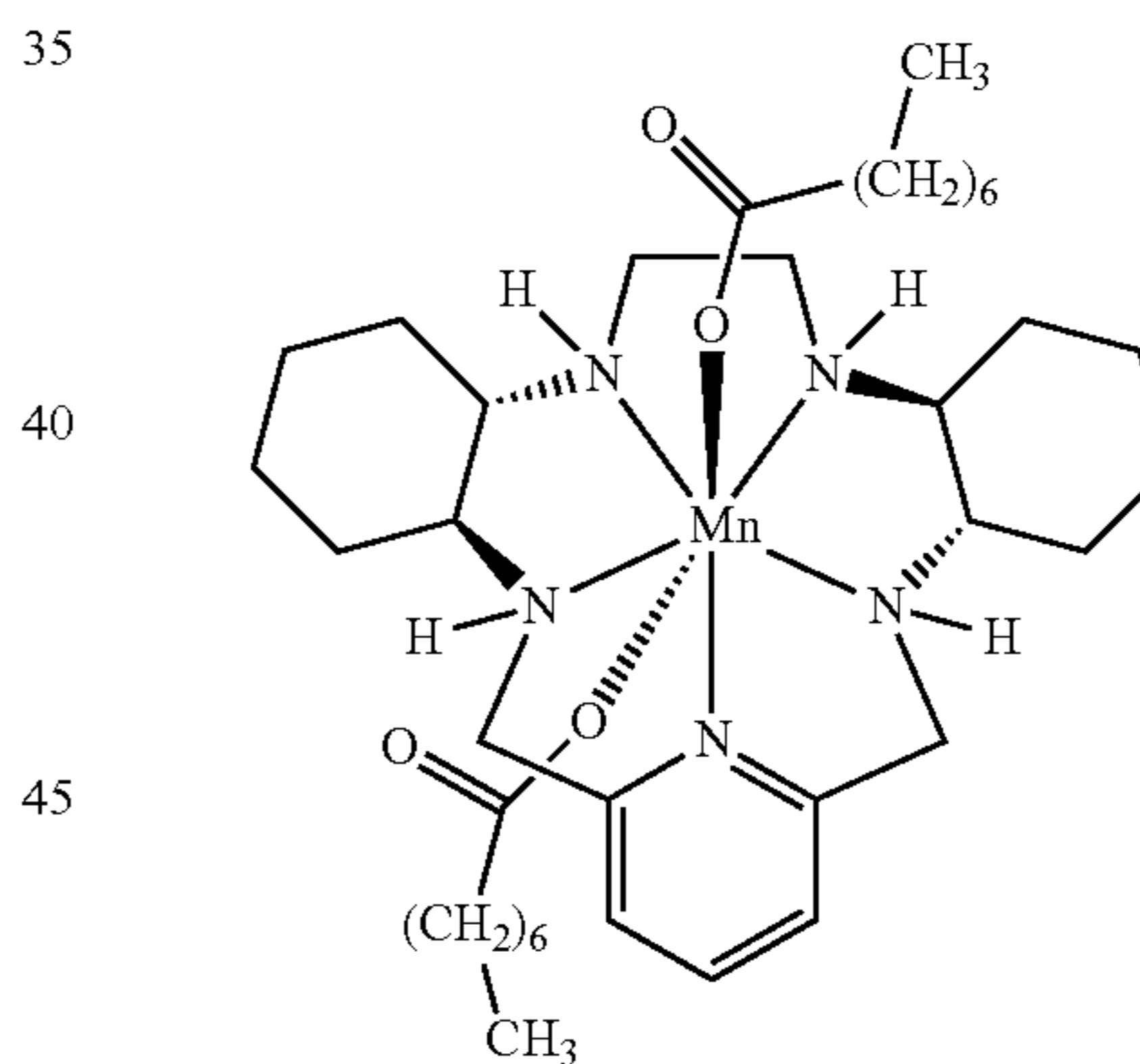
[Bis-Octanoato(GC4419)] C 37 H 65 MnN 5 O 4 MW 698.90
