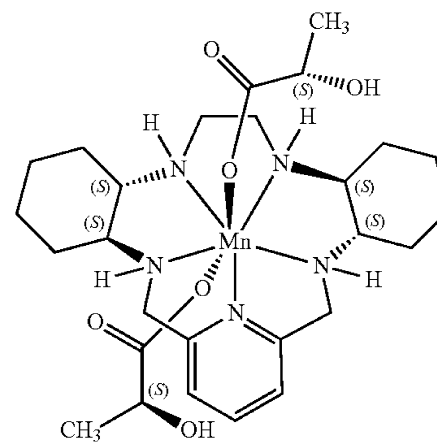
C 27 H 45 MnN 5 O 6 MW 590.62
