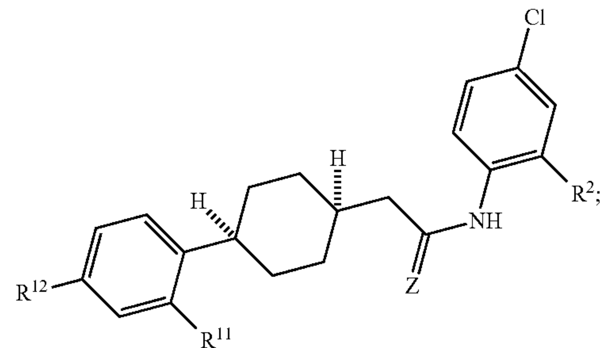
Formula (LIVz)
