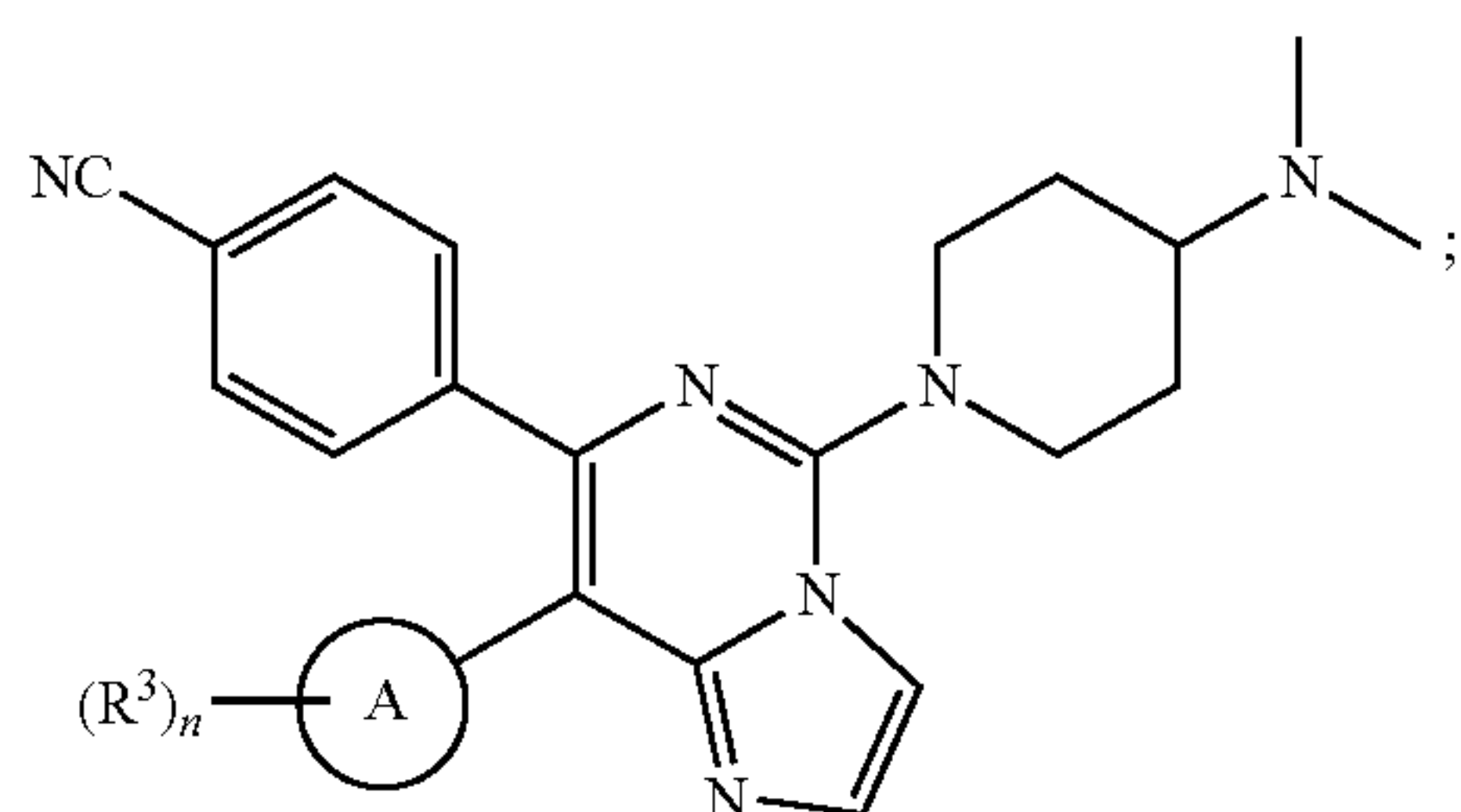
Formula (XVIIIIn)
