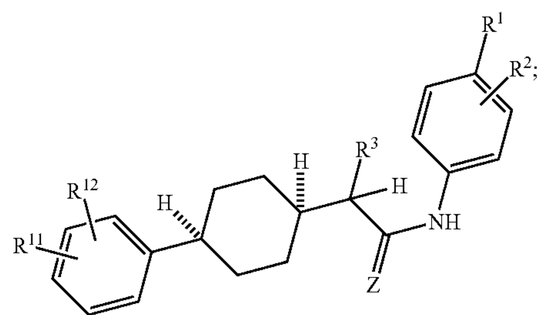
Formula (LIVp)
