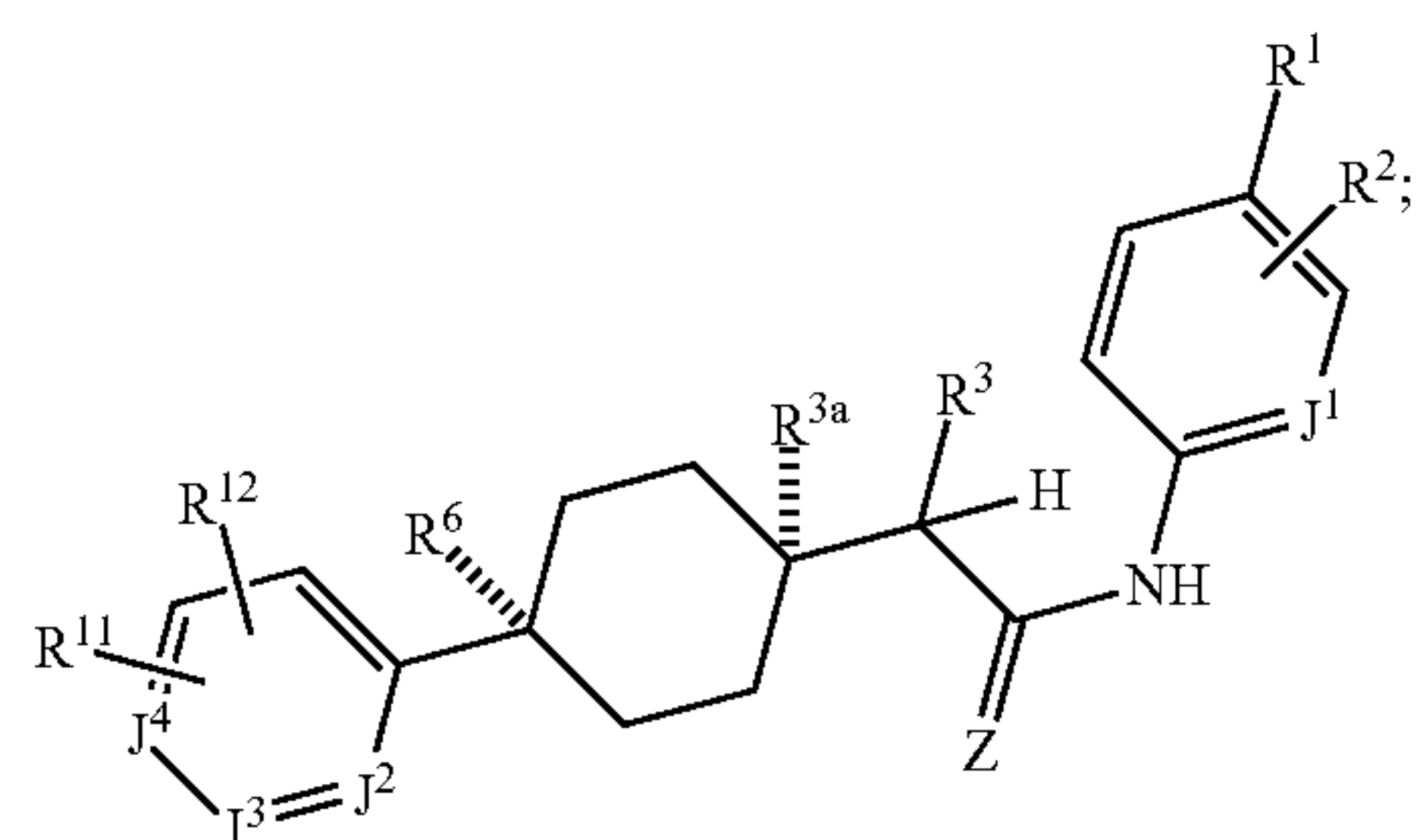
Formula (LIVn)
