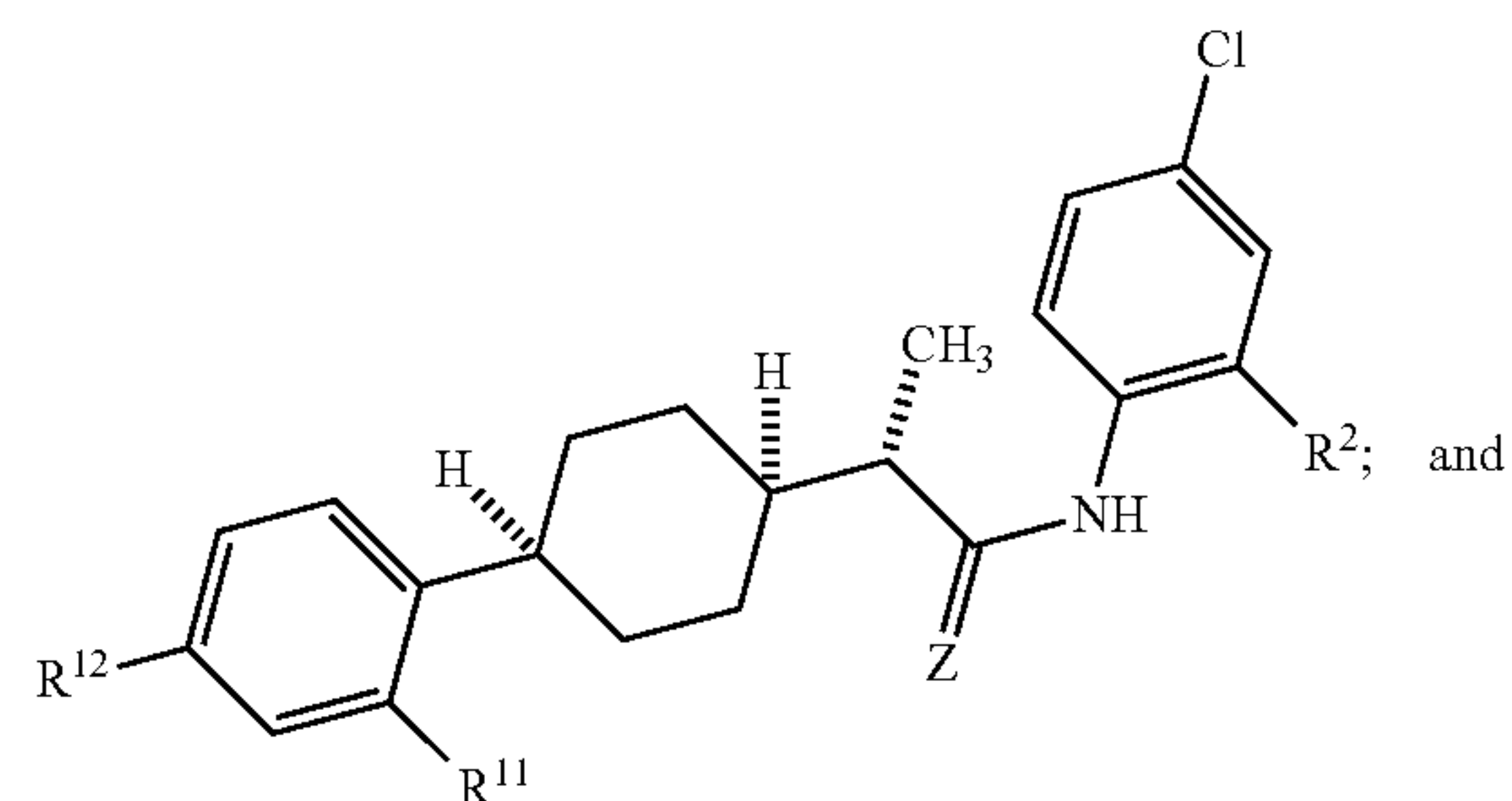
Formula (LIVaa)
