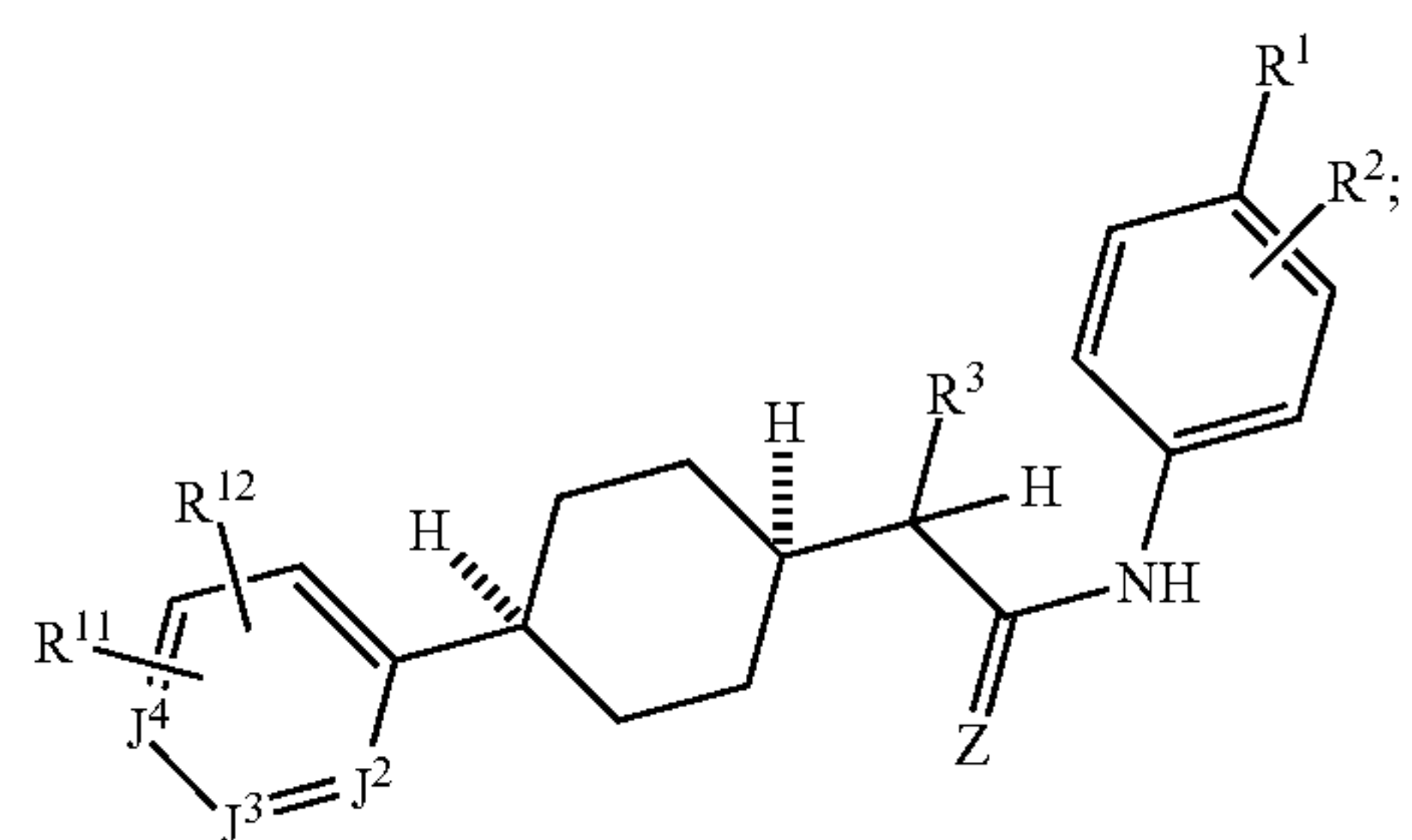
Formula (LIVo)
