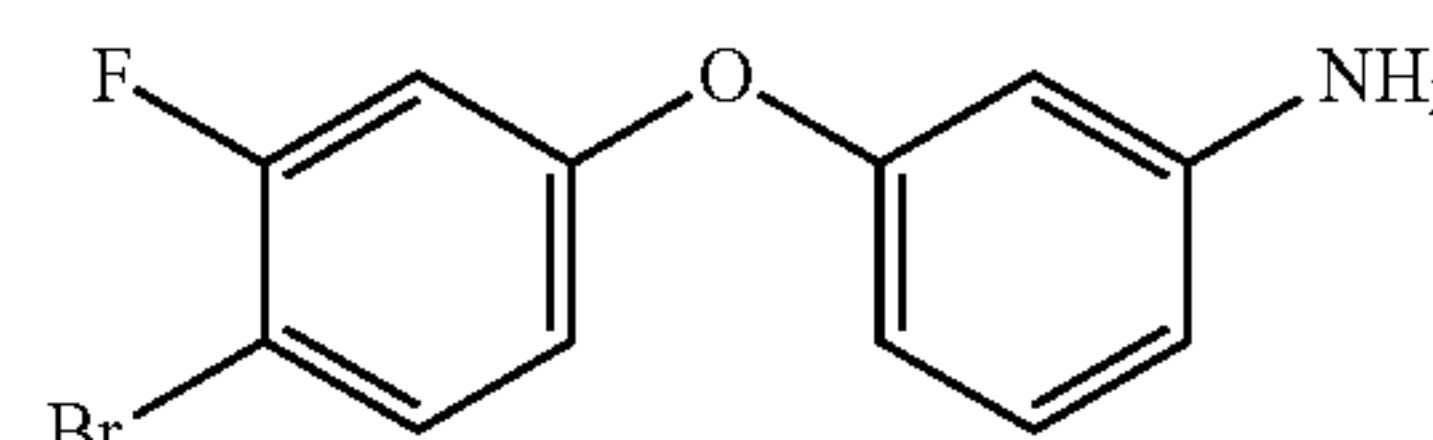
3-(4-bromo-3-fluorophenoxy)benzenamine
