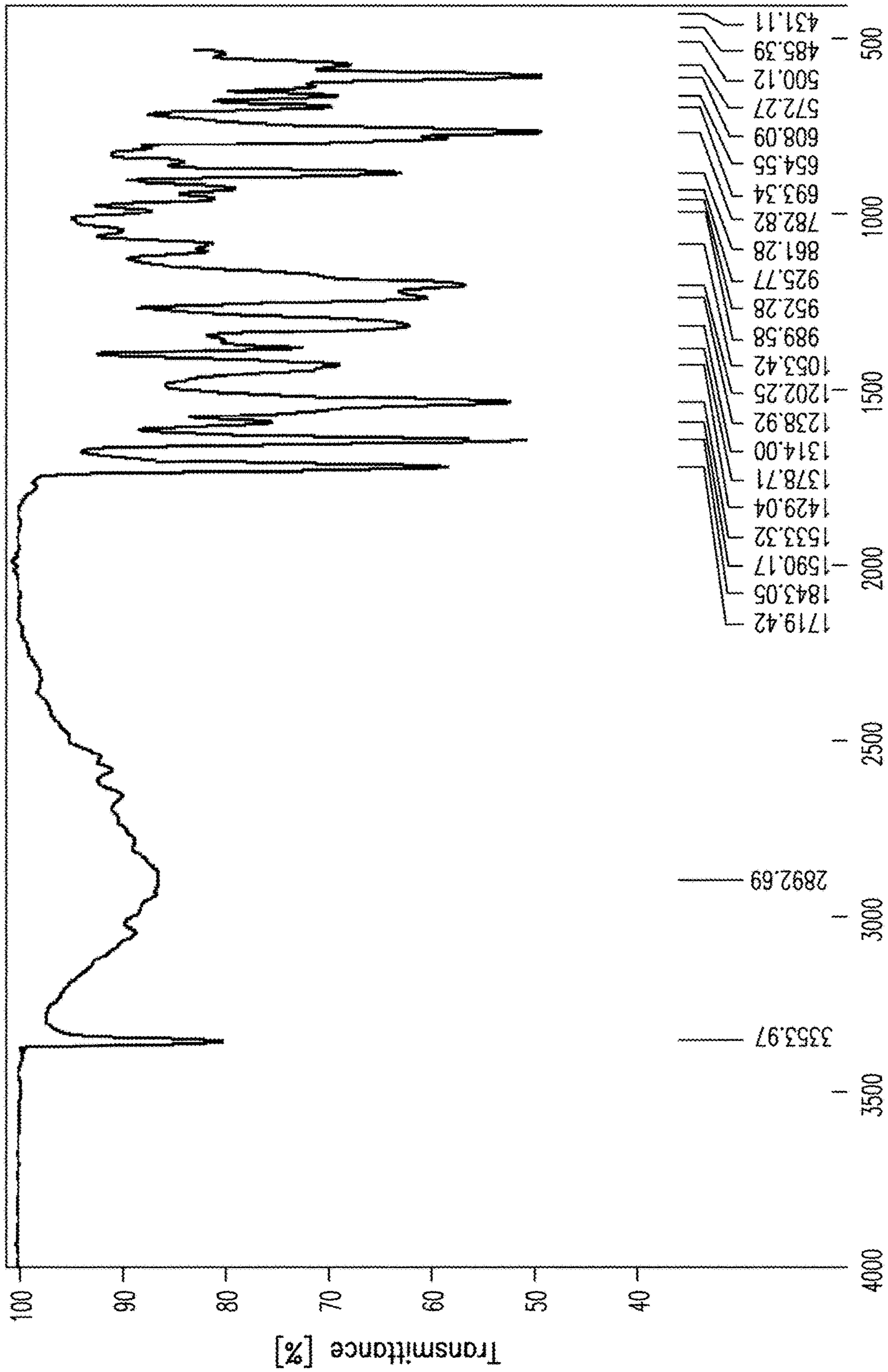
Wavenumber cm-1
