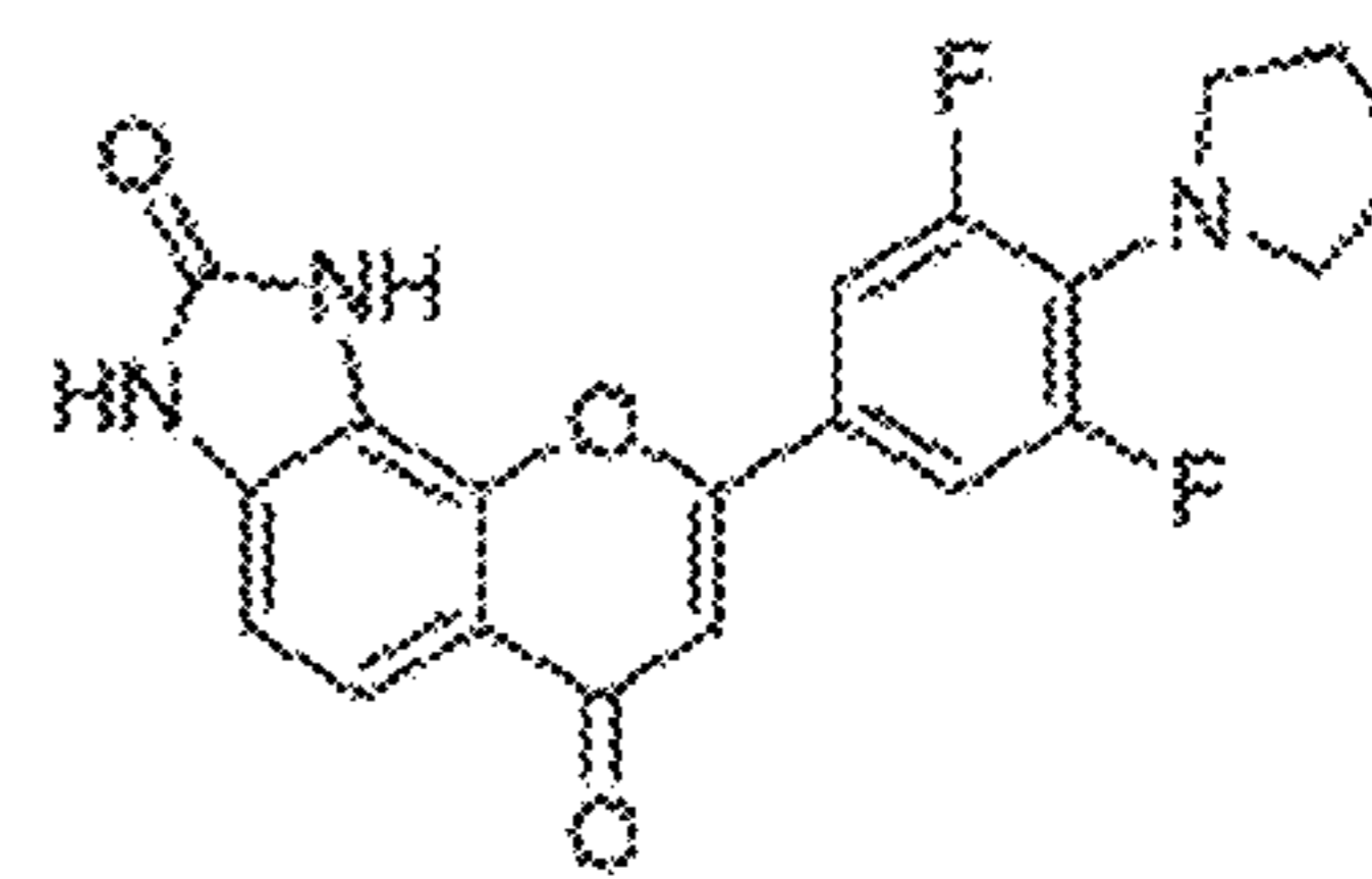
TCRS-202 MW = 383
