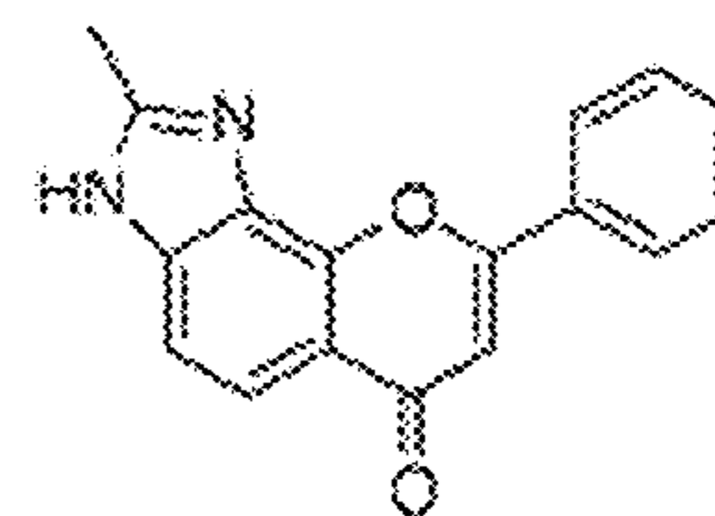
EU-D MW = 276
