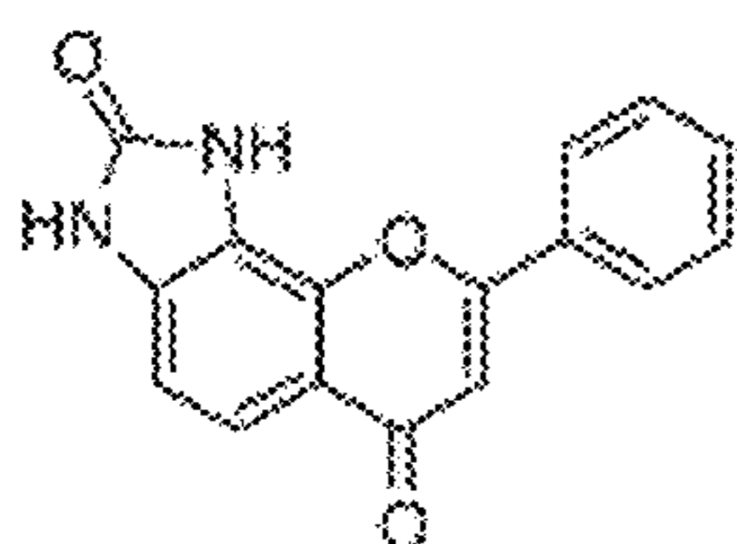
EU-E MW = 278
