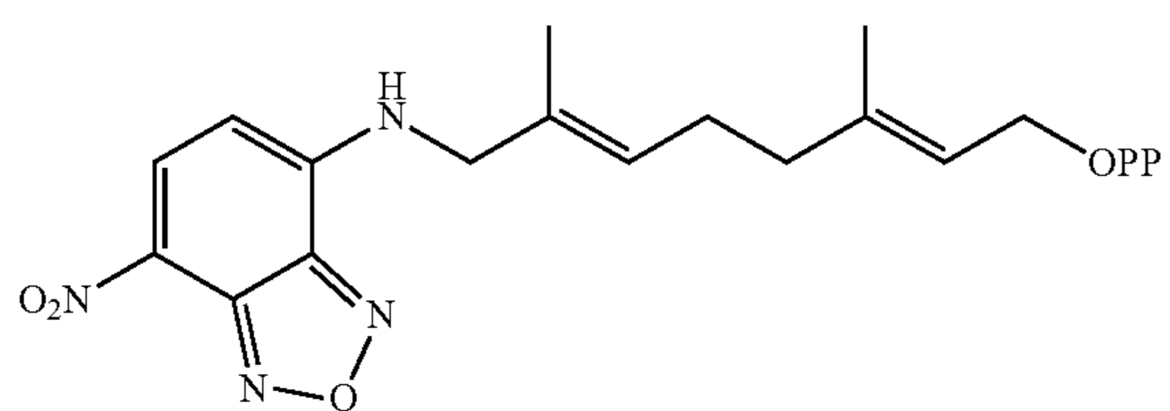
NBD-GPP
