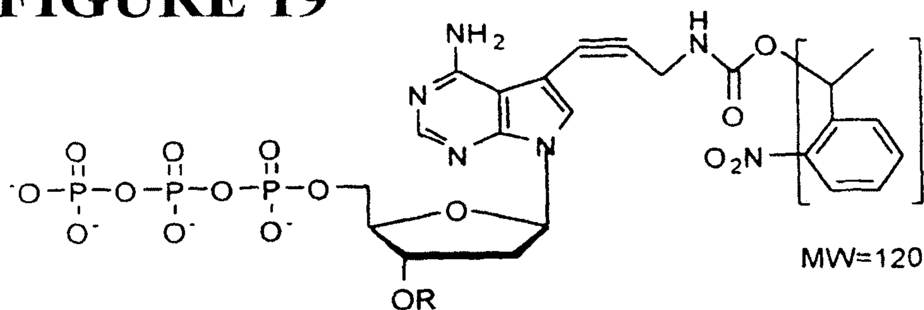
(Nitro-Benzyl)-dATP
