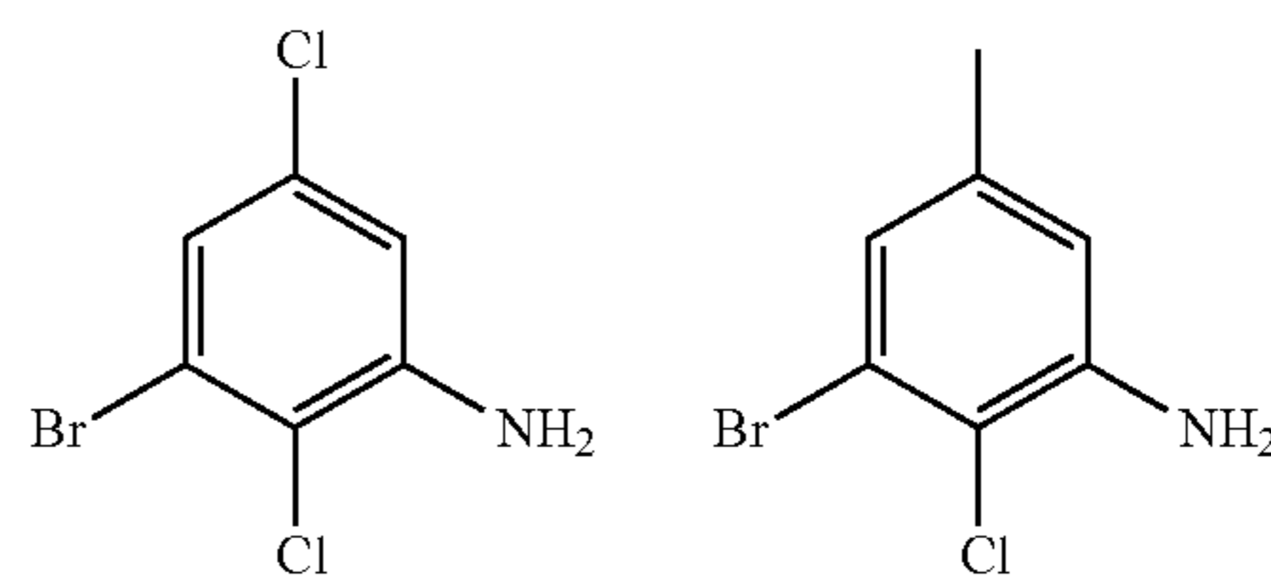
3-bromo-2,5-dichloroaniline
