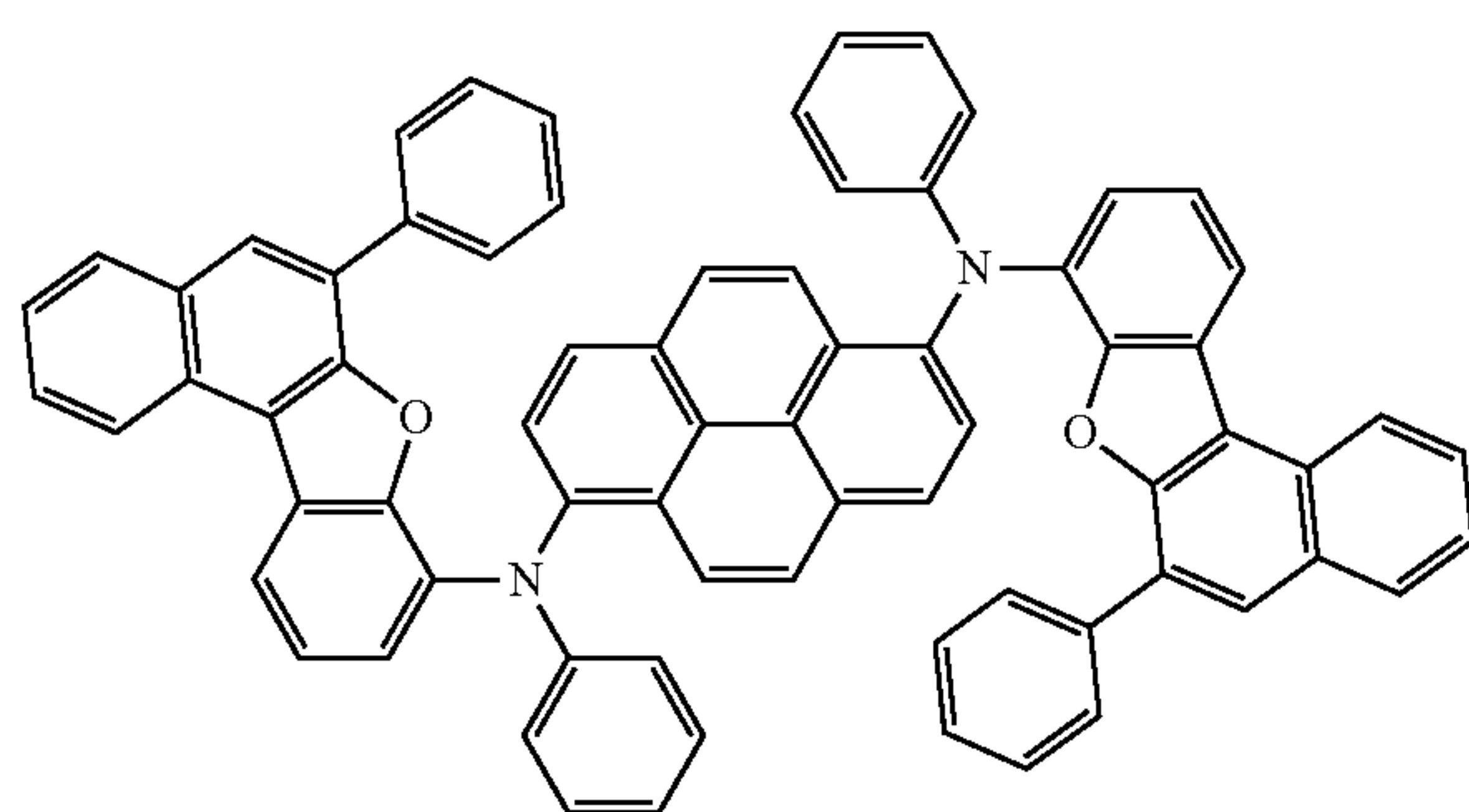
1,6BnfAPrn-03
