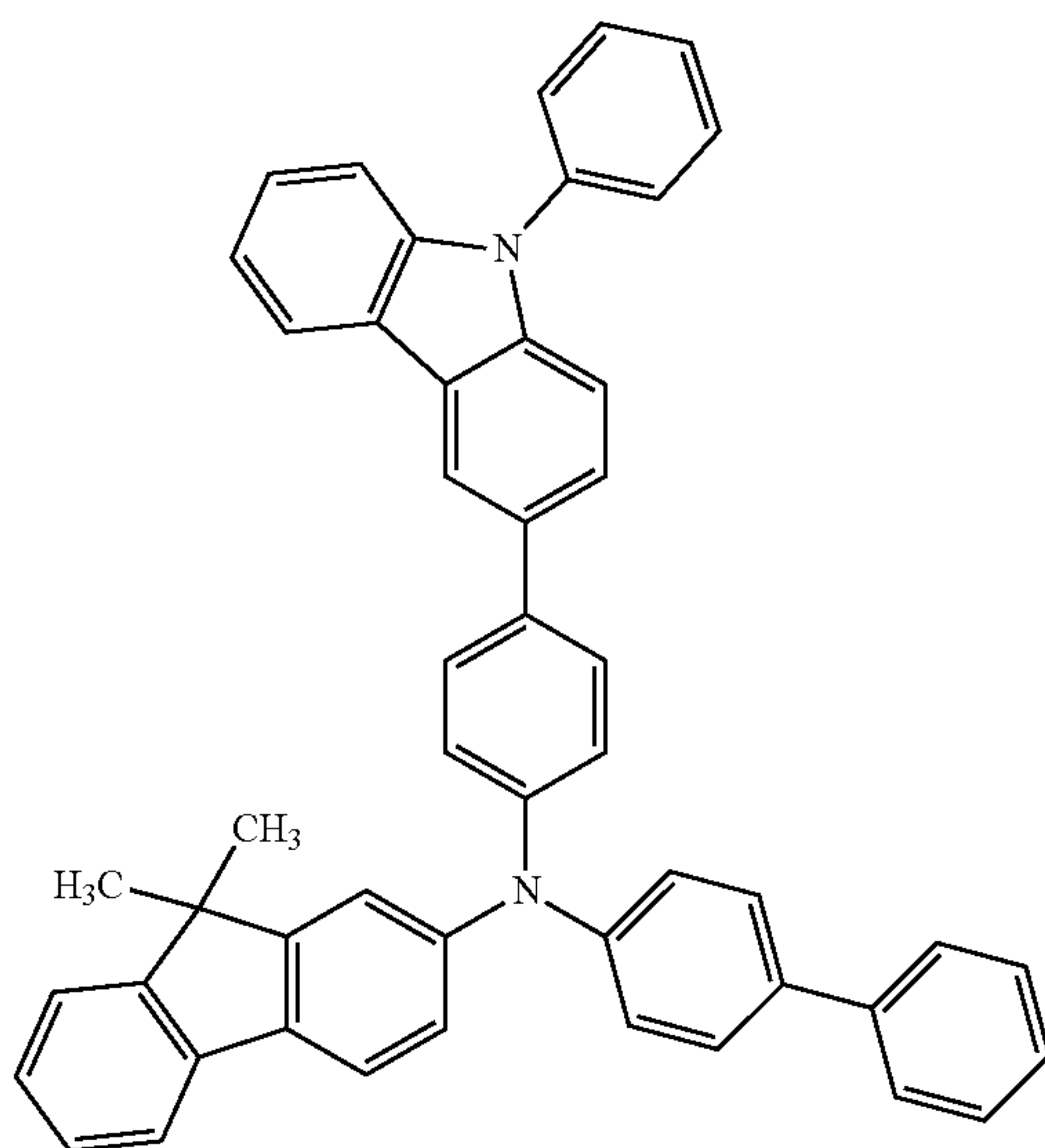
PCBBiF
