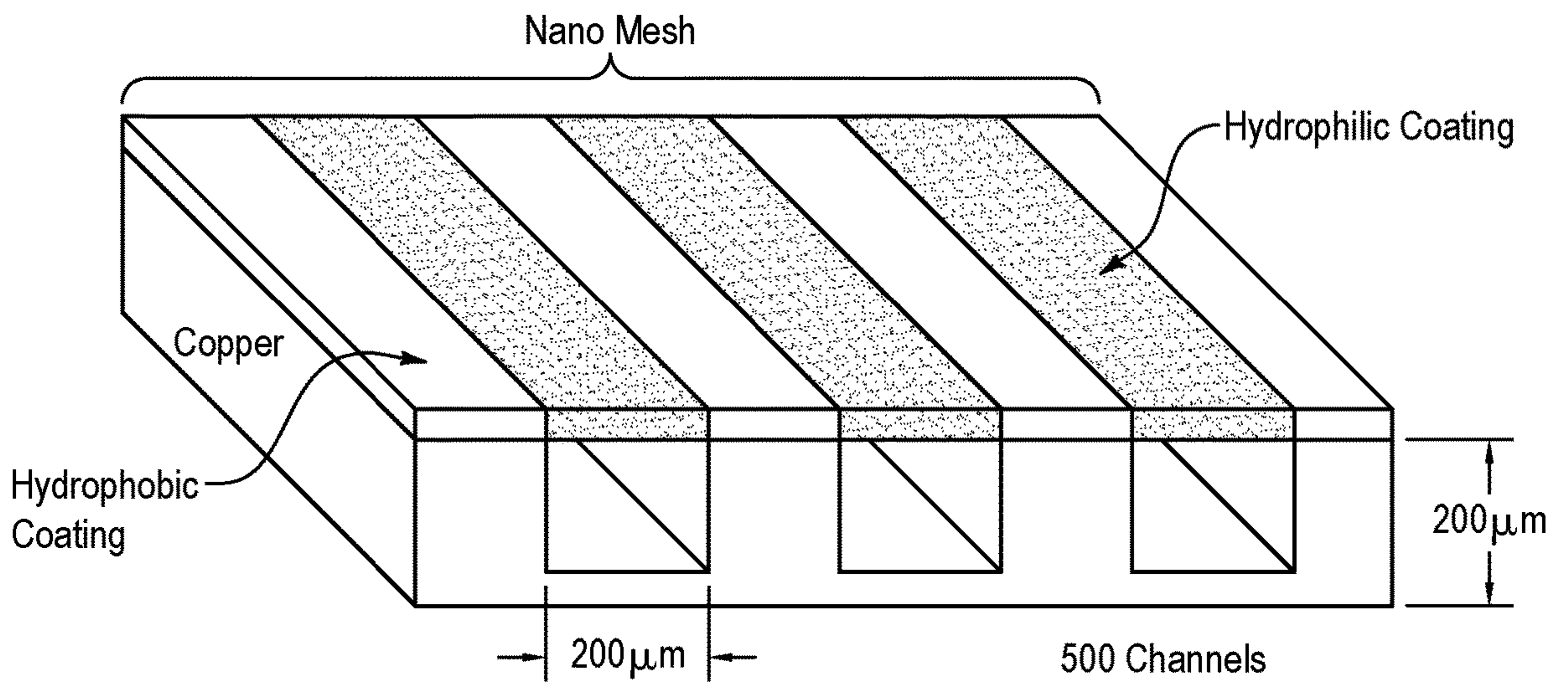
Condenser FIG. 20-b
