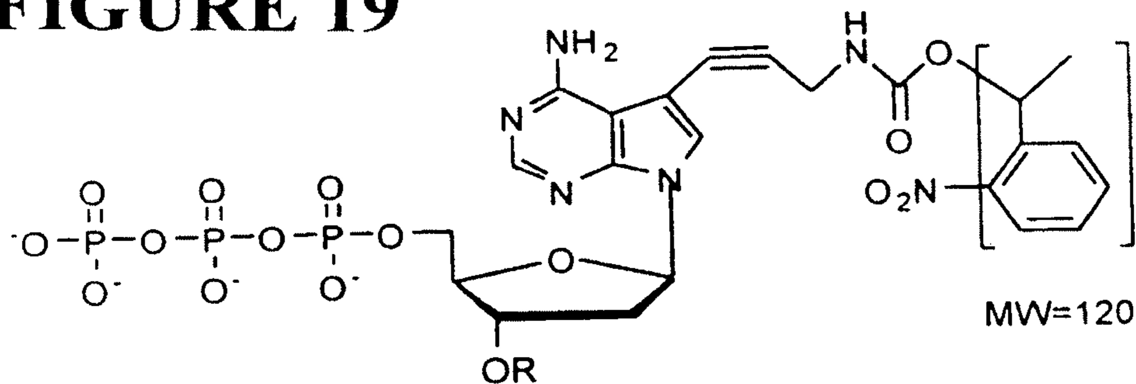
(Nitro-Benzyl)-dATP
