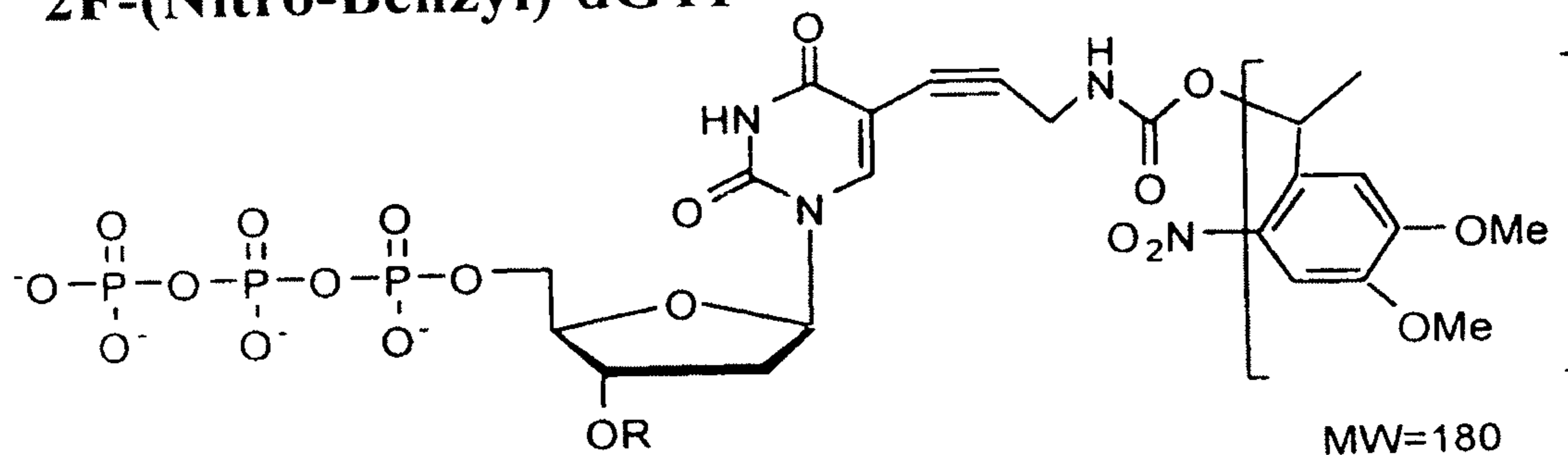
2(Meo)-(Nitro-Benzyl)-dTTP
