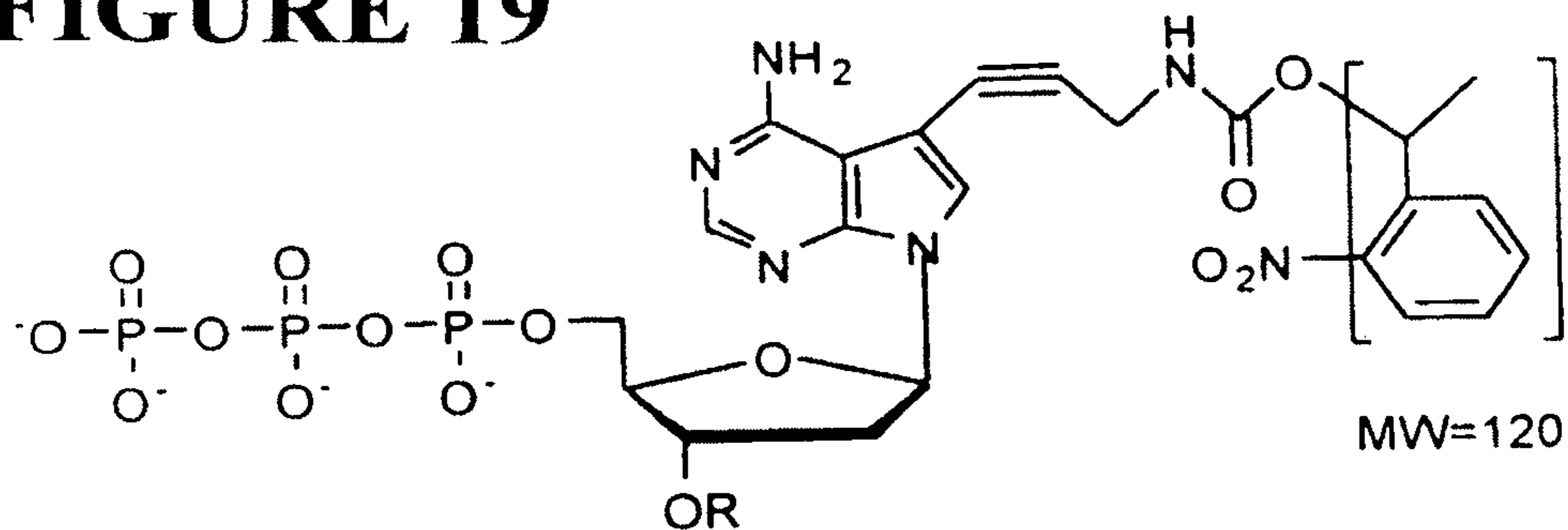
(Nitro-Benzyl)-dATP
