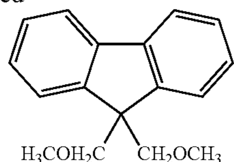
9,9-bis(methoxymethyl)fluorene
