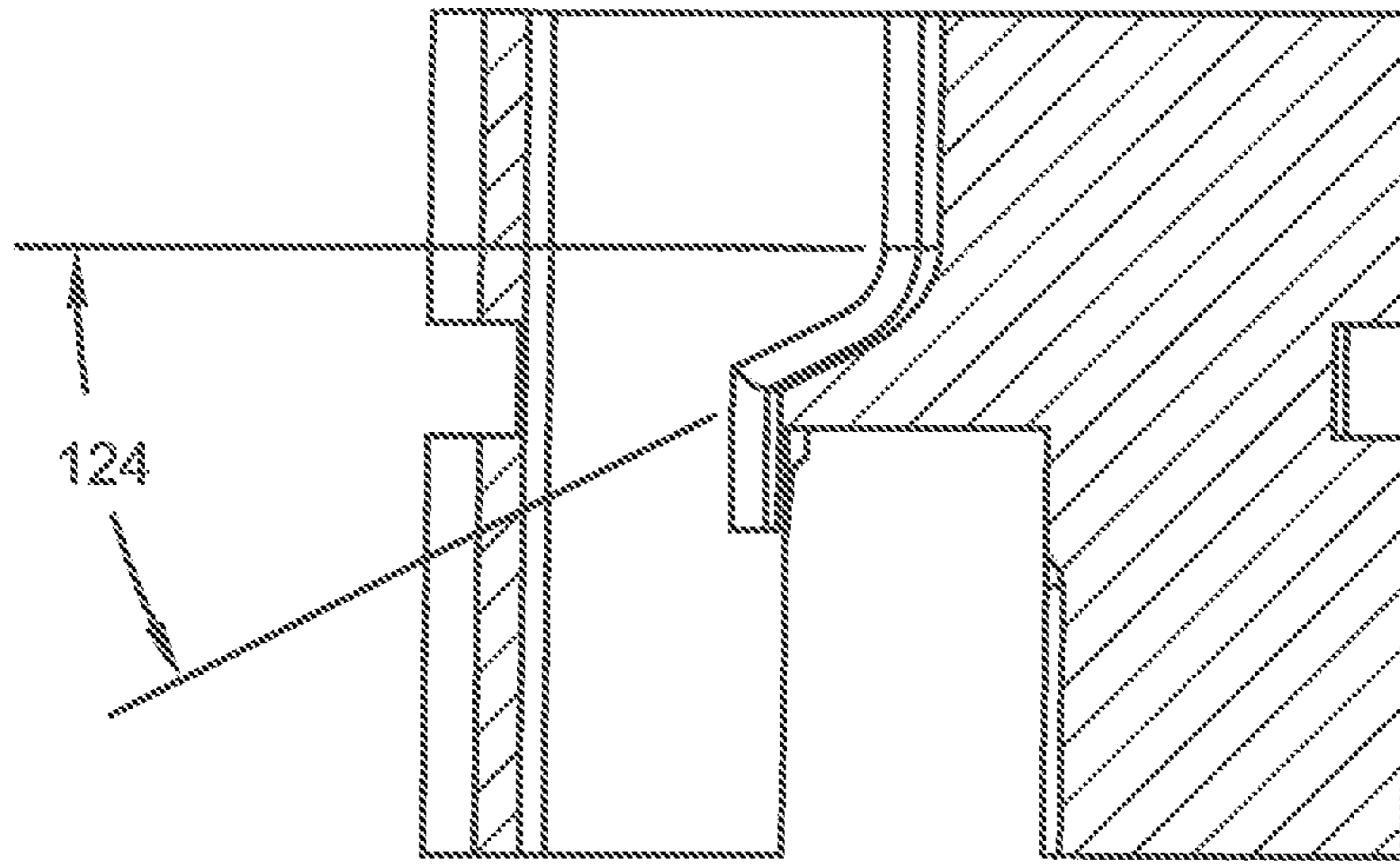
SECTION A-A
