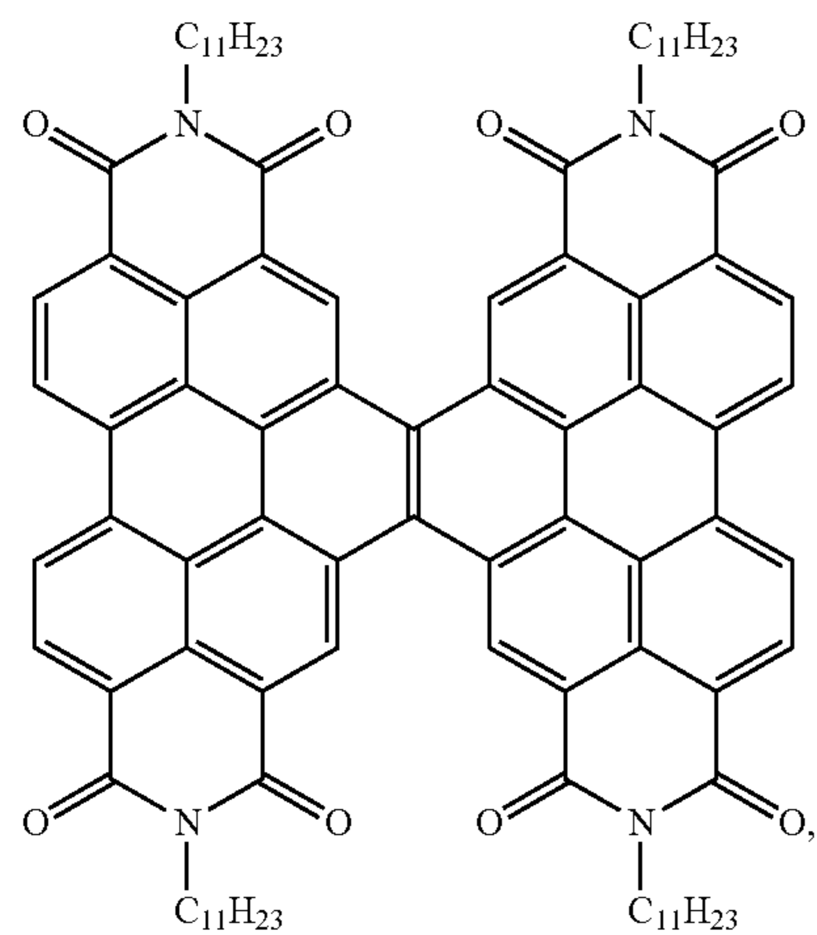
Dimer
