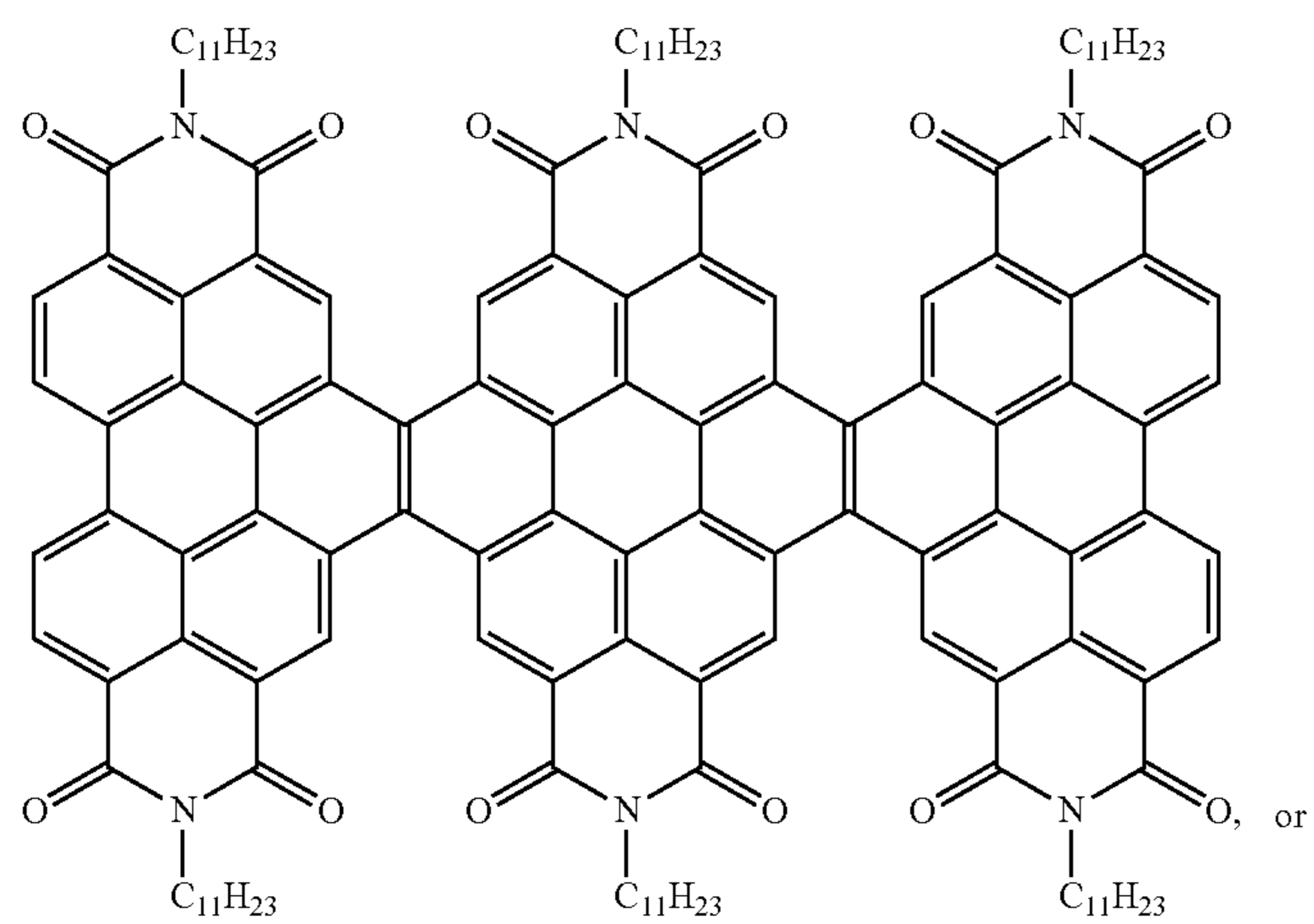
Trimer
