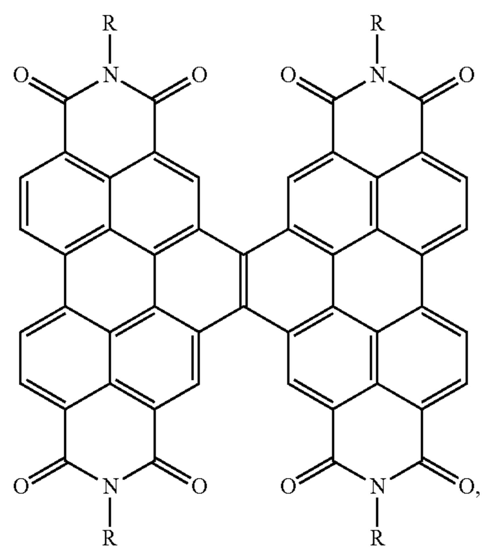
Dimer
