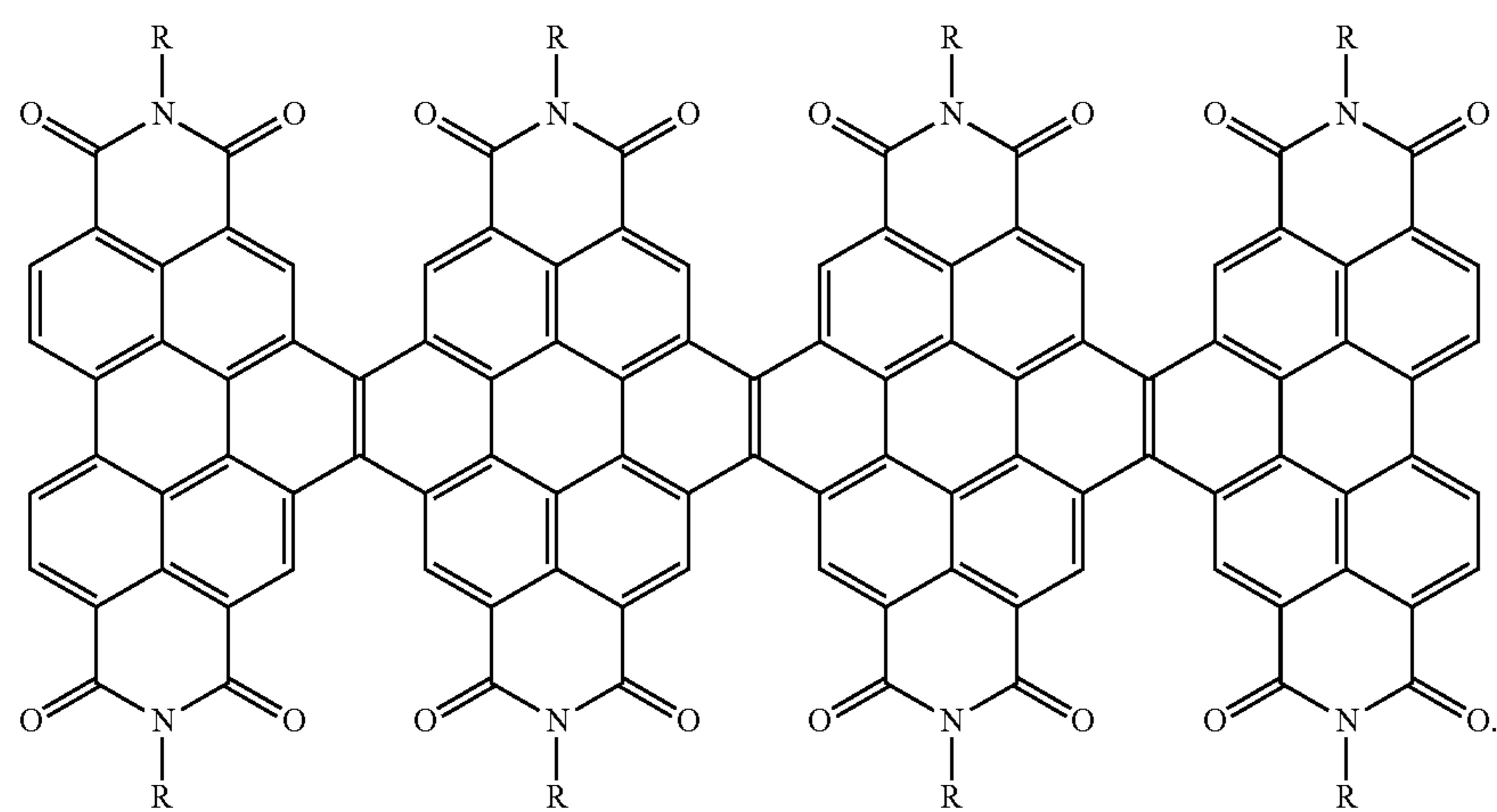
Tetramer
