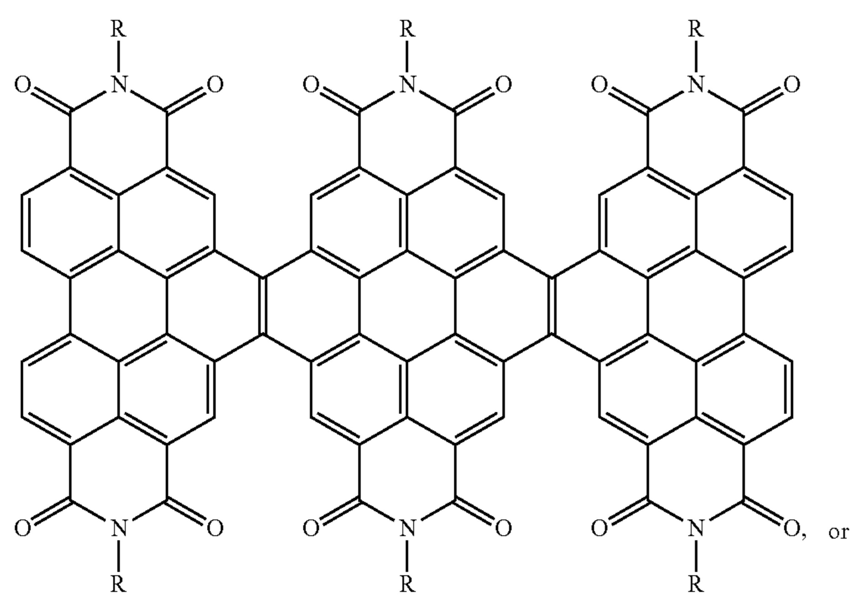
Trimer
