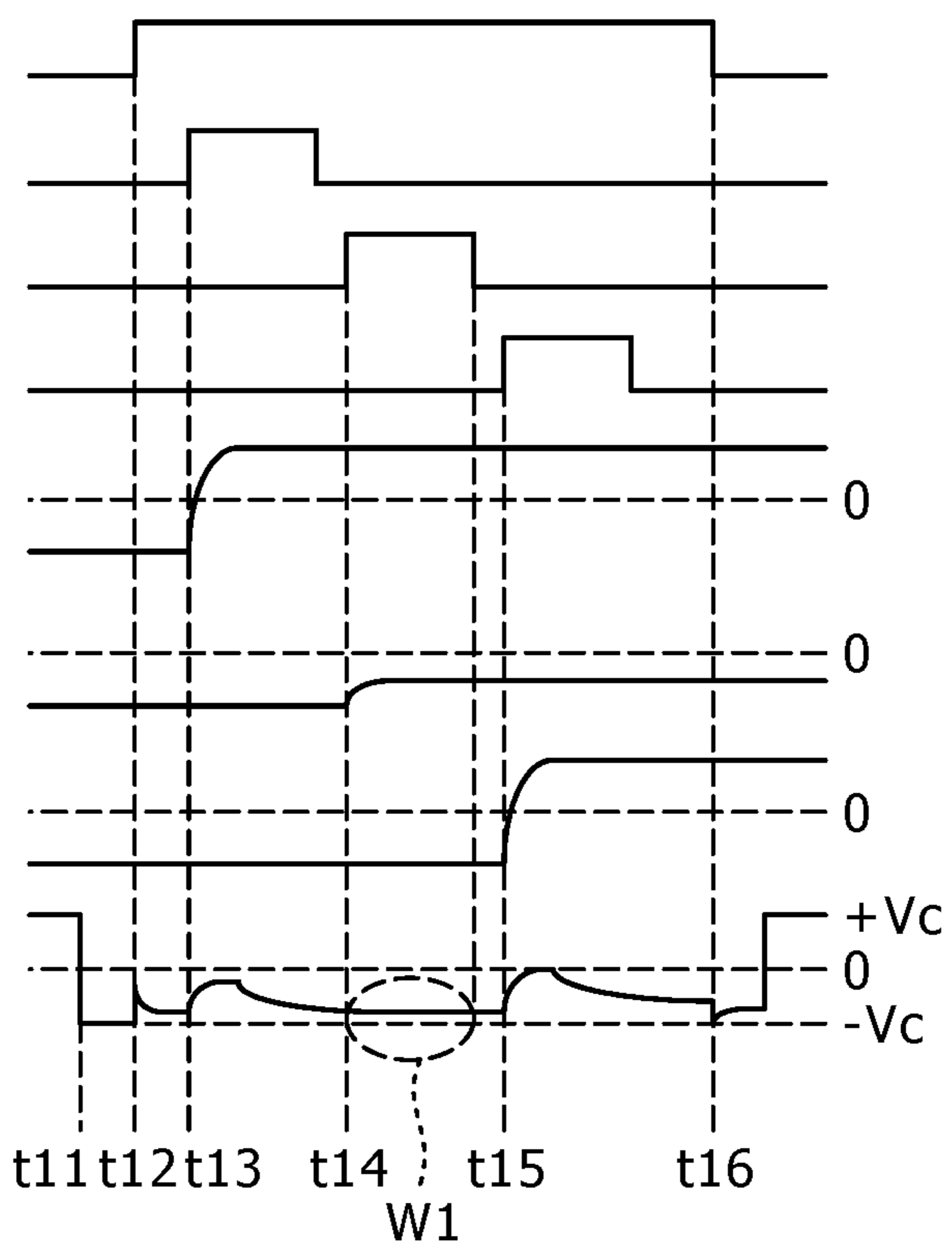
FIG. 12A V_{scan}(n)
