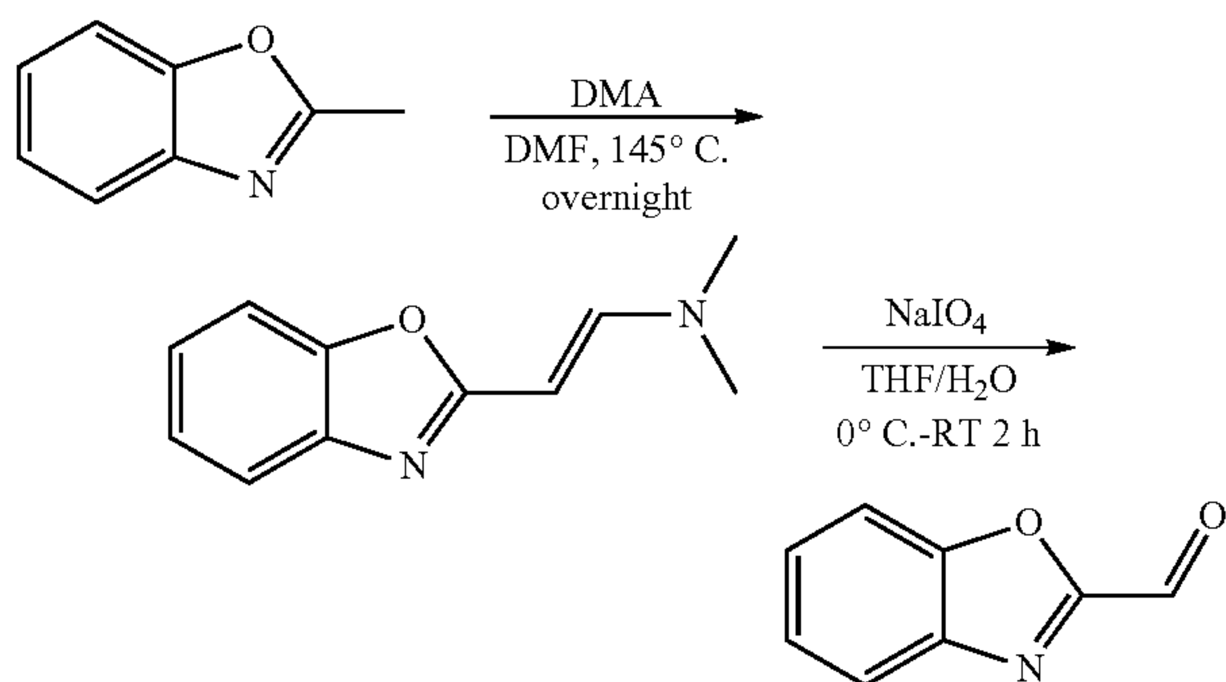
(a) (E)-2-(Benzo[d]oxazol-2-yl)-N,N-dimethylethanamine
