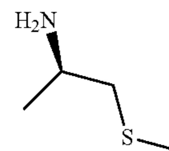
A. (R)-1-(Methylthio)propan-2-amine
