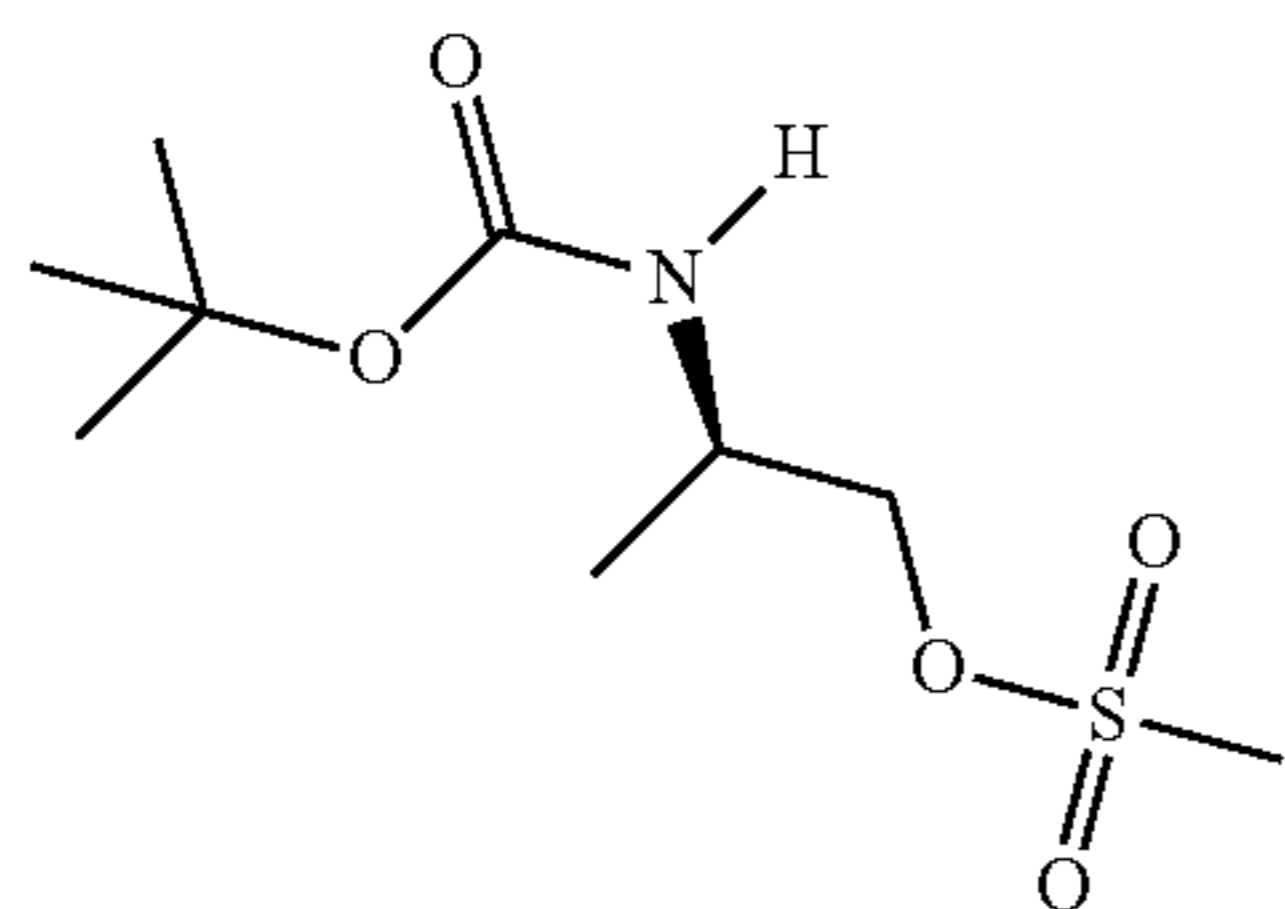
A. (R)-2-((tert-Butoxycarbonyl)amino)propyl methanesulfonate
