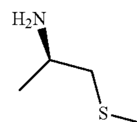
C. (R)-1-(Methylthio)propan-2-amine hydrochloride
