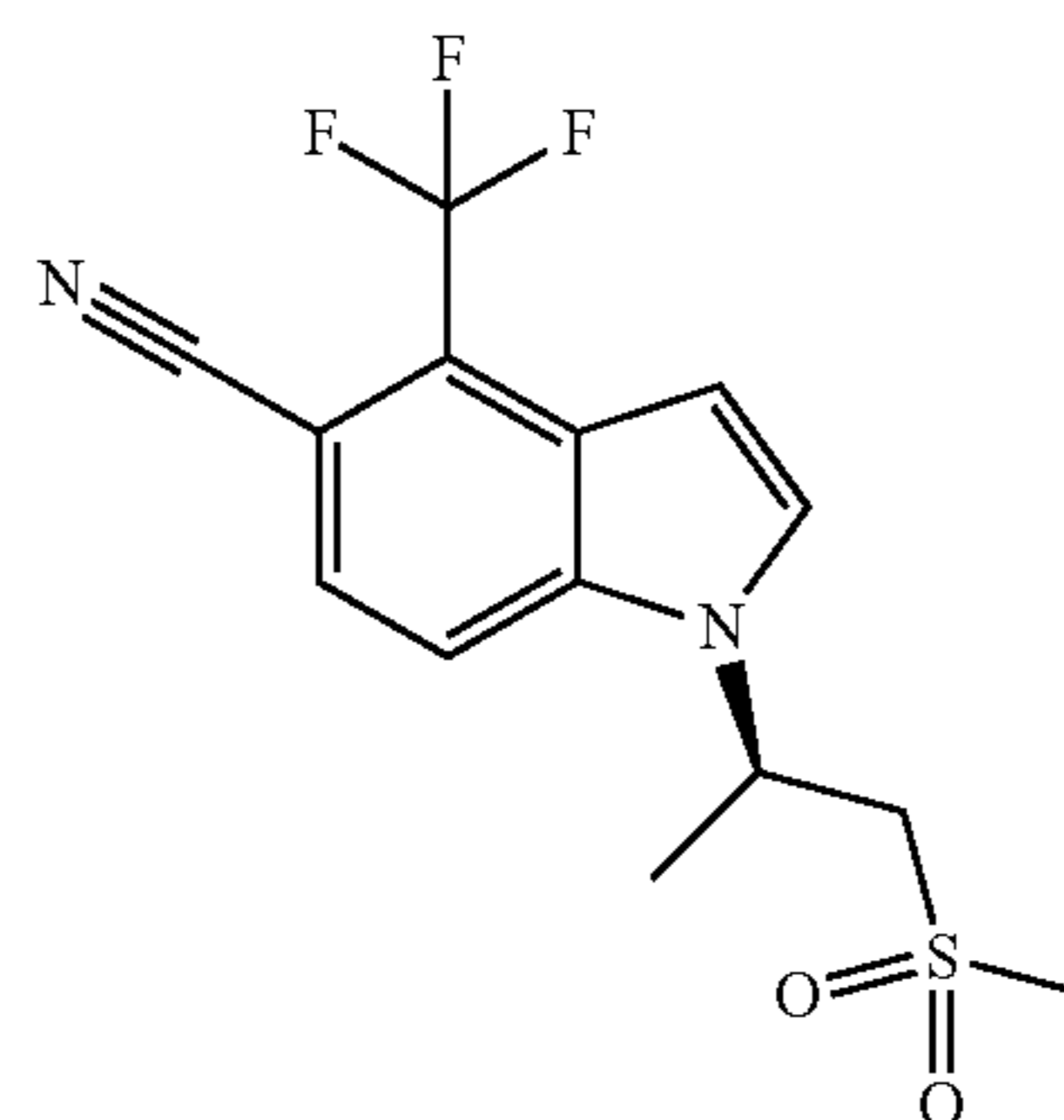
(R)-1-(1-(methylsulfonyl)propan-2-yl)-4-(trifluoromethyl)-1H-indole-5-carbonitrile
