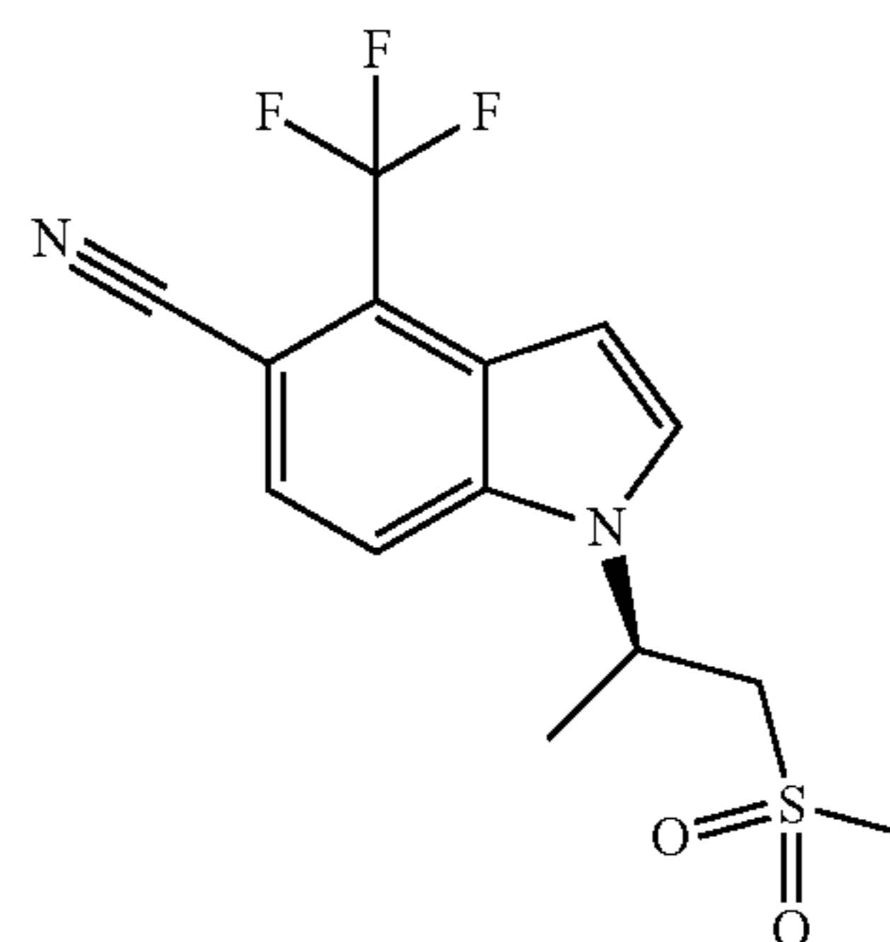
(R)-1-(1-(methylsulfonyl)propan-2-yl)-4-(trifluoromethyl)-1H-indole-5-carbonitrile
