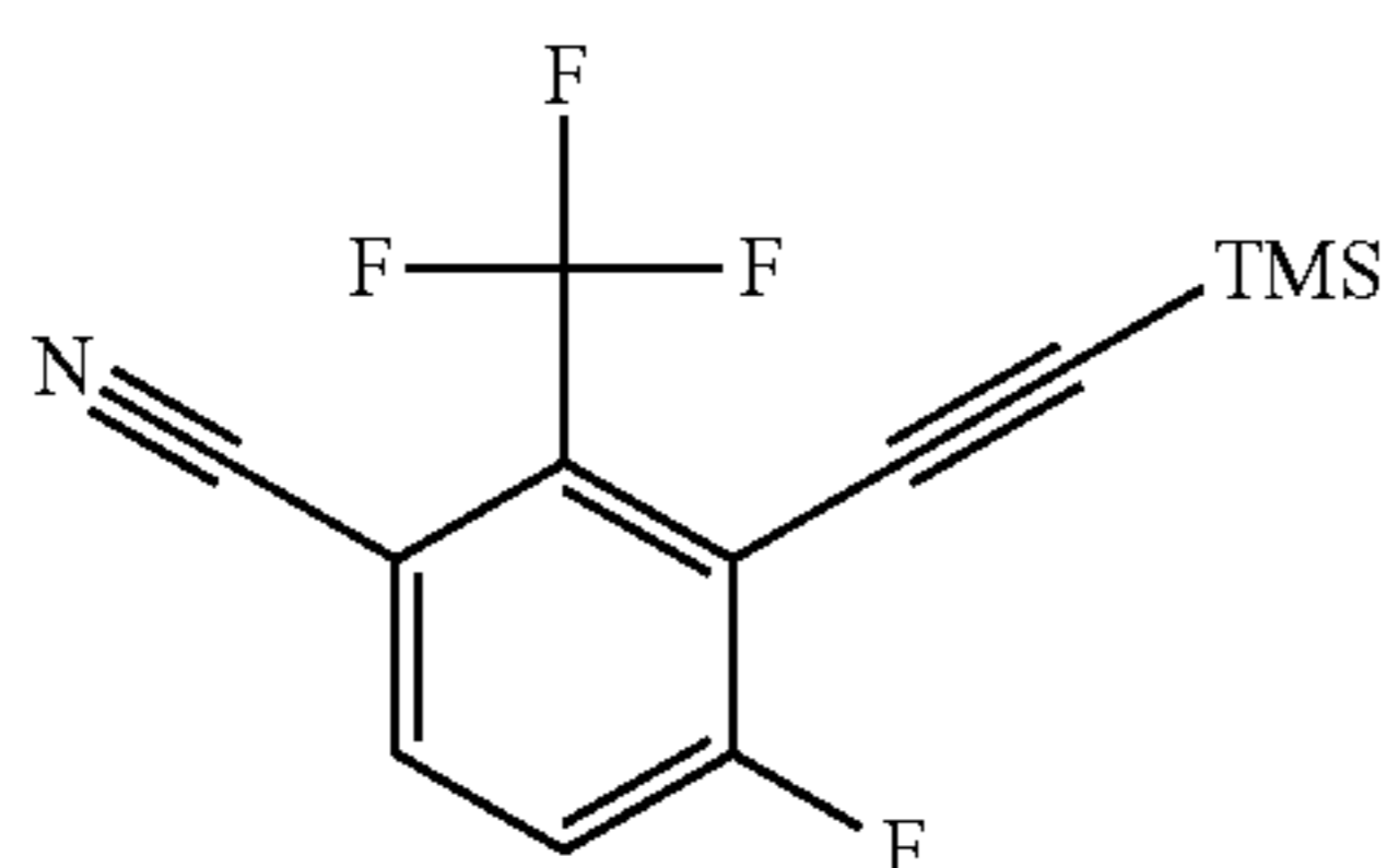
E. 4-Fluoro-2-(trifluoromethyl)-3-((trimethylsilyl)ethynyl)benzonitrile
