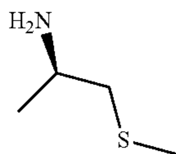
(R)-1-(methylthio)propan-2-amine hydrochloride
