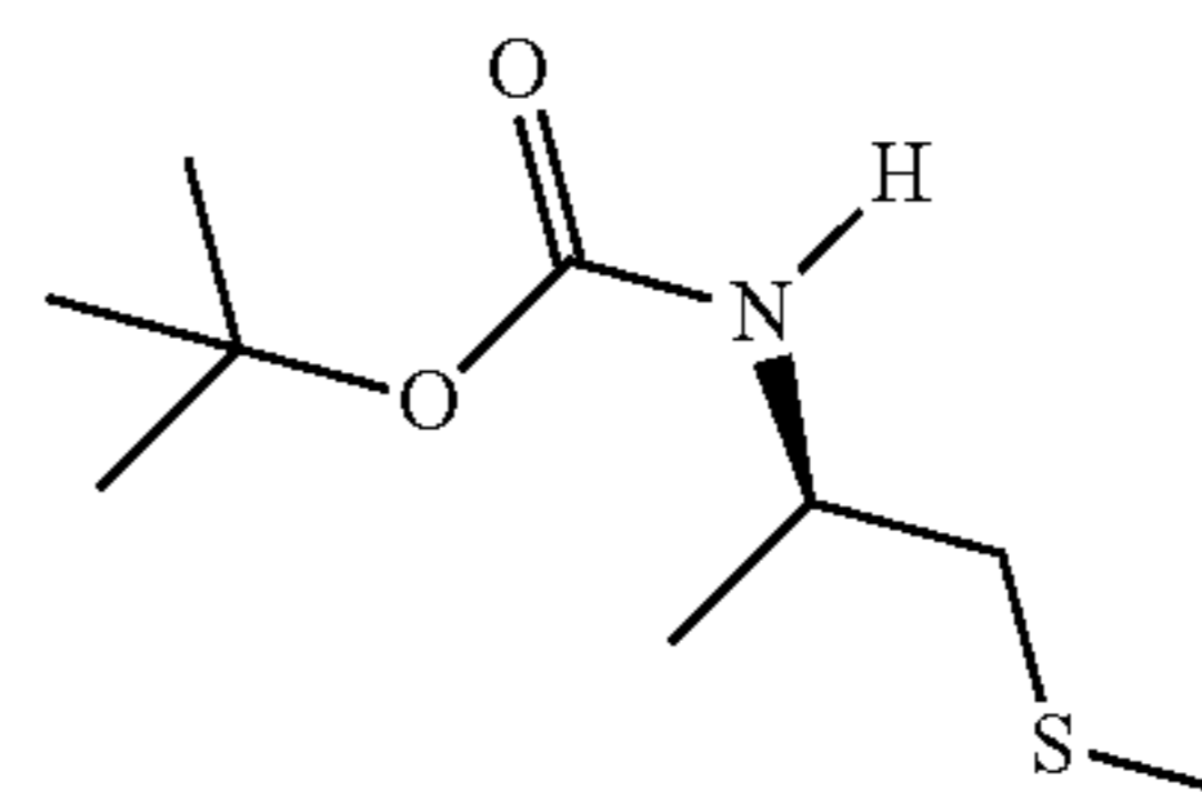
B. (R)-tert-Butyl (1-(methylthio)propan-2-yl)carbamate
