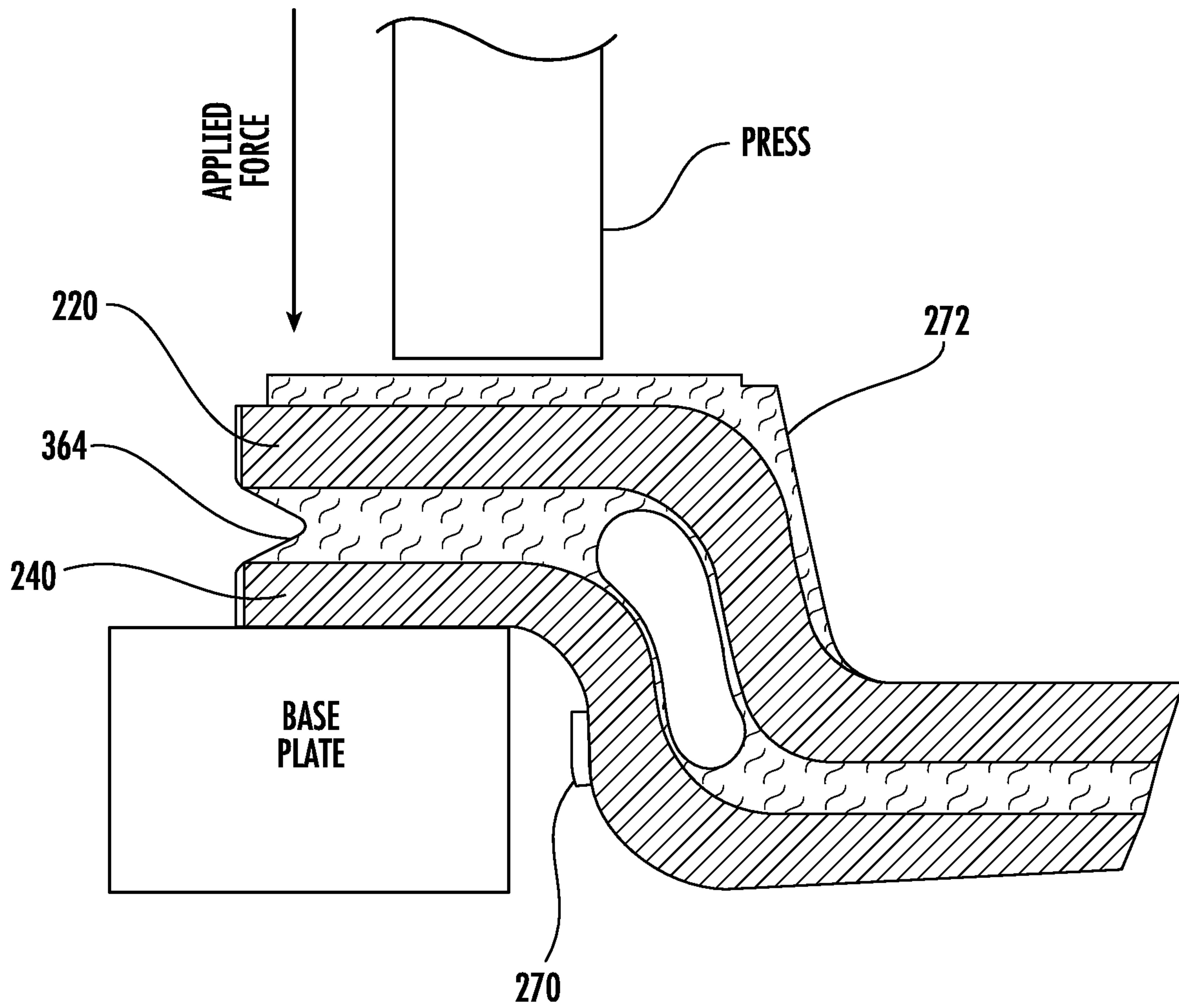
FIG. 24
