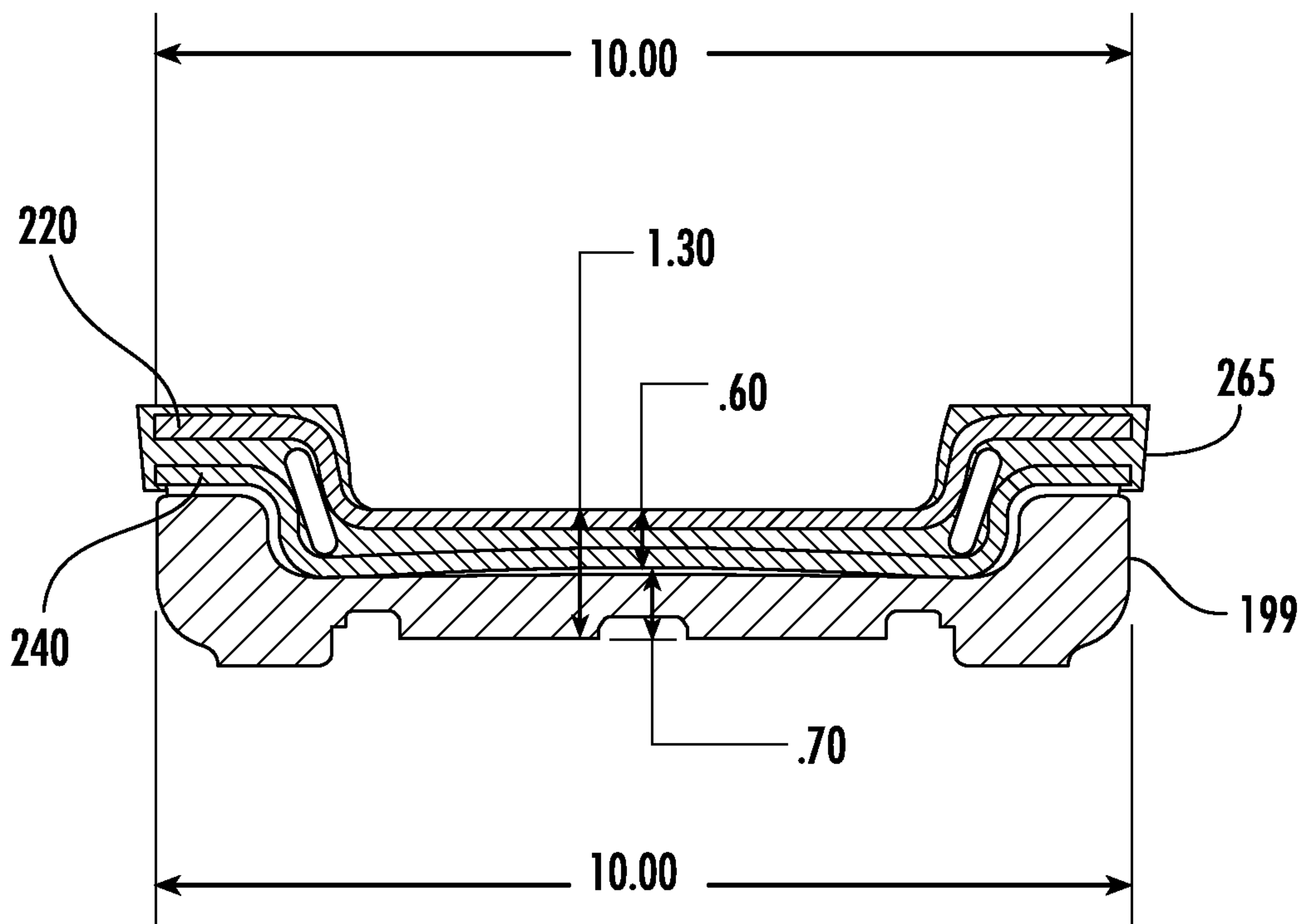
FIG. 13C
