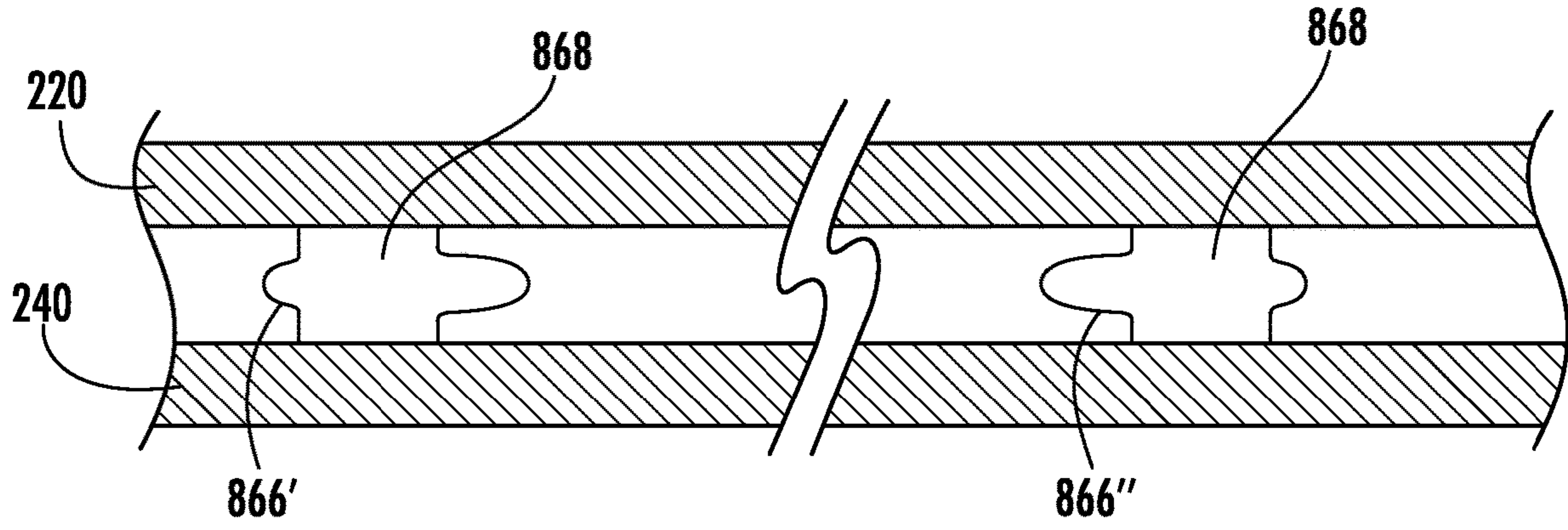
FIG. 20A
