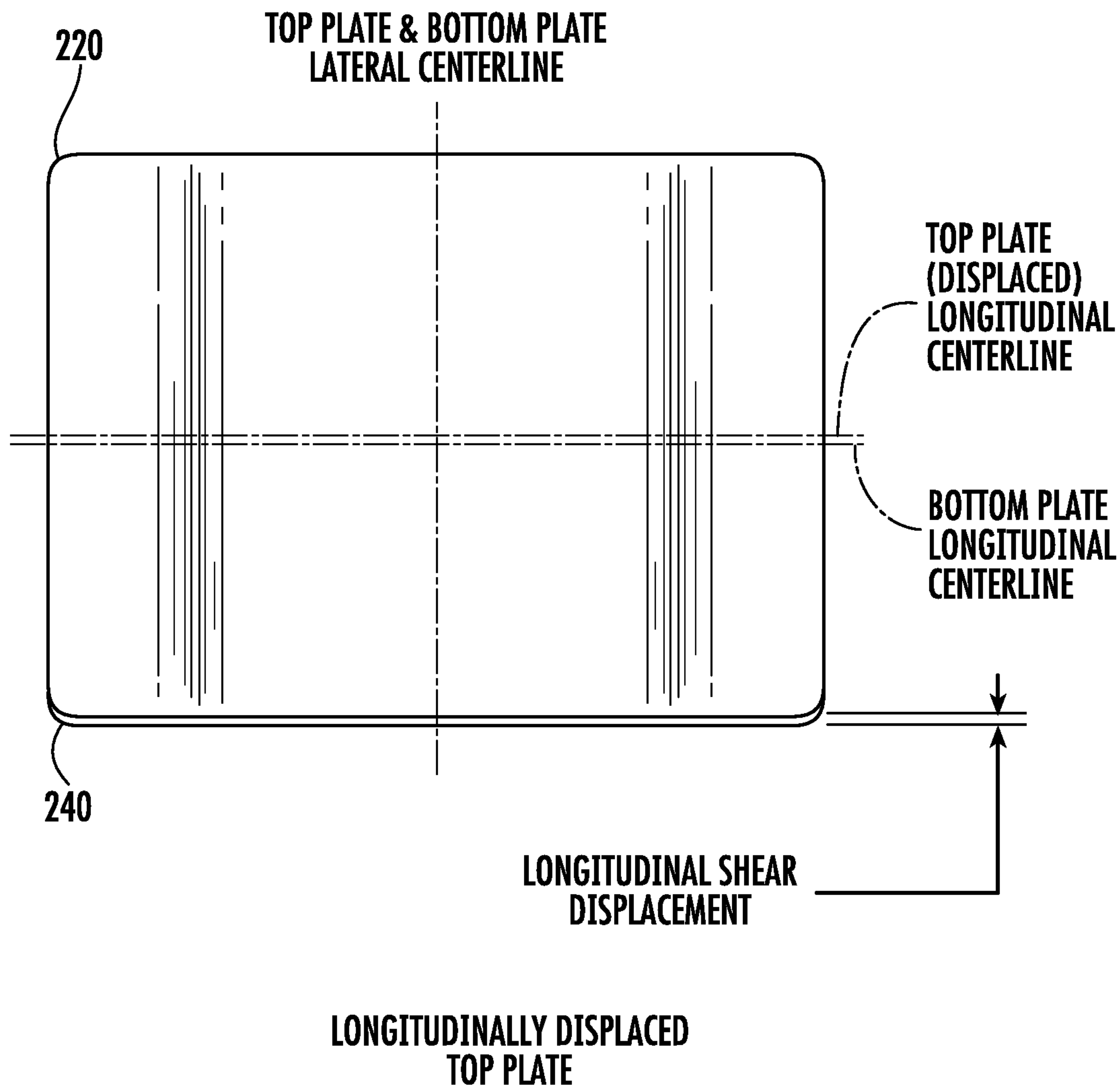
FIG. 17B
