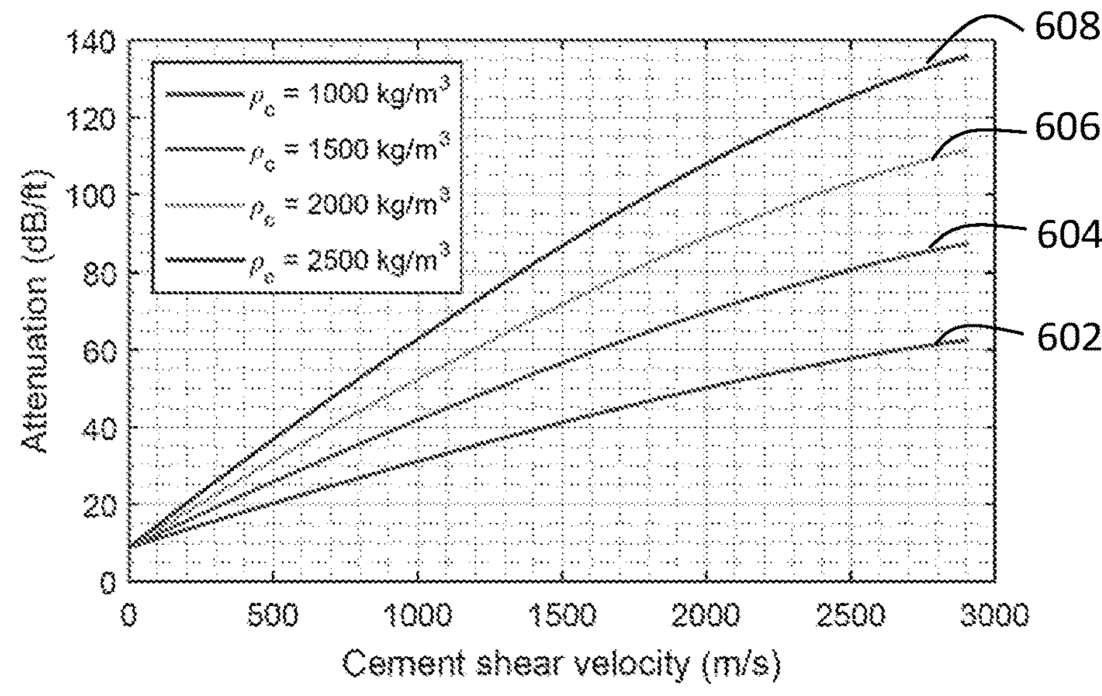
FIG. 6C
