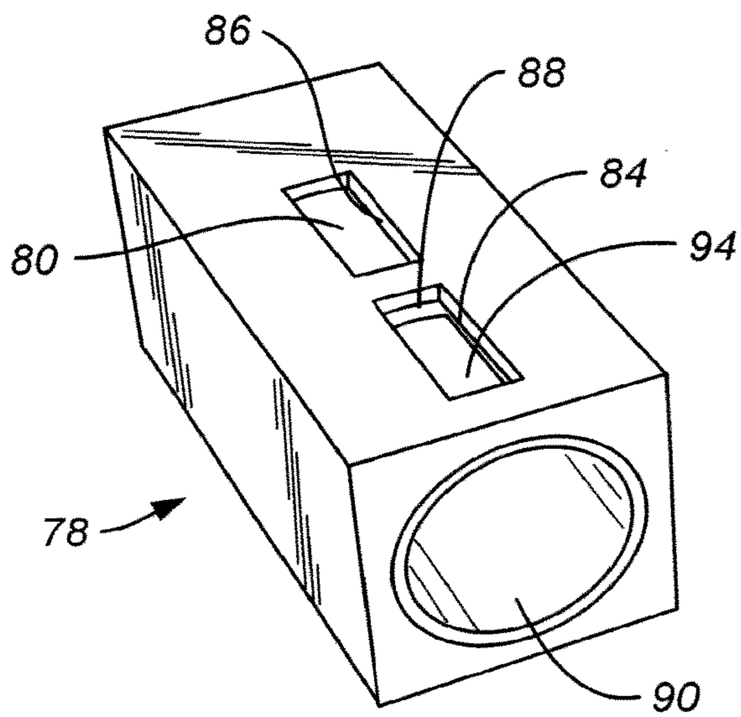
FIG. 14
