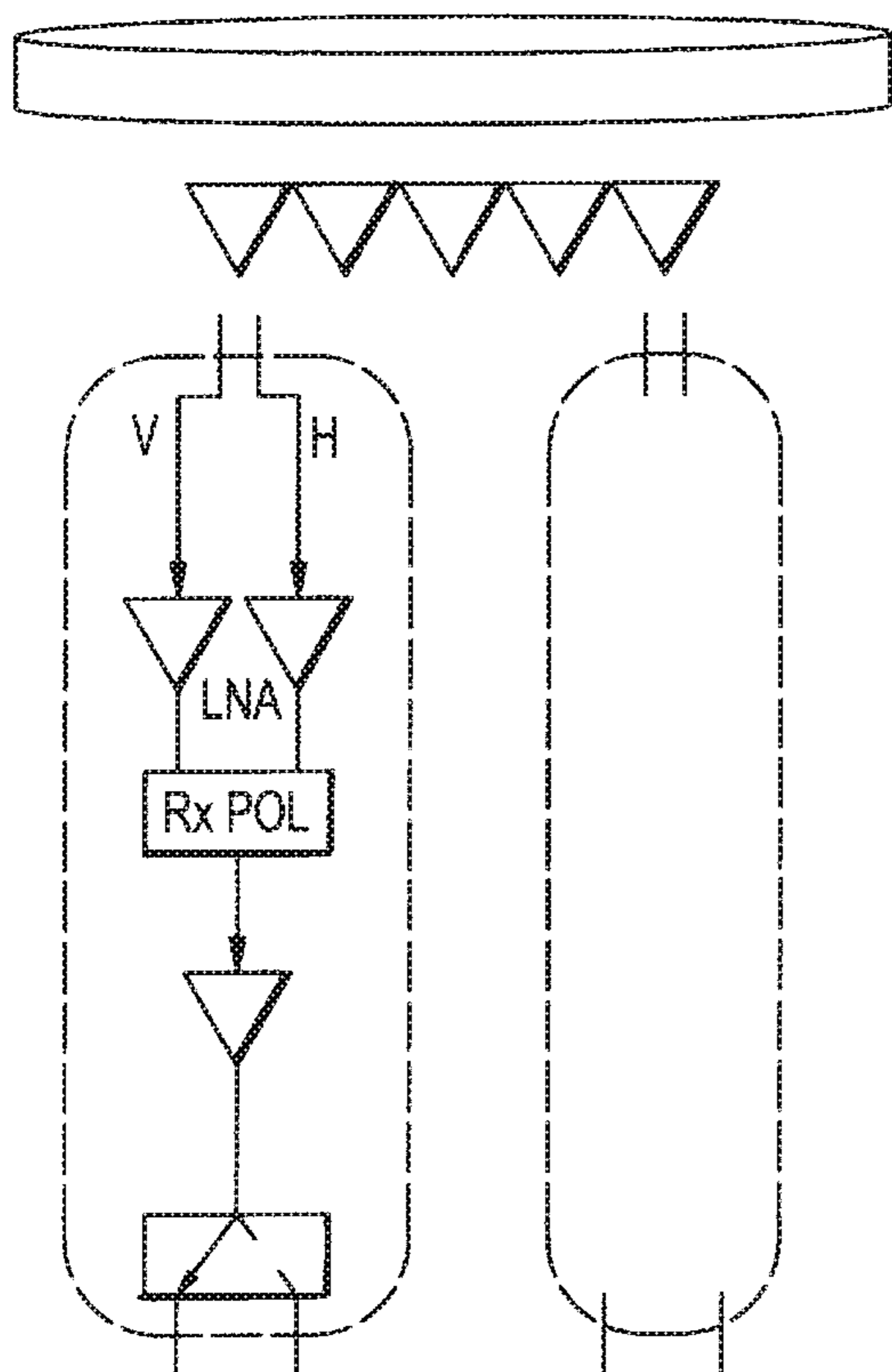
FIG. 9a
