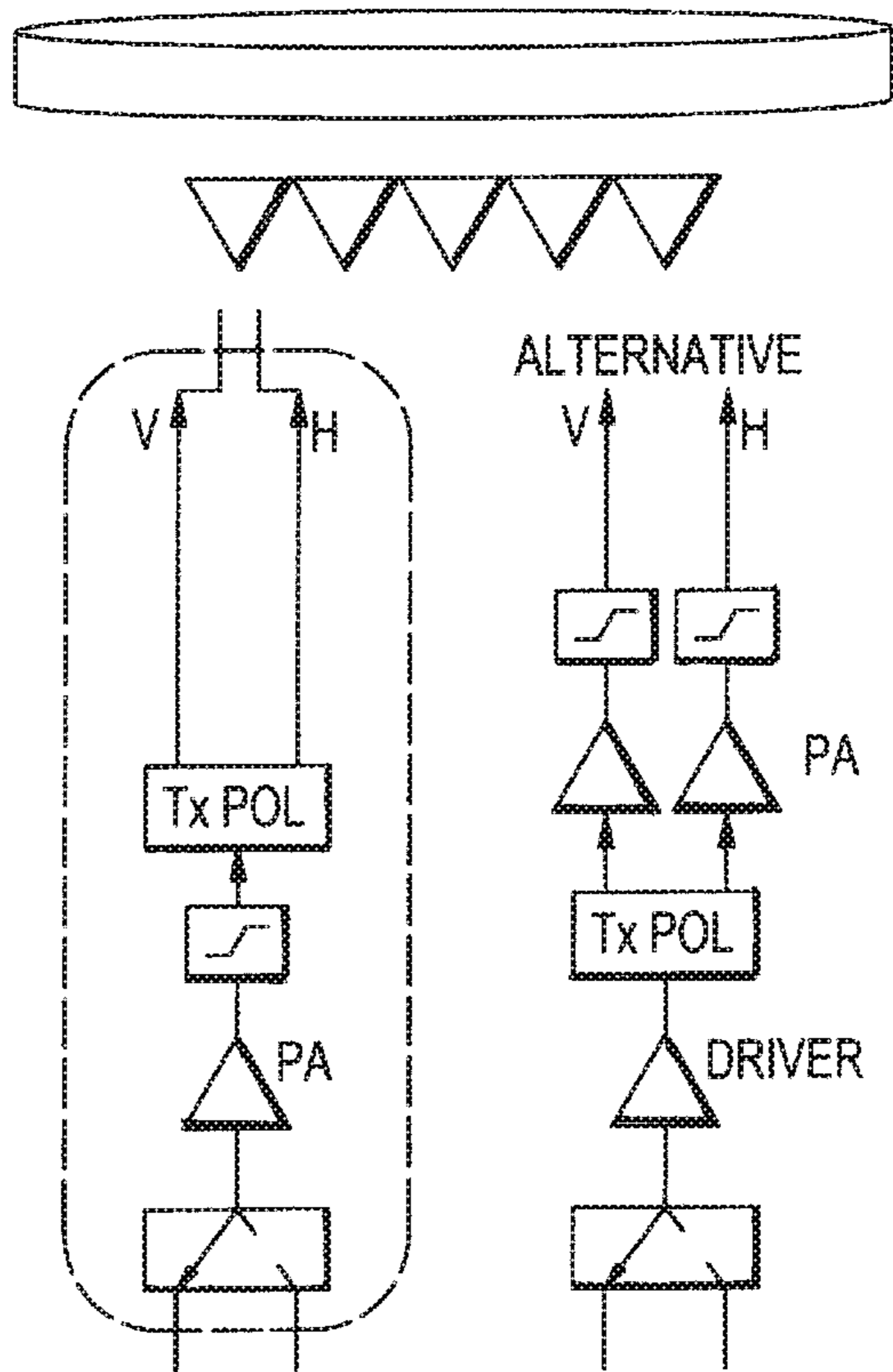
FIG. 9b
