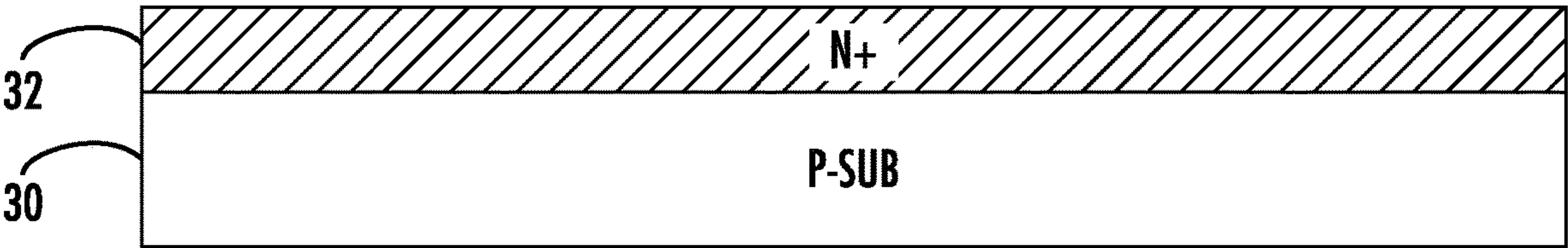
FIG. 3A (A~A')
