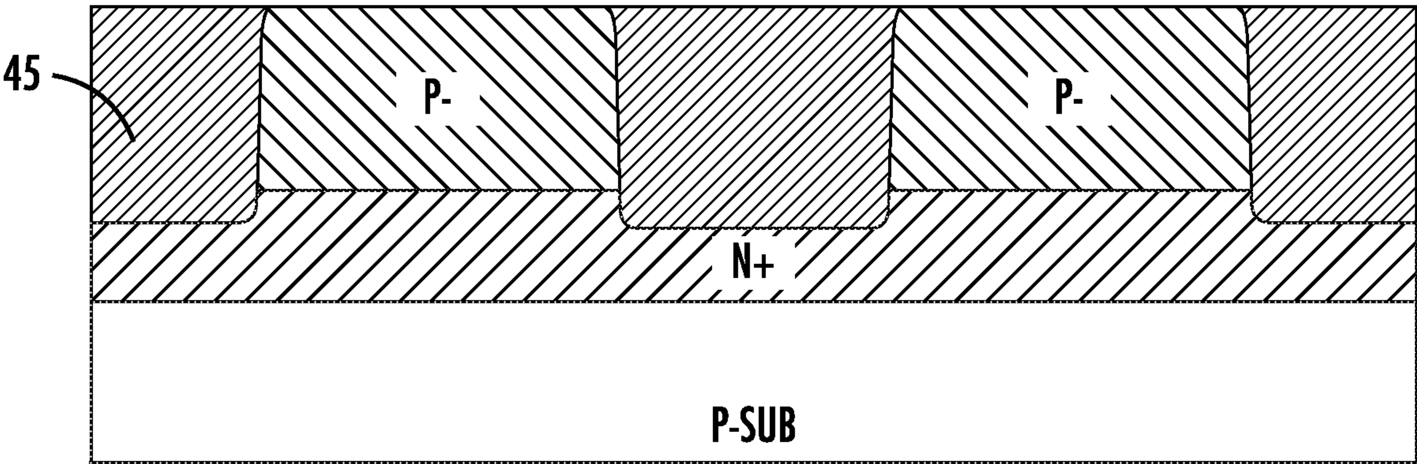
FIG. 7B (B~B')
