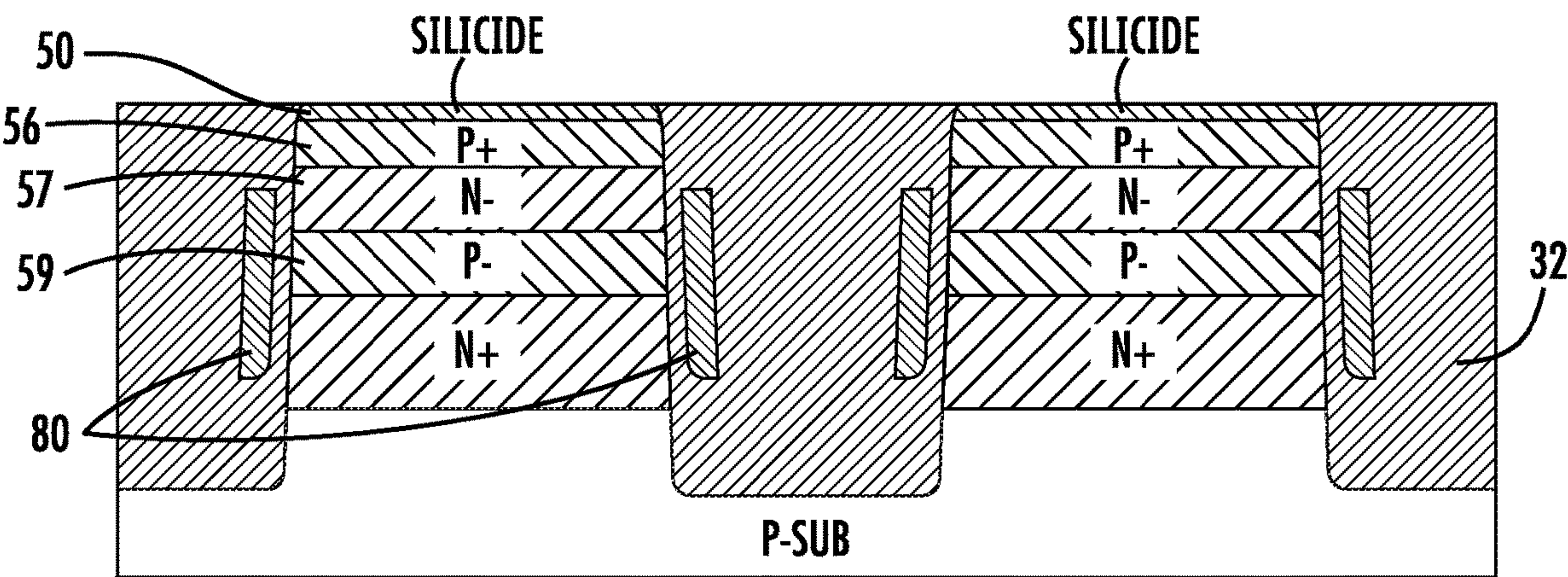
FIG. 15A (A~A')
