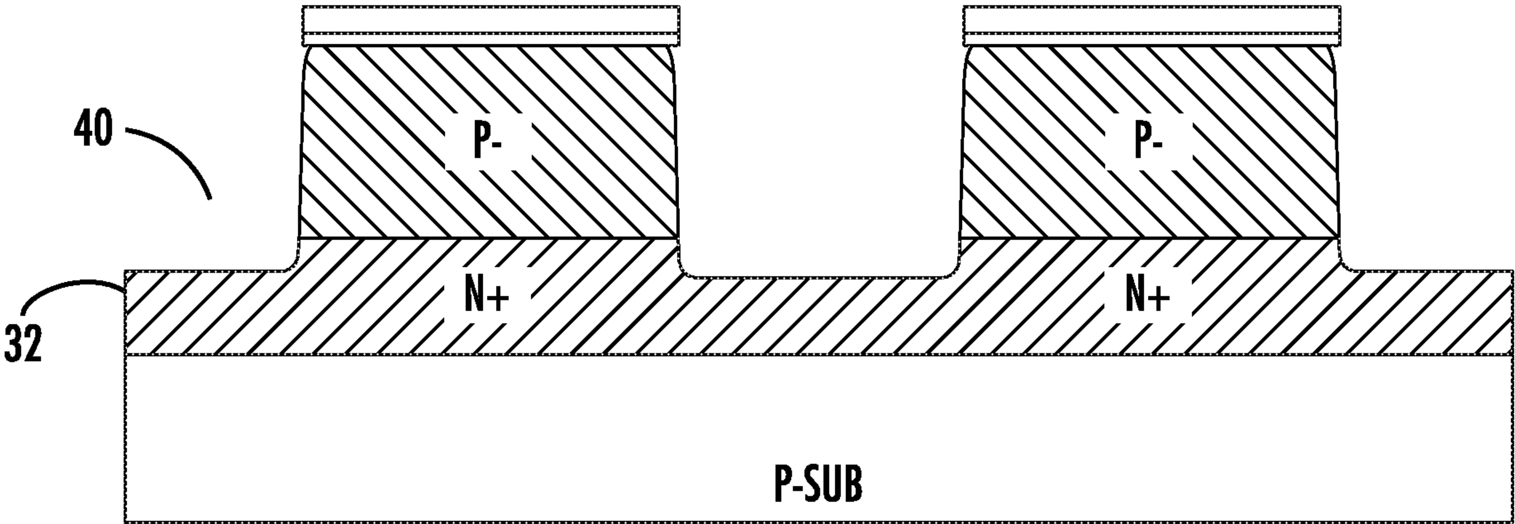
FIG. 6B (B~B')
