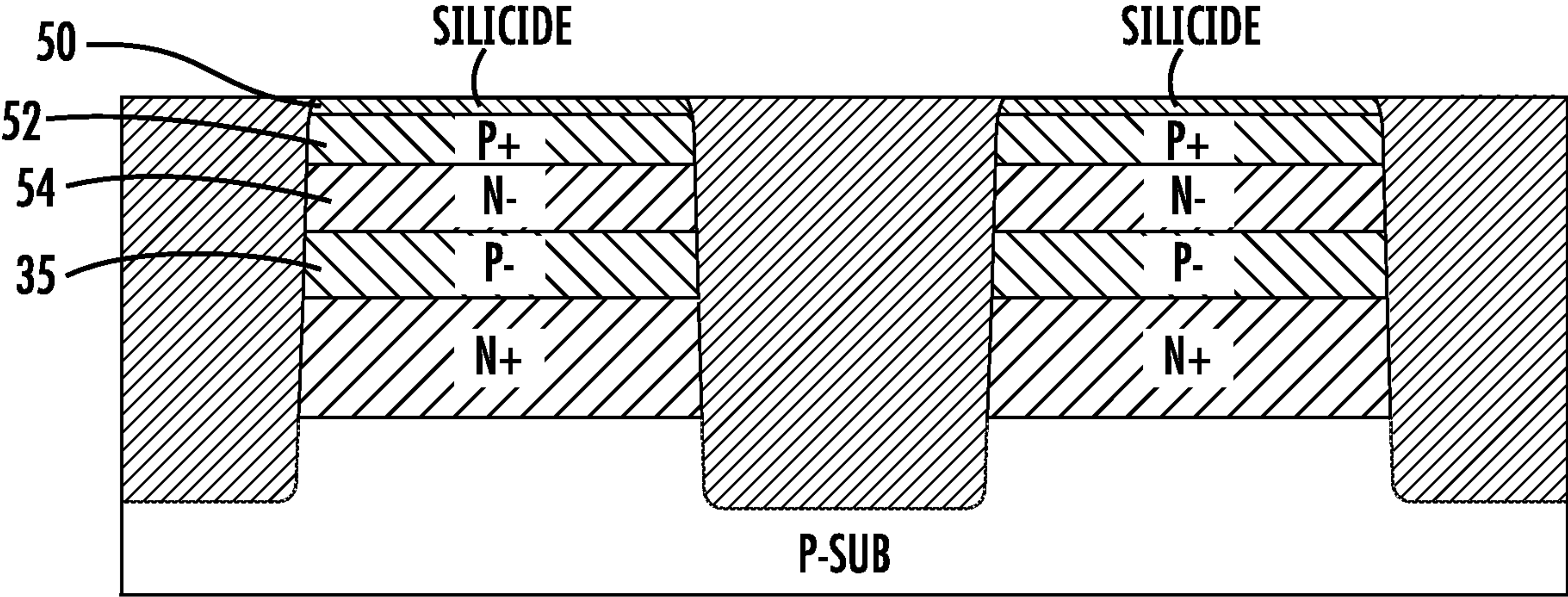
FIG. 8A (A~A')
