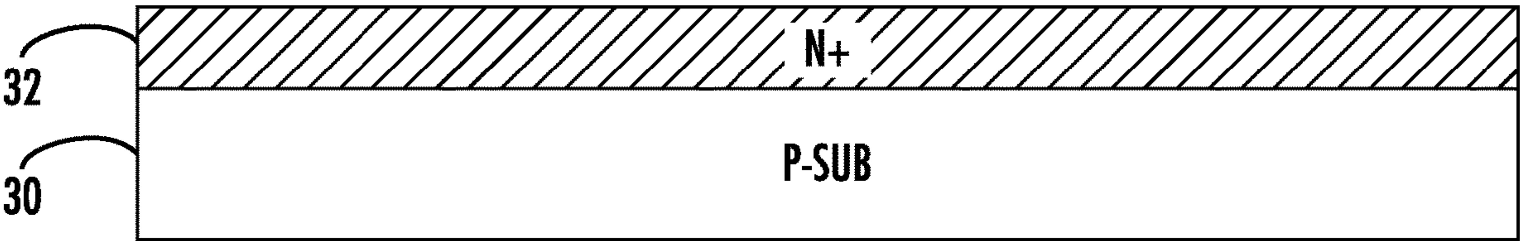
FIG. 3B (B~B')
