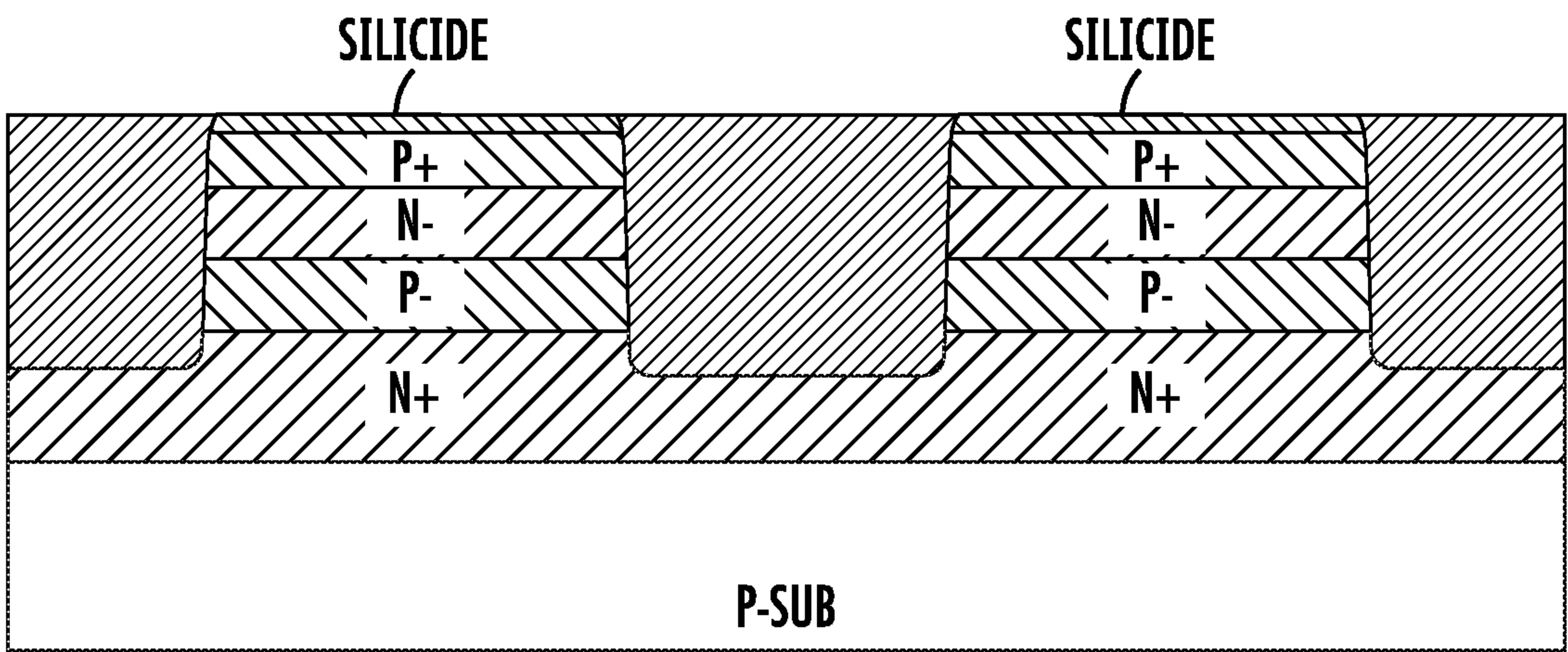
FIG. 17B (B~B')
