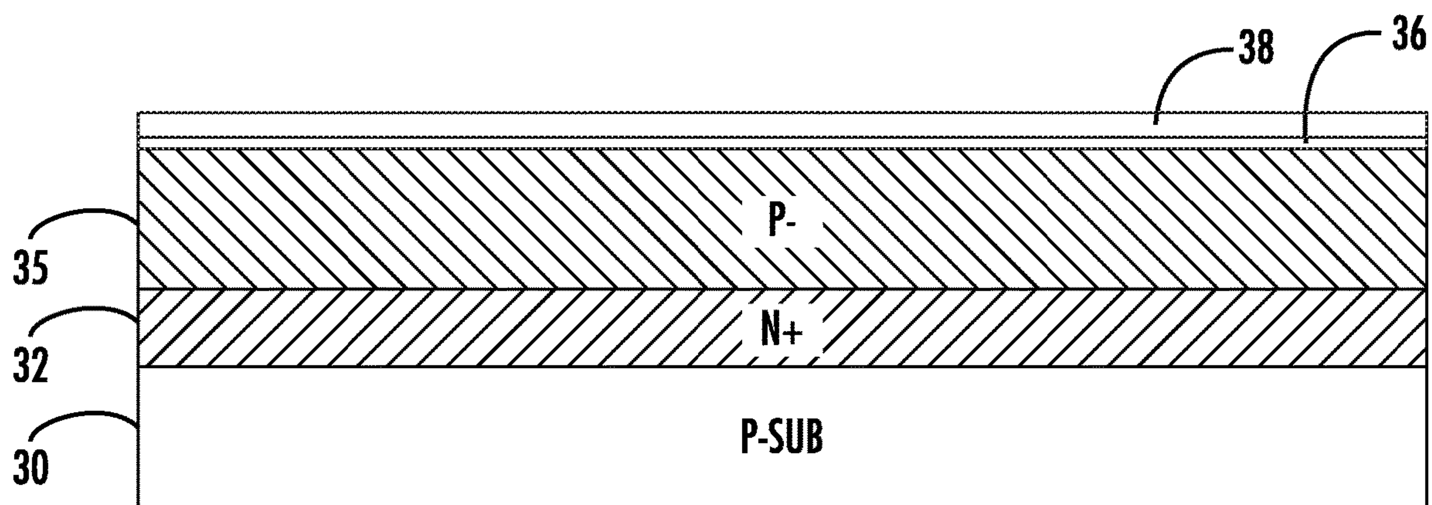
FIG. 5B (B~B')
