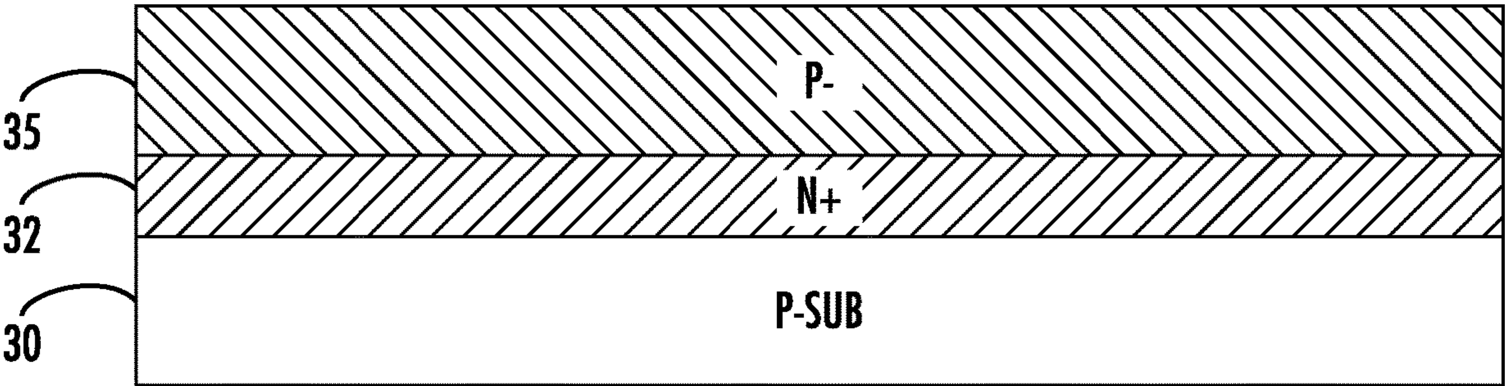
FIG. 4B (B~B')
