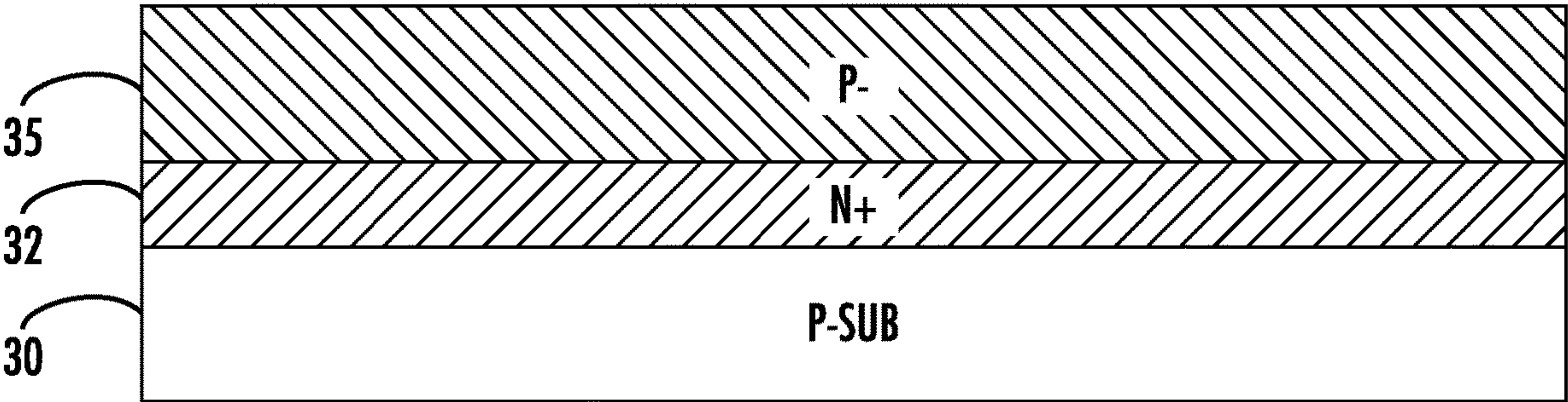
FIG. 4A (A~A')
