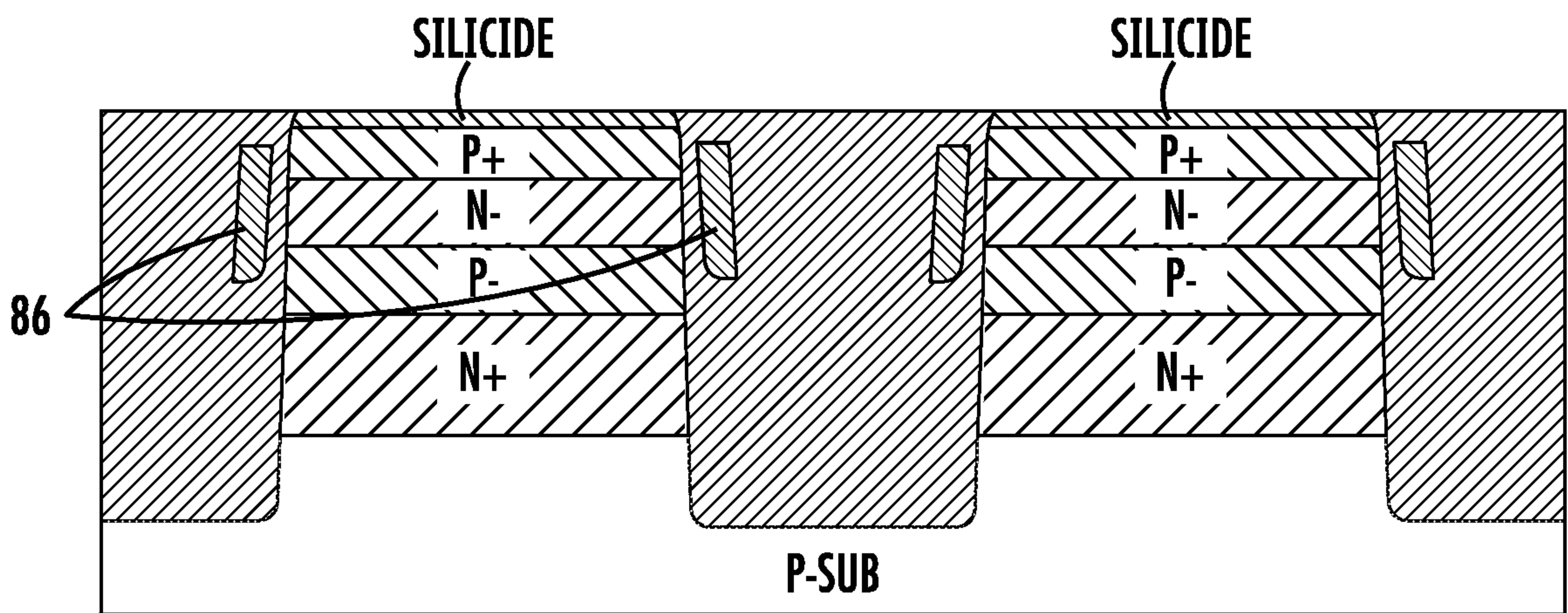
FIG. 17A (A~A')
