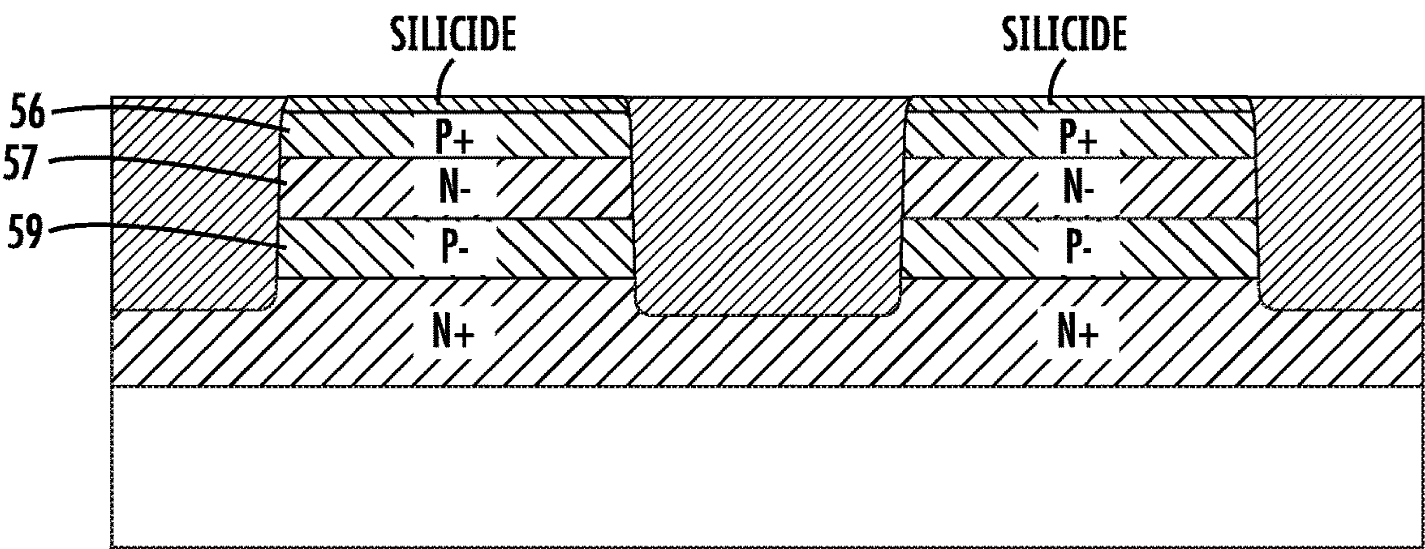
FIG. 15B (B~B')
