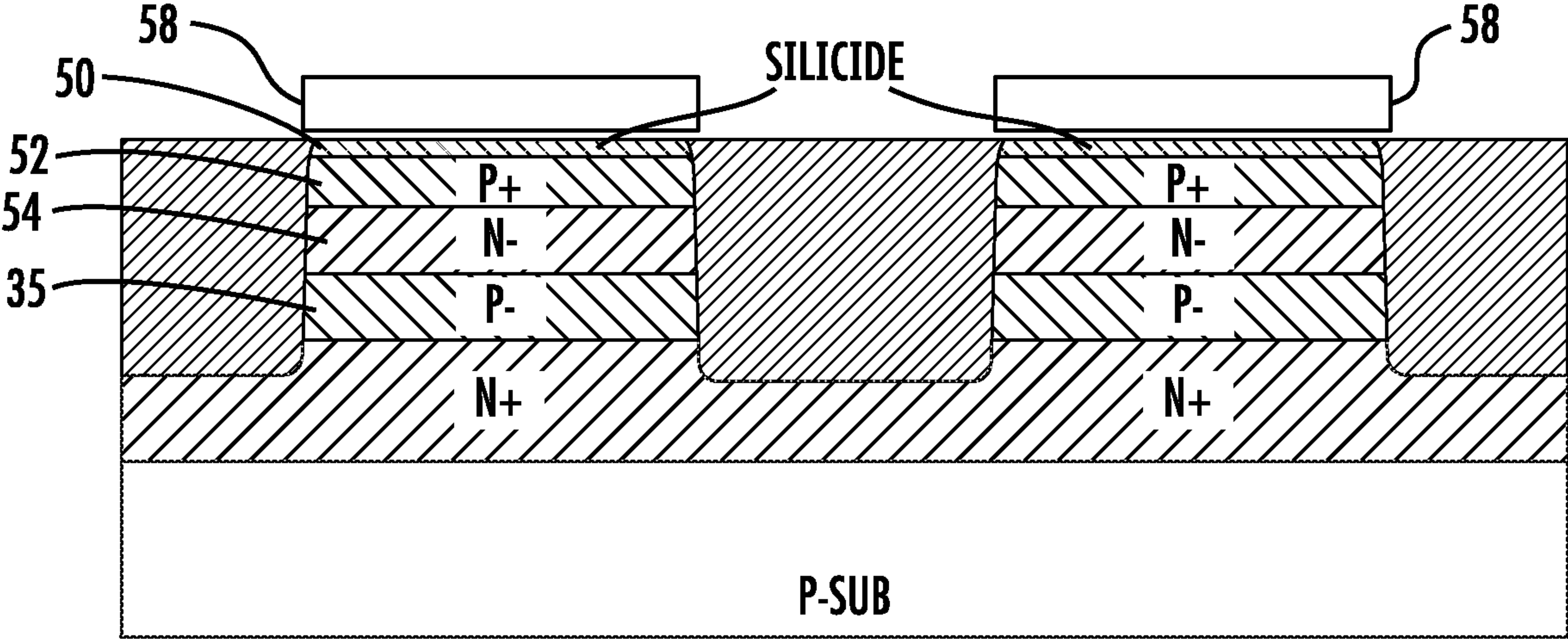
FIG. 8B (B~B')
