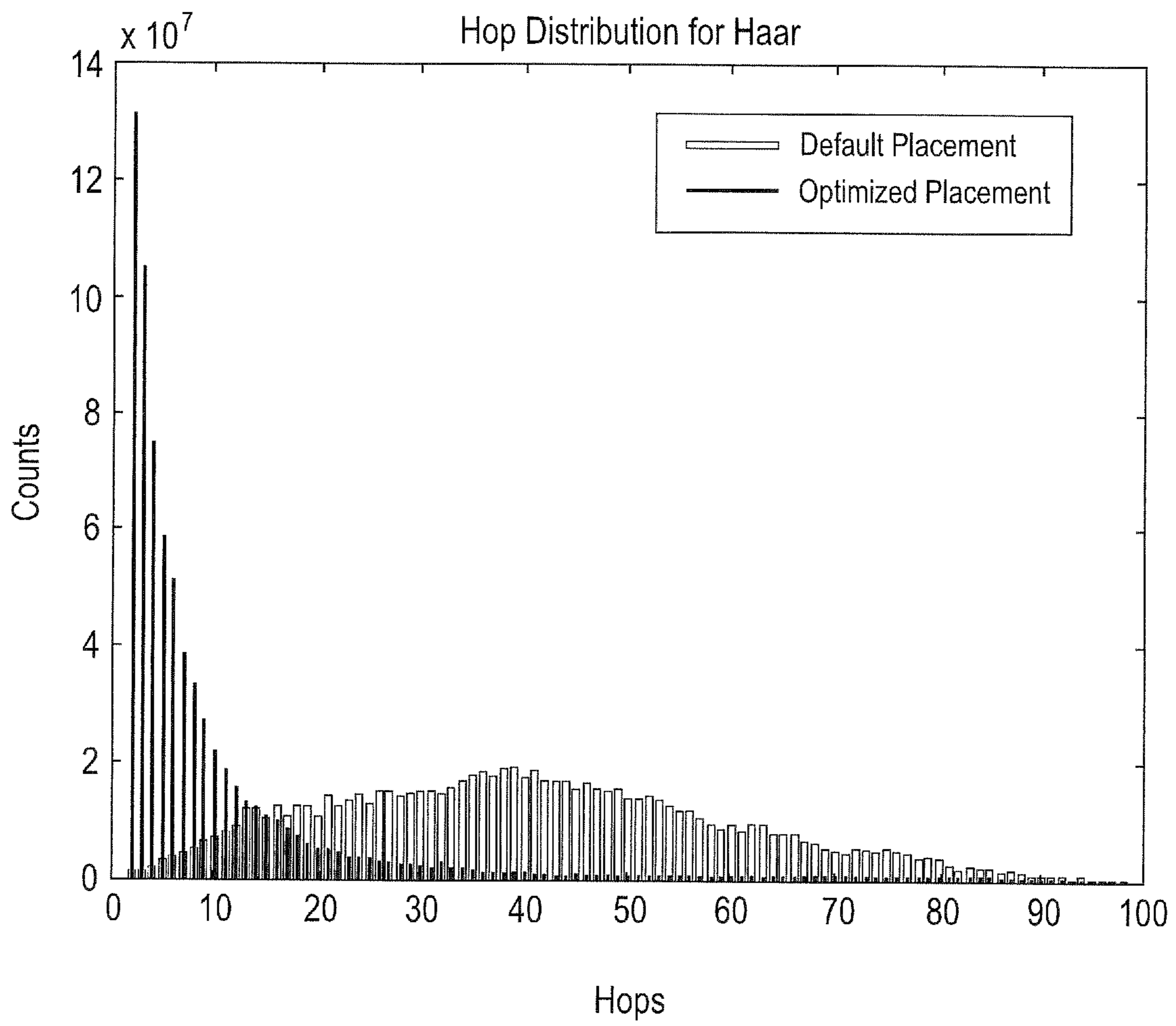
FIG. 8A
