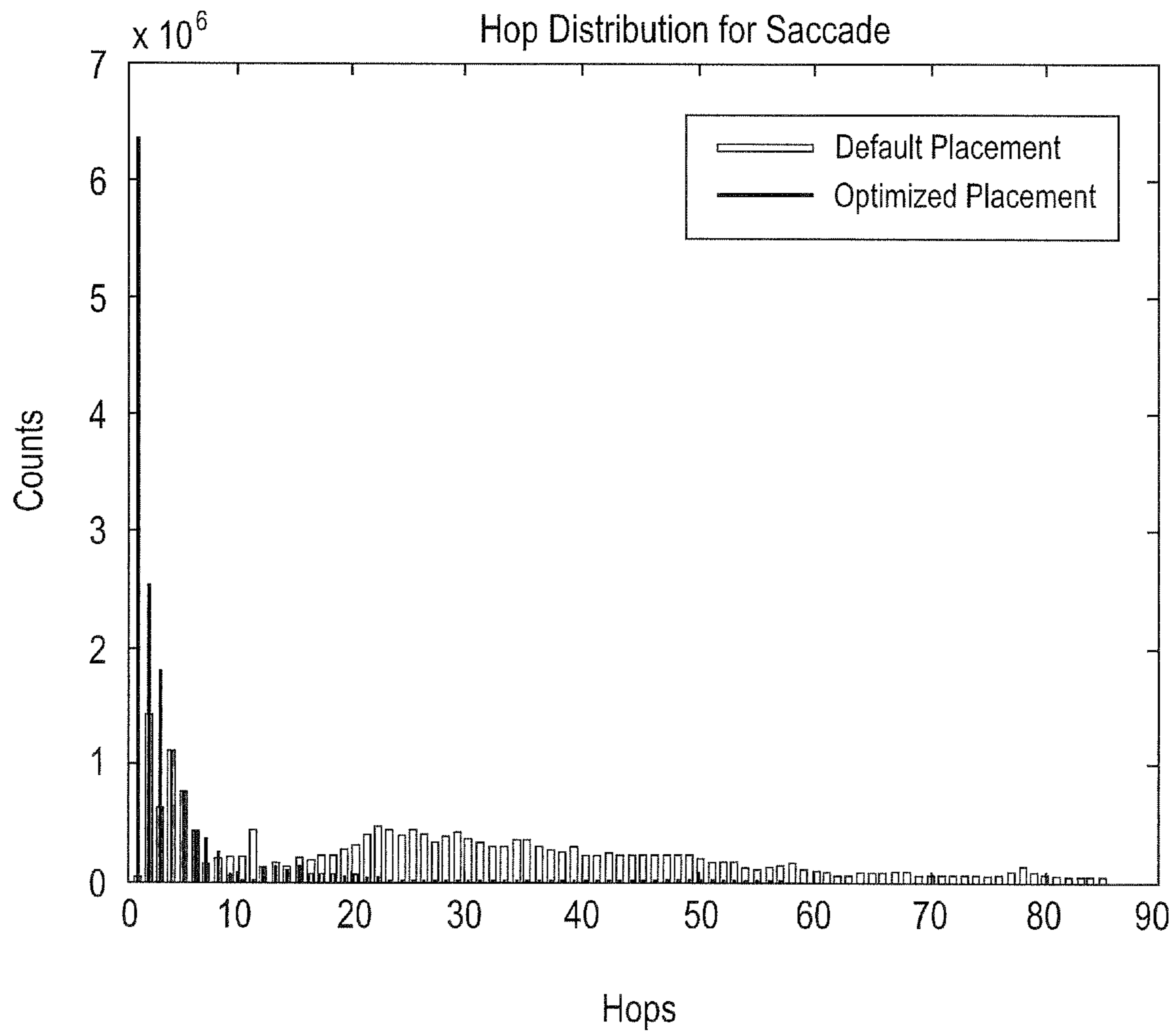
FIG. 8C
