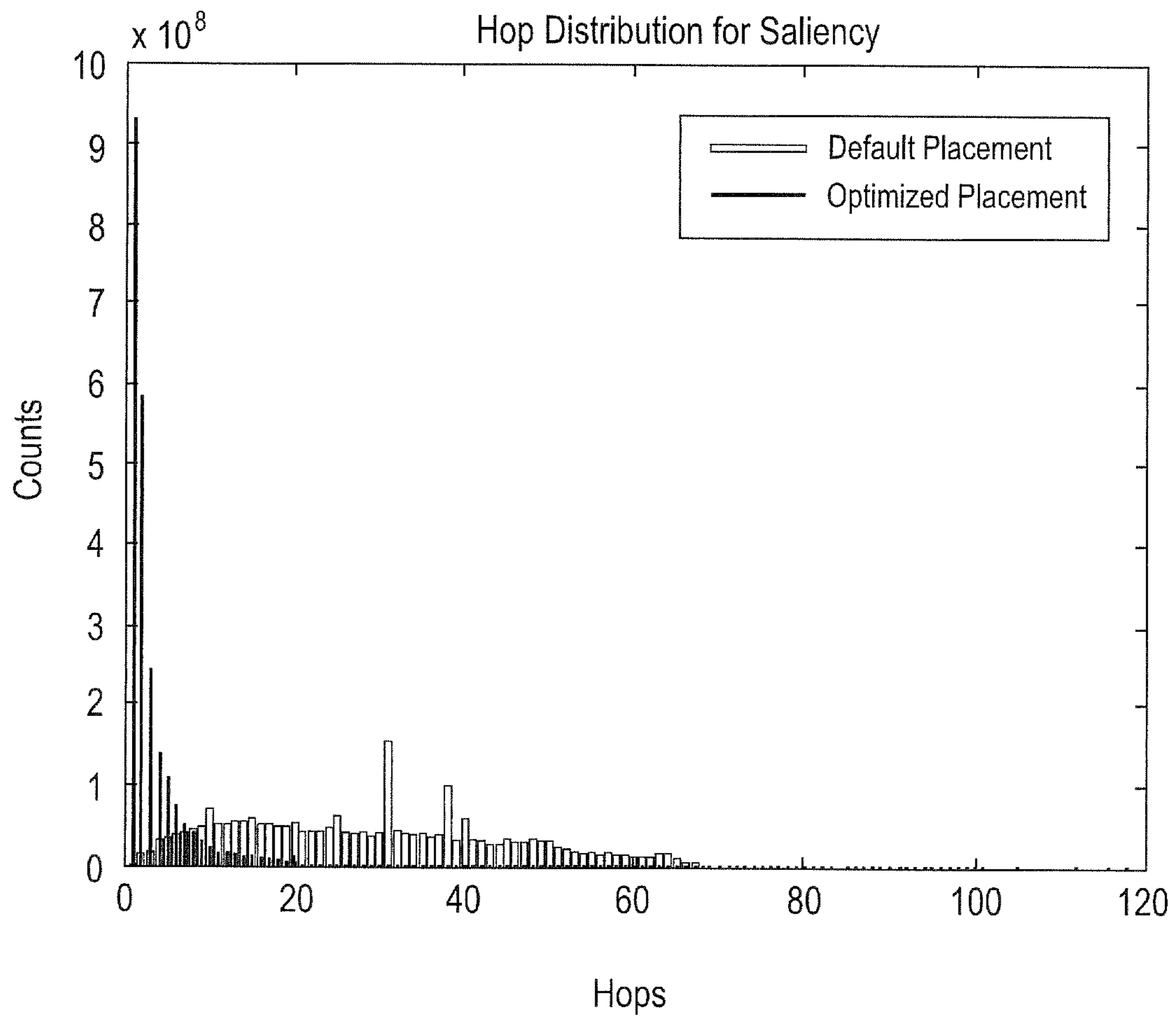
FIG. 8D
