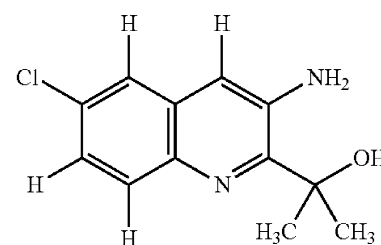
2-(3-amino-6-chloroquinolin-2-yl)propan-2-ol
