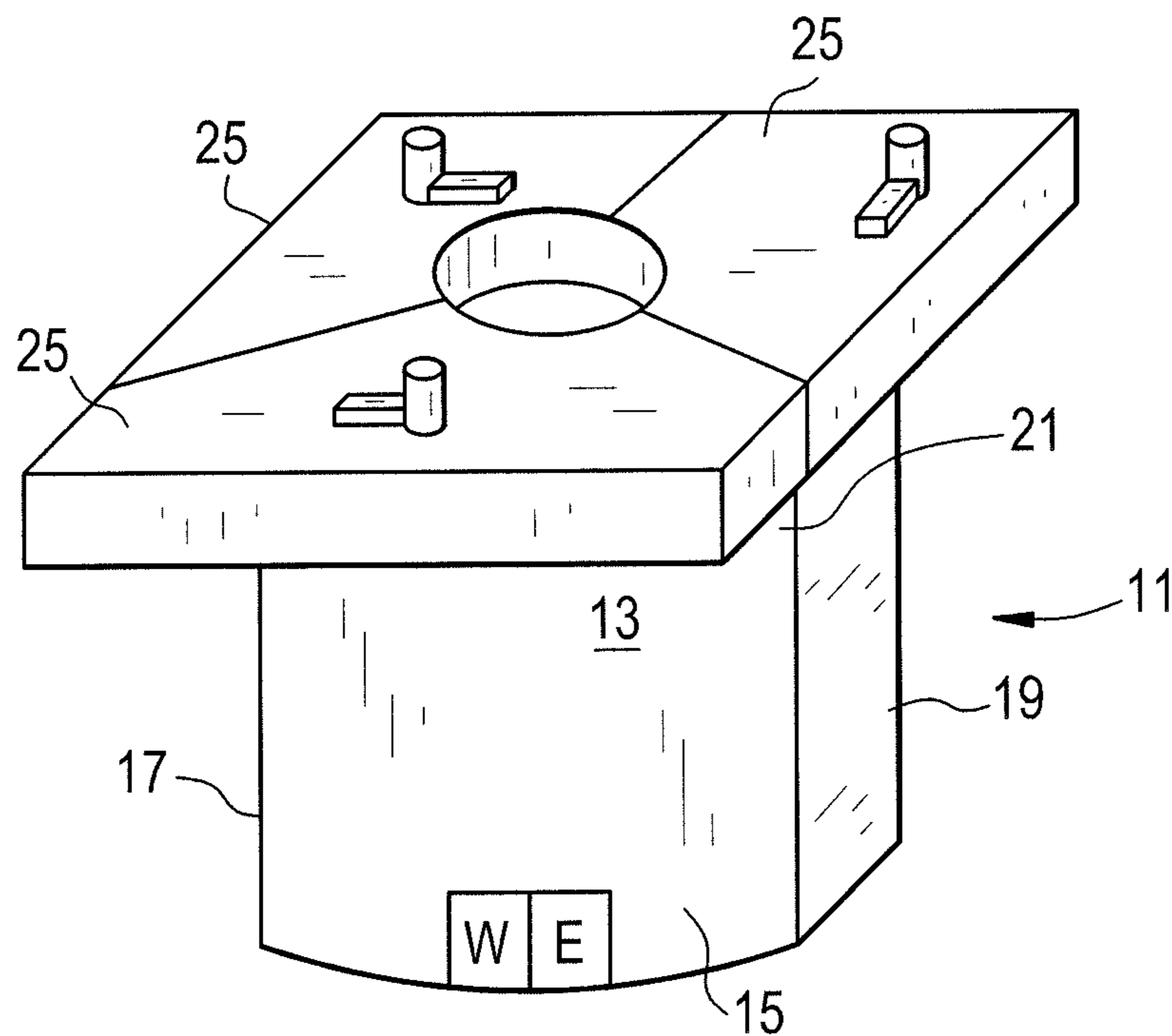
FIG. 2C
