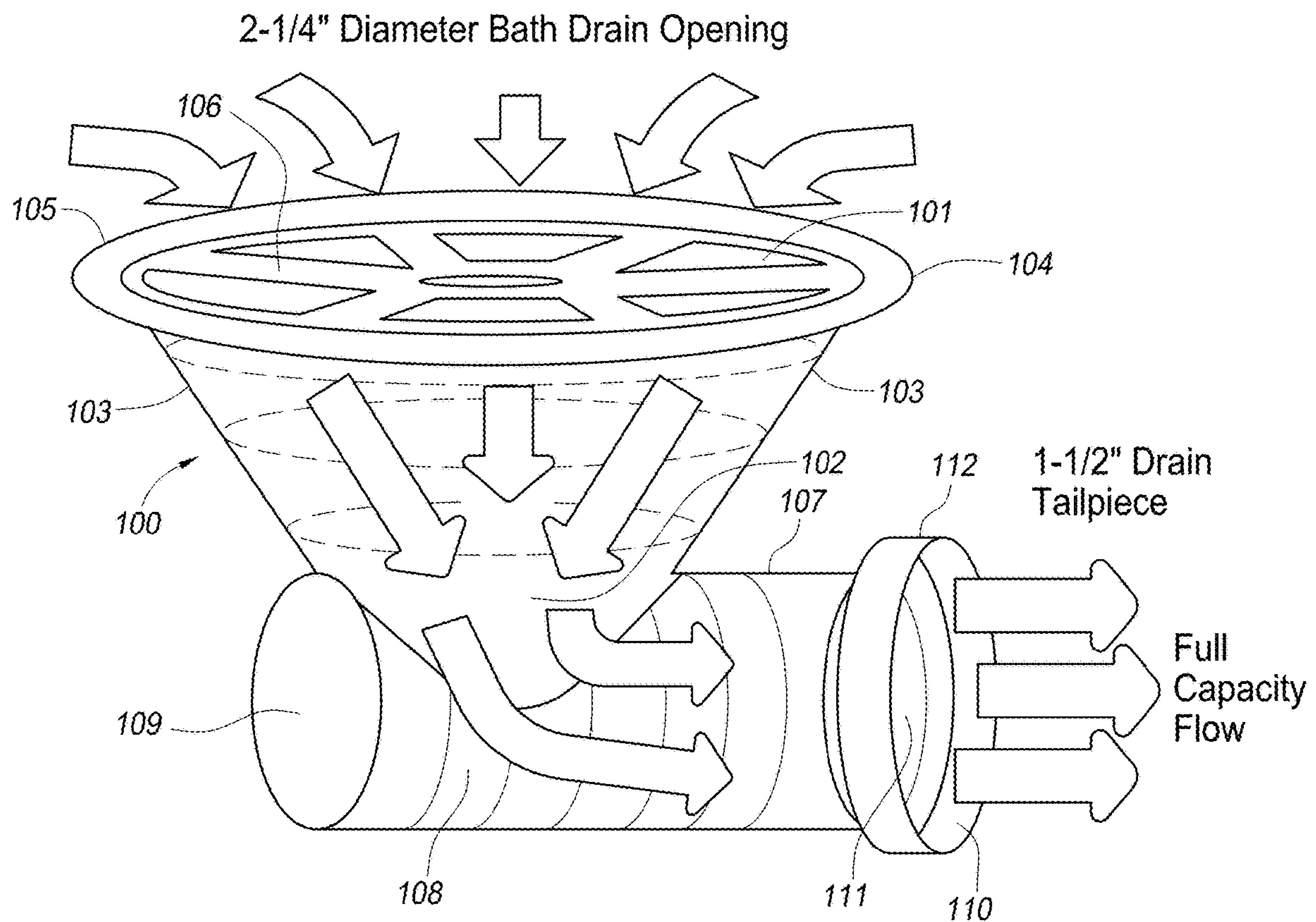
FIG. 1
