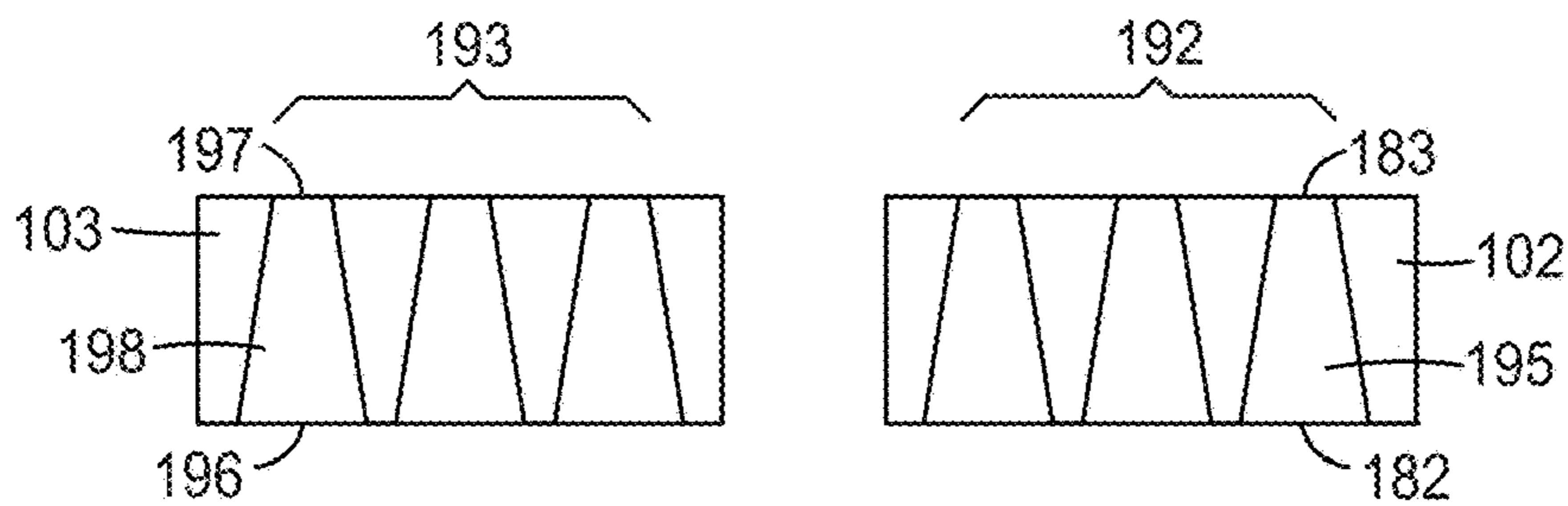
FIG. 1M
