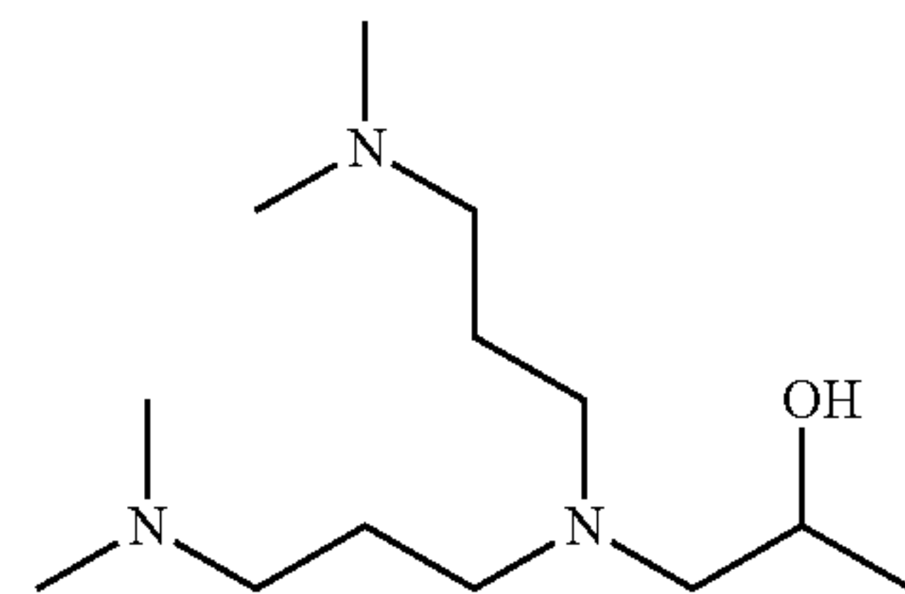
1-(bis(3-(dimethylamino)propyl)amino)propan-2-ol
