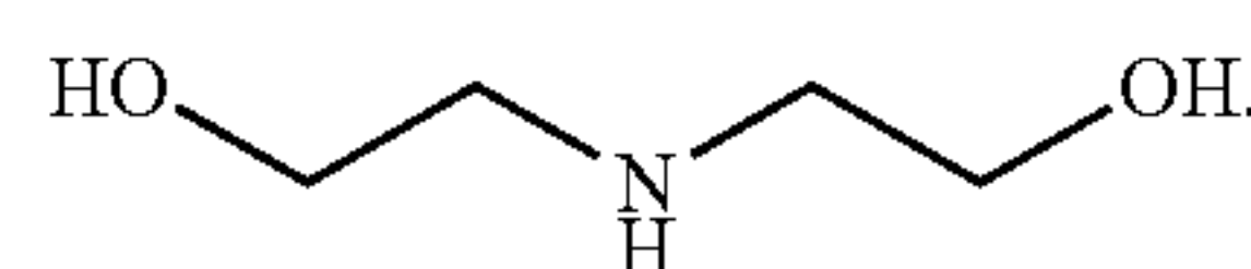
2,2'-azanediylbis(ethan-1-ol)
