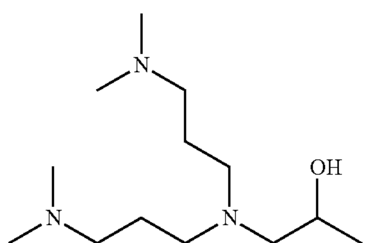
1-(bis(3-(dimethylamino)propyl)amino)propan-2-ol
