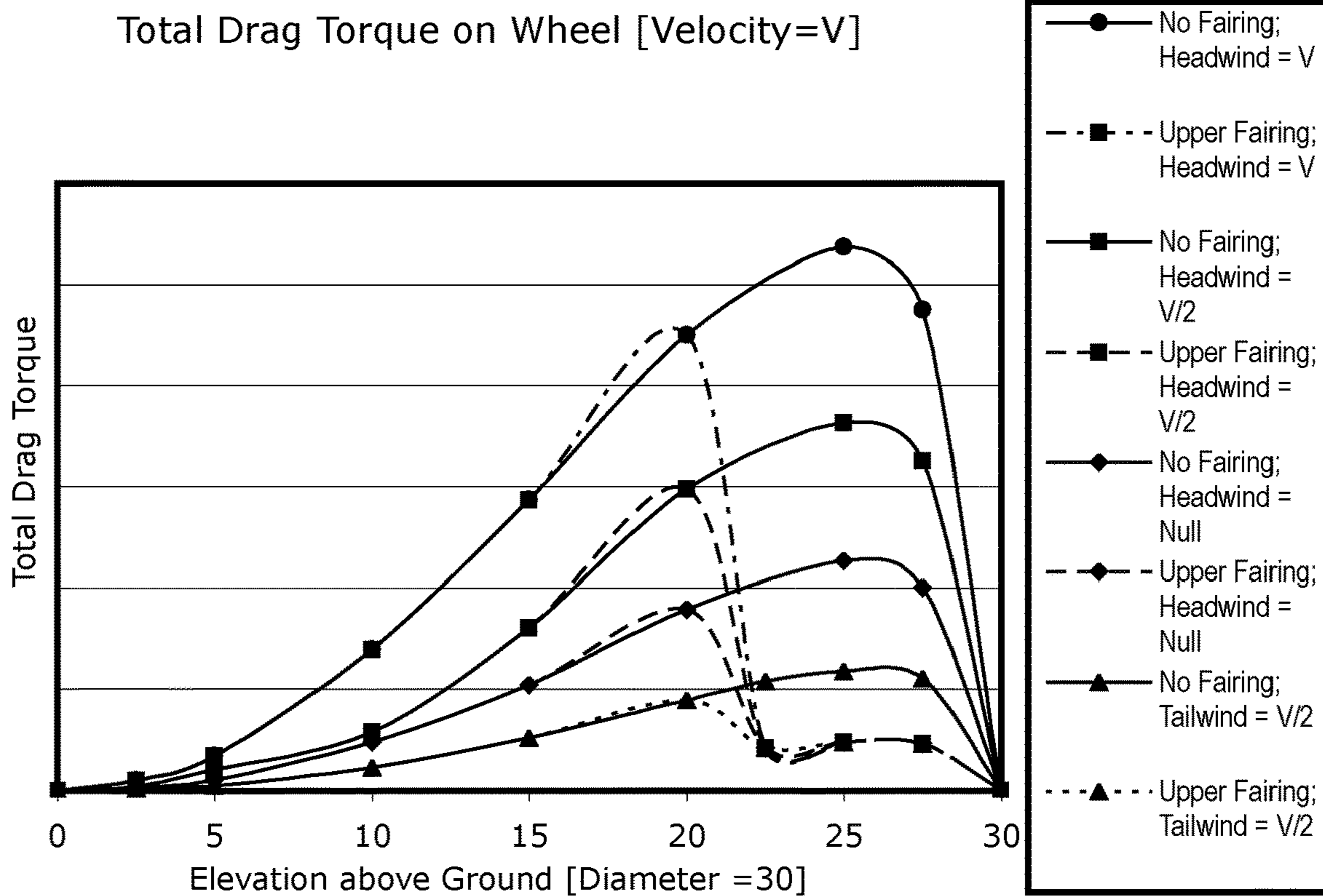
FIG. 18
