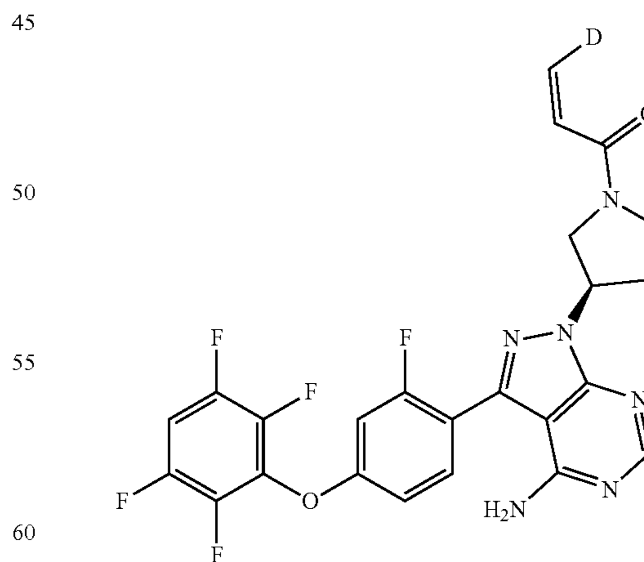
(Z)-1-((R)-3-(4-amino-3-(2-fluoro-4-(3-fluorophenoxy)phenyl)-1H-pyrazolo[3,4-d]pyrimidin-1-yl)pyrrolidin-1-yl)-3-deuterium-prop-2-en-1-one
