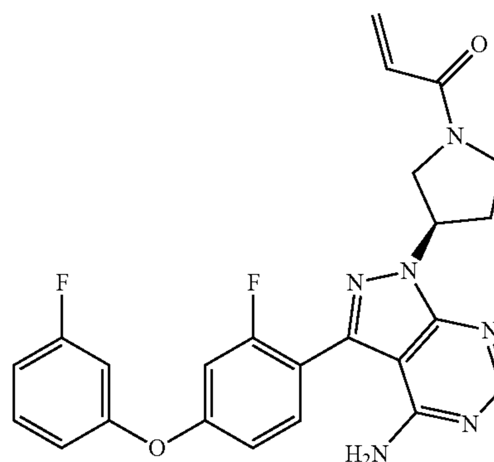
1-((R)-3-(4-amino-3-(2-fluoro-4-(3-fluorophenoxy)phenyl)-1H-pyrazolo[3,4-d]pyrimidin-1-yl)pyrrolidin-1-yl)prop-2-en-1-one
