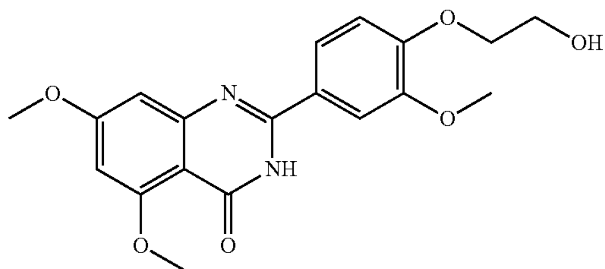
2-(4-(2-hydroxyethoxy)-3-methoxyphenyl)-5,7-dimethoxyquinazolin-4(3H)-one
