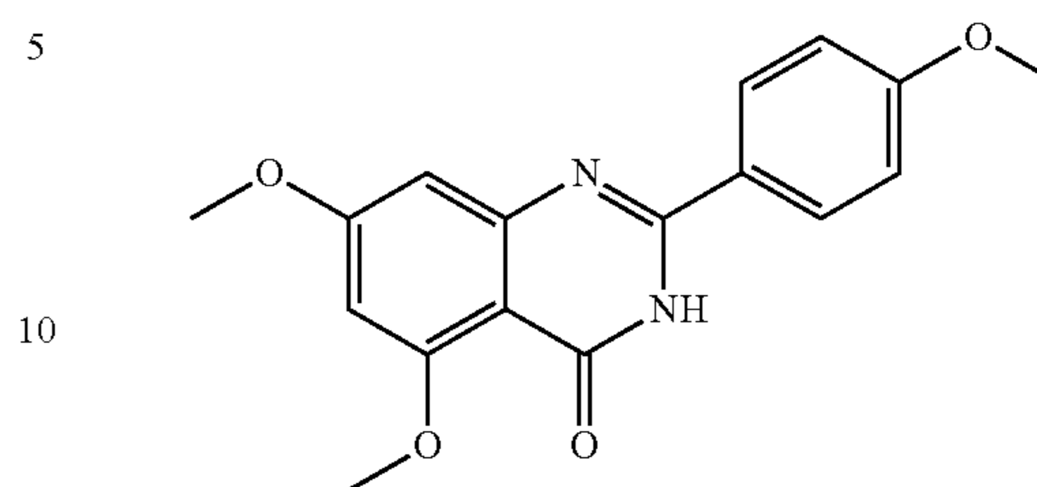
5,7-dimethoxy-2-(4-methoxyphenyl)quinazolin-4(3H)-one
