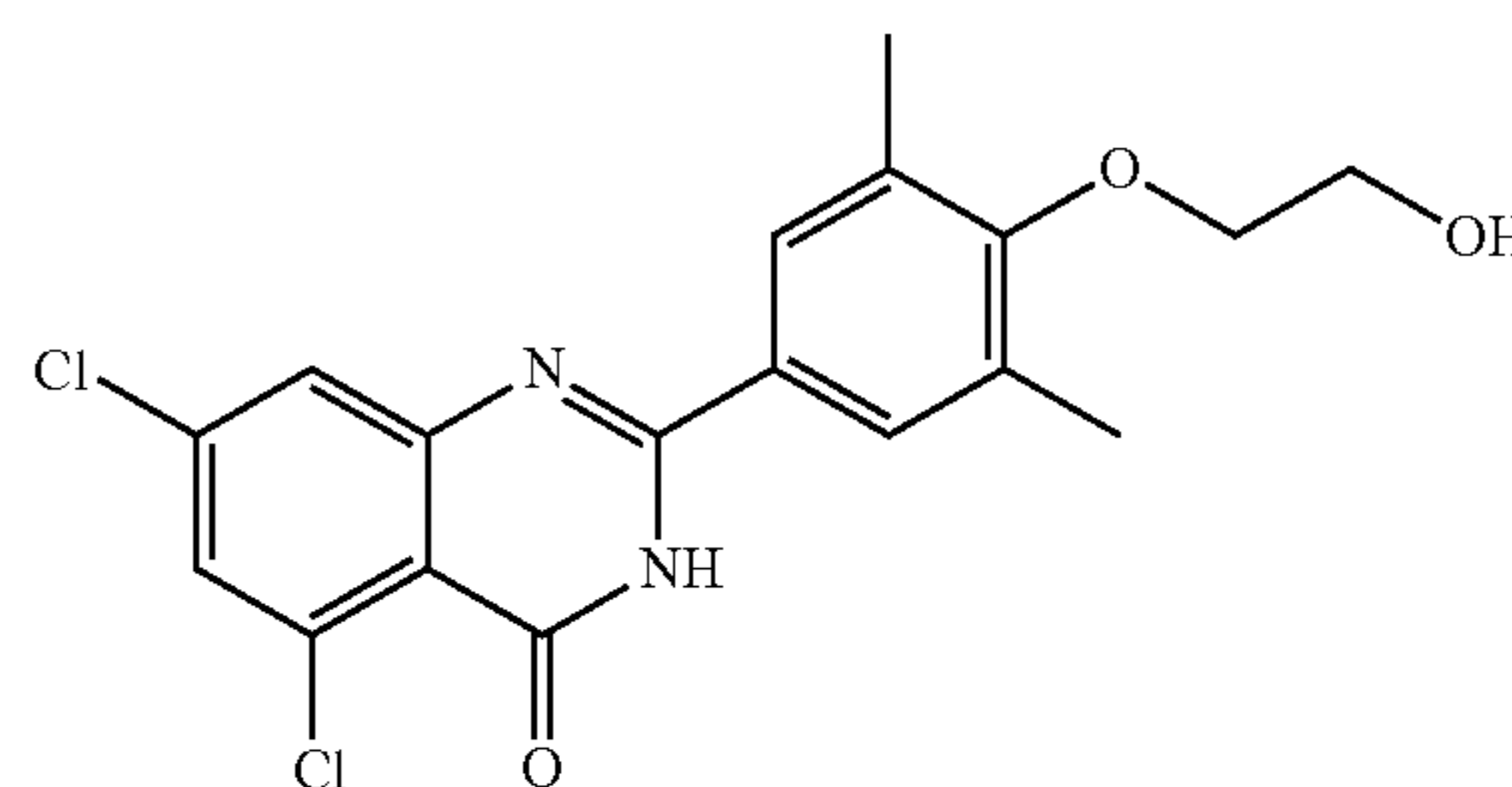
5,7-dichloro-2-(4-(2-hydroxyethoxy)-3,5-dimethylphenyl)quinazolin-4(3H)-one
