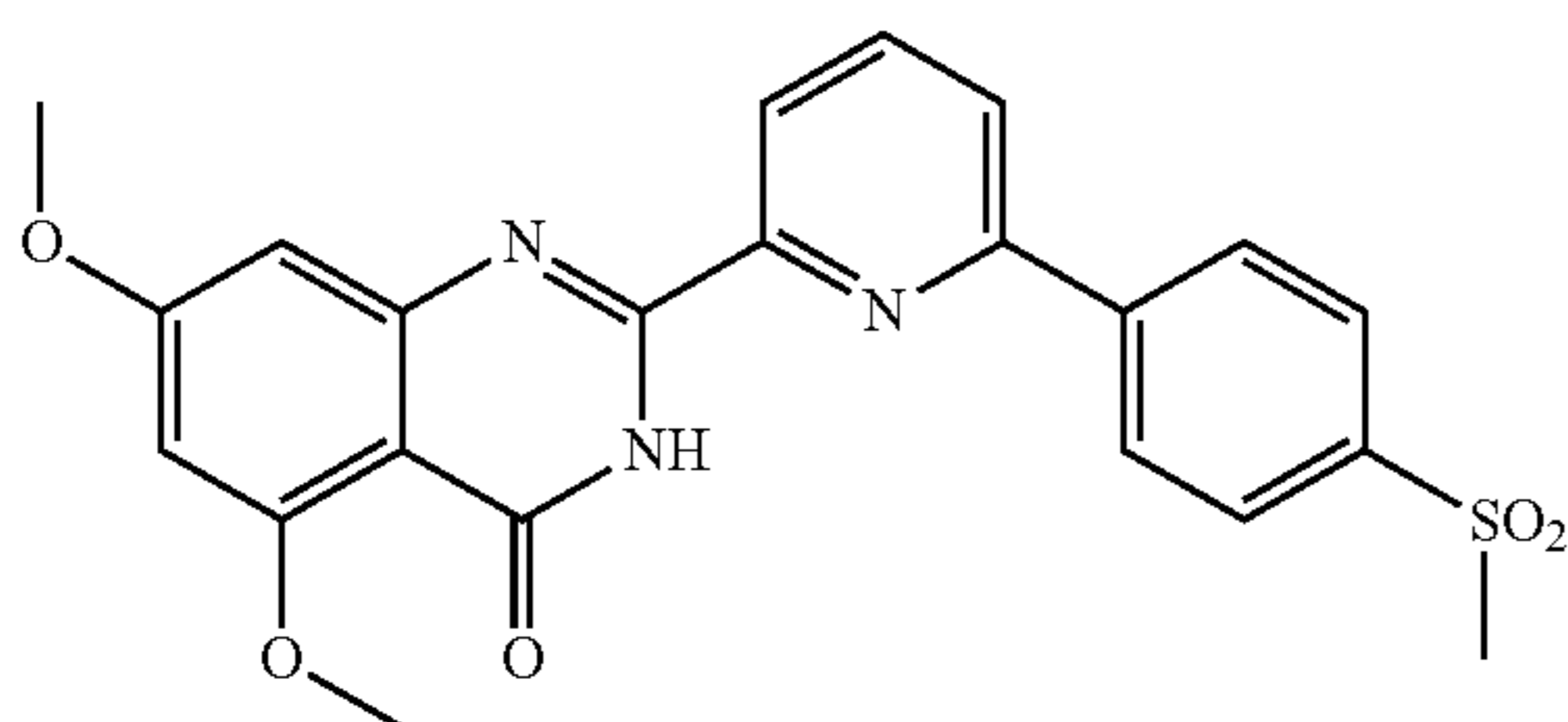
5,7-dimethoxy-2-(6-(4-(methylsulfonyl)phenyl)pyridin-2-yl)quinazolin-4(3H)-one
