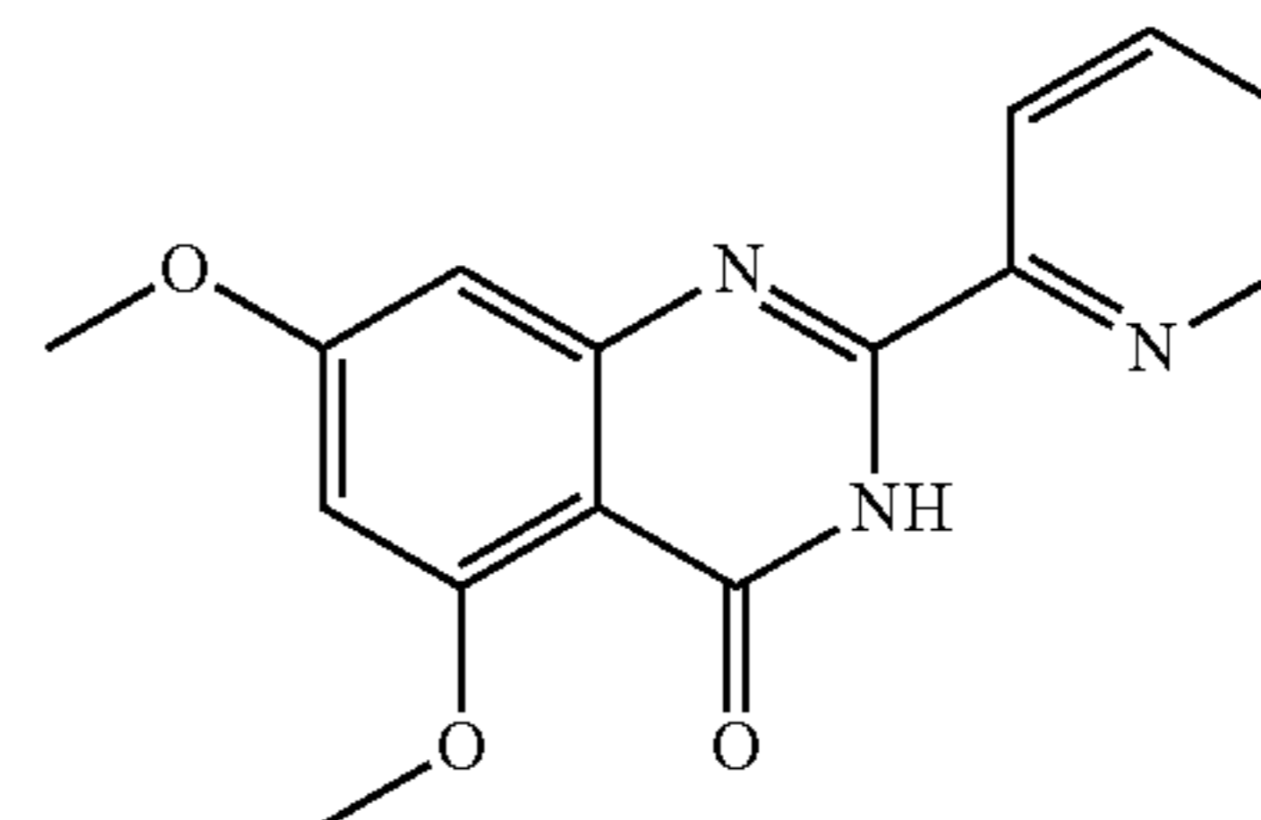
5,7-dimethoxy-2-(pyridin-2-yl)quinazolin-4(3H)-one
