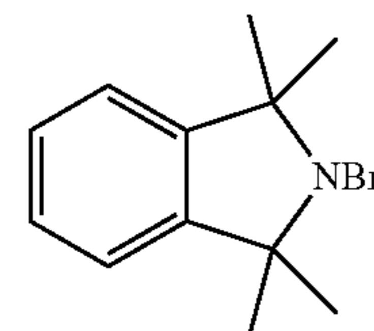
2-Benzyl-1,1,3,3-tetramethylisindoline (16)
