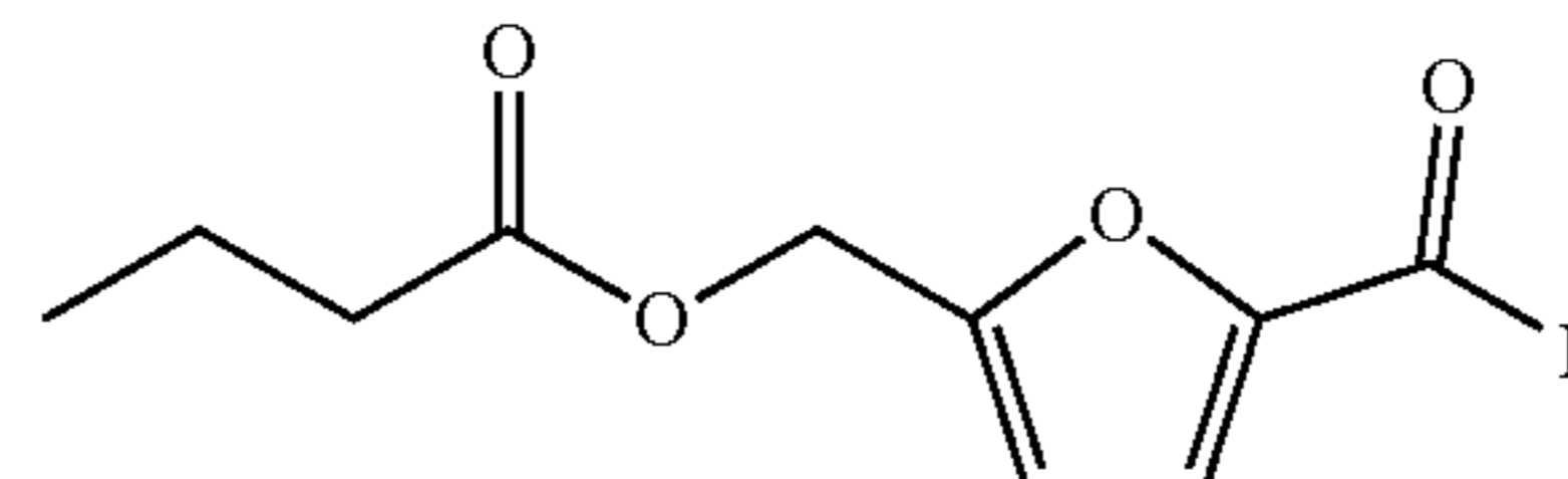
5-butyroxyethylfurfural
