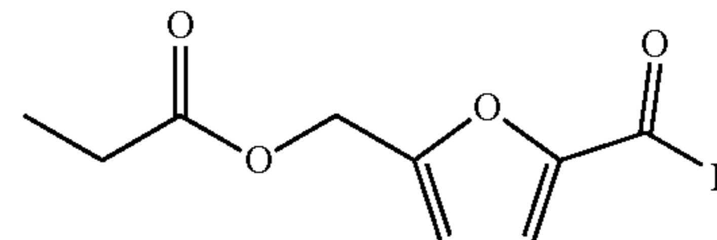
5-propionoxymethylfurfural
