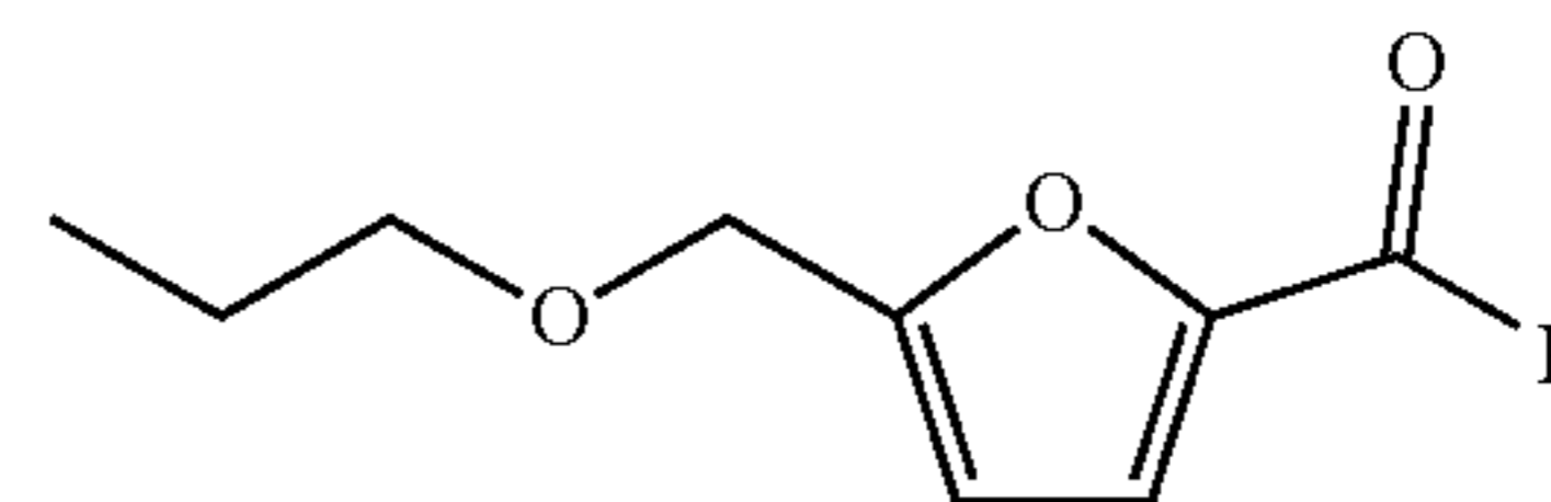
5-propoxymethylfurfural
