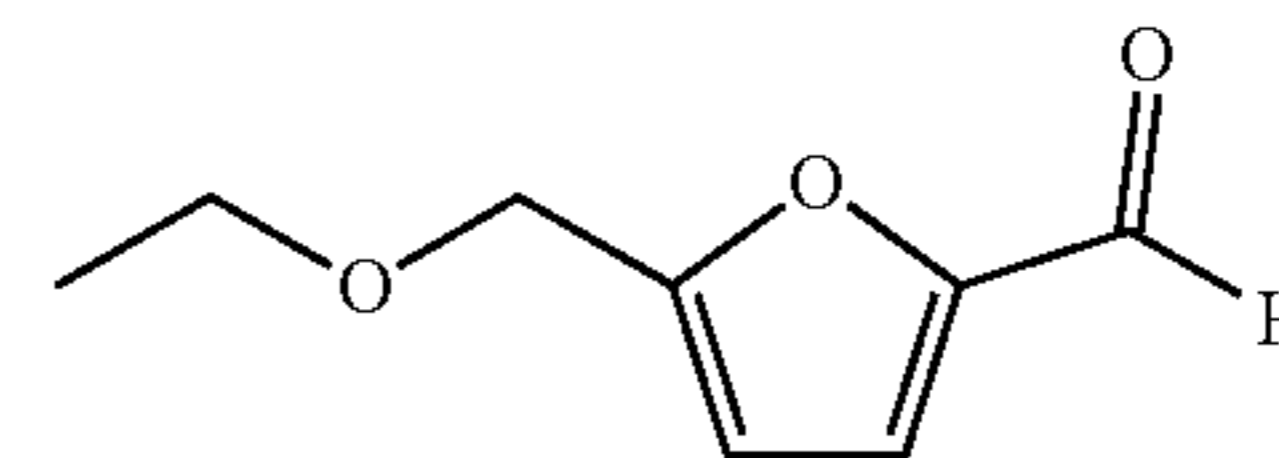
5-ethoxymethylfurfural
