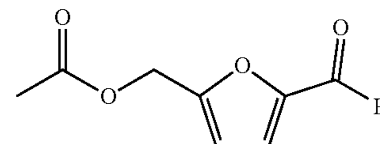
5-acetoxymethylfurfural
