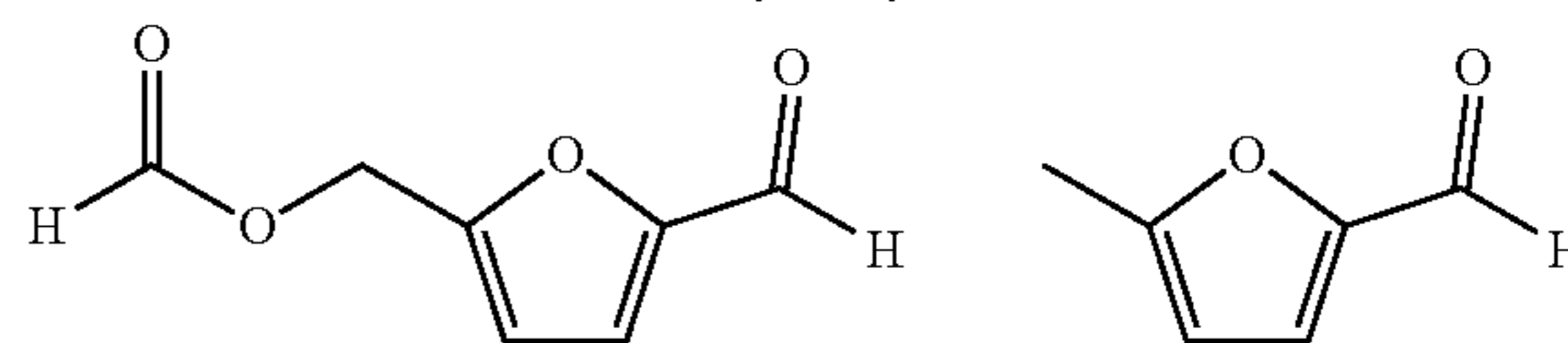
5-formoxymethylfurfural
