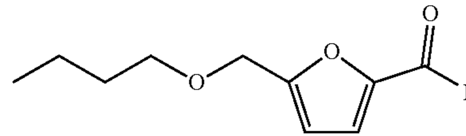
5-butoxymethylfurfural
