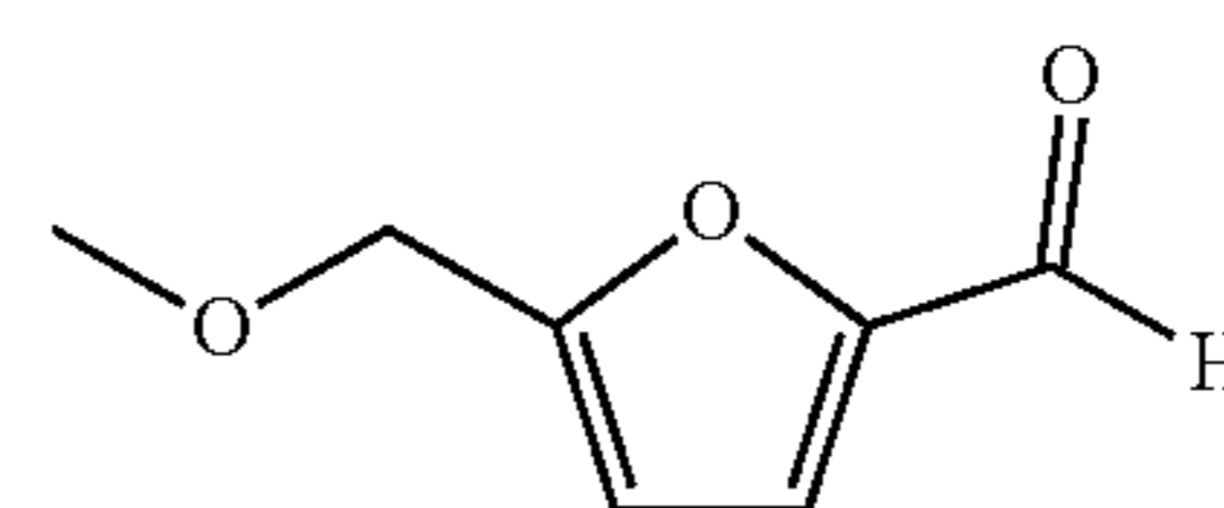
5-methoxymethylfurfural
