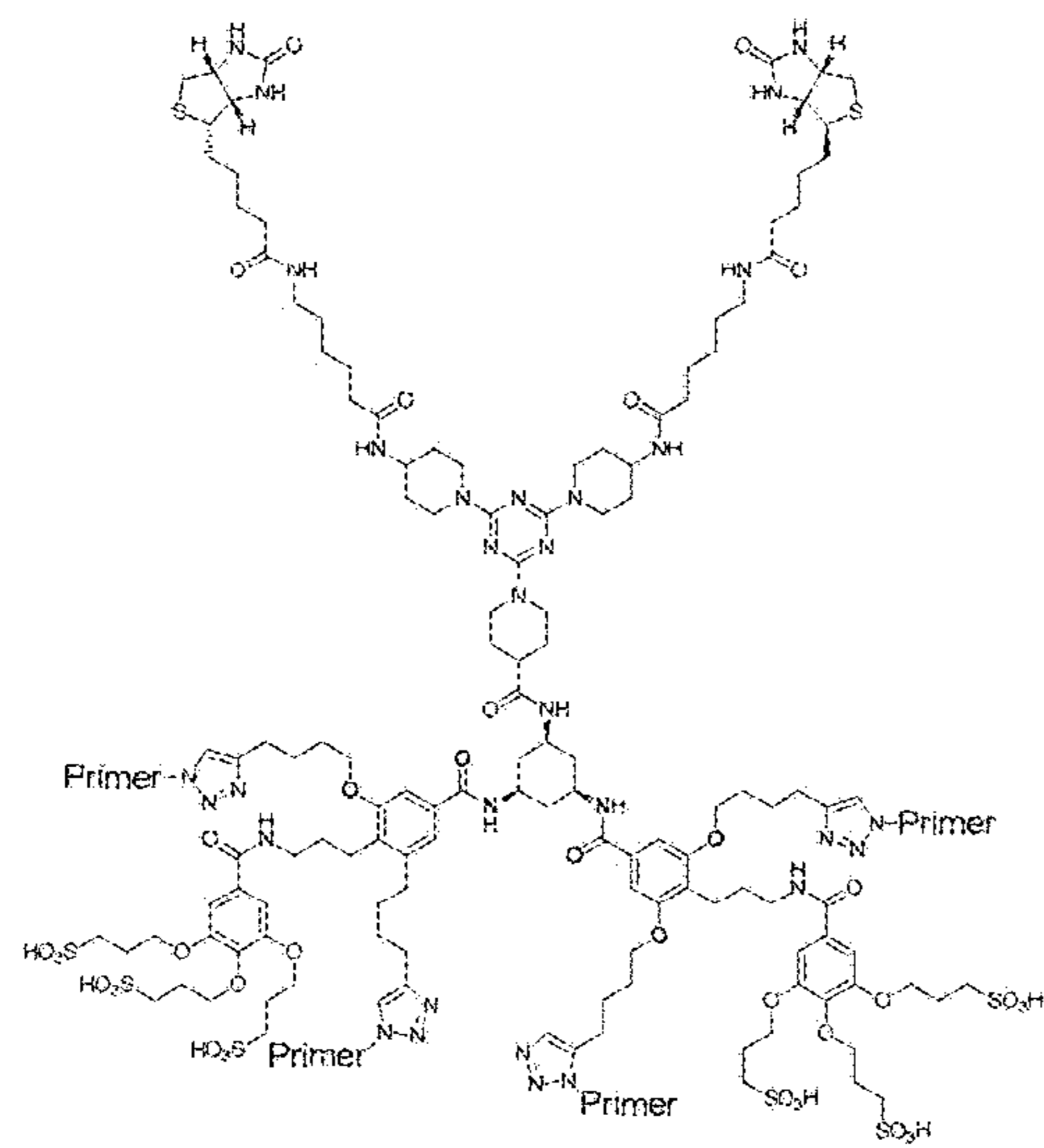
6-Arm A-Ball SC2 Scaffold
