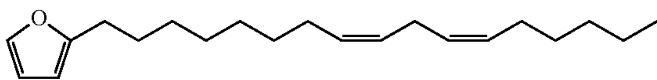
2-(8Z, 11Z-heptadecadienyl)furan
