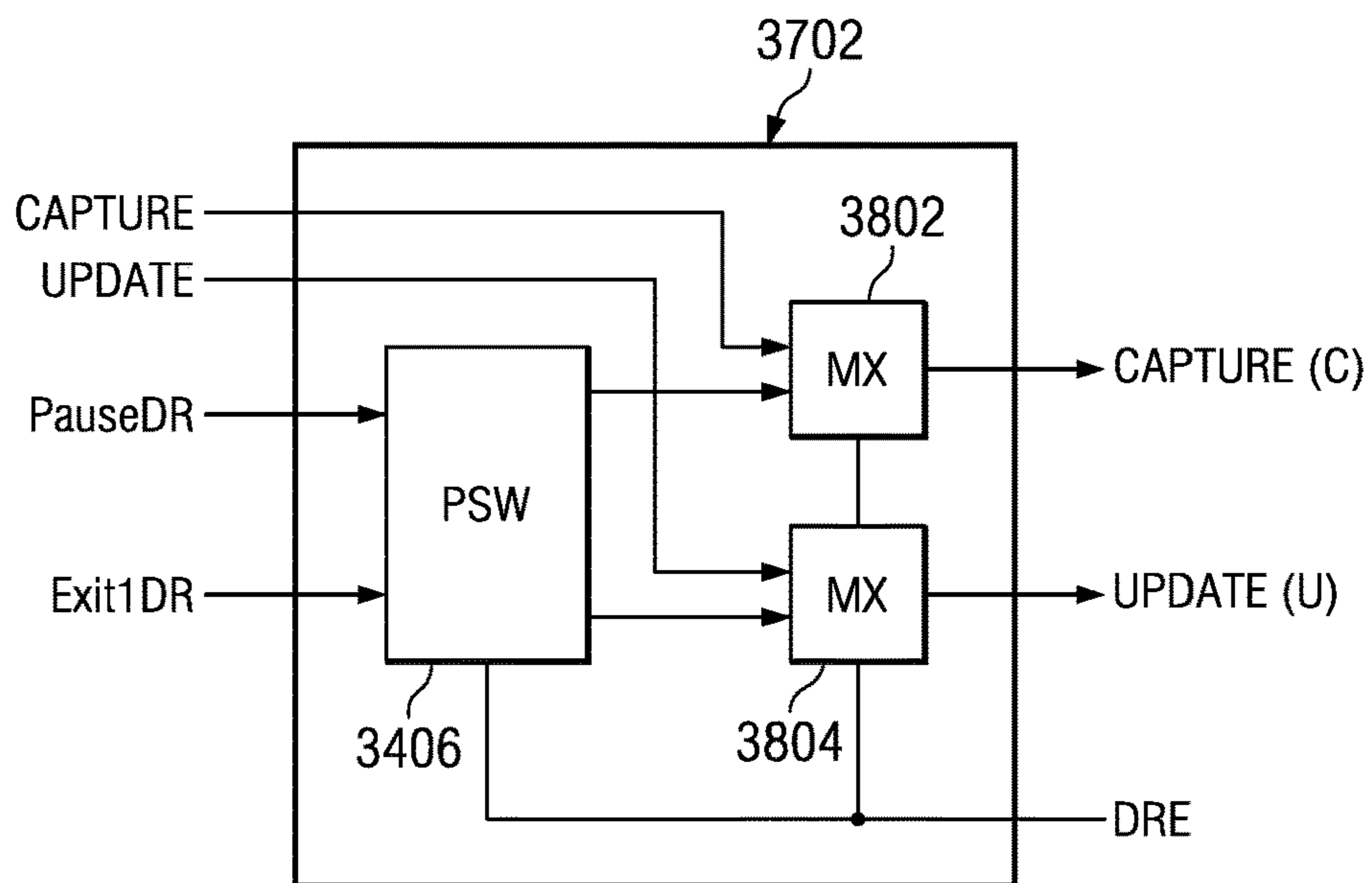
FIG. 38
