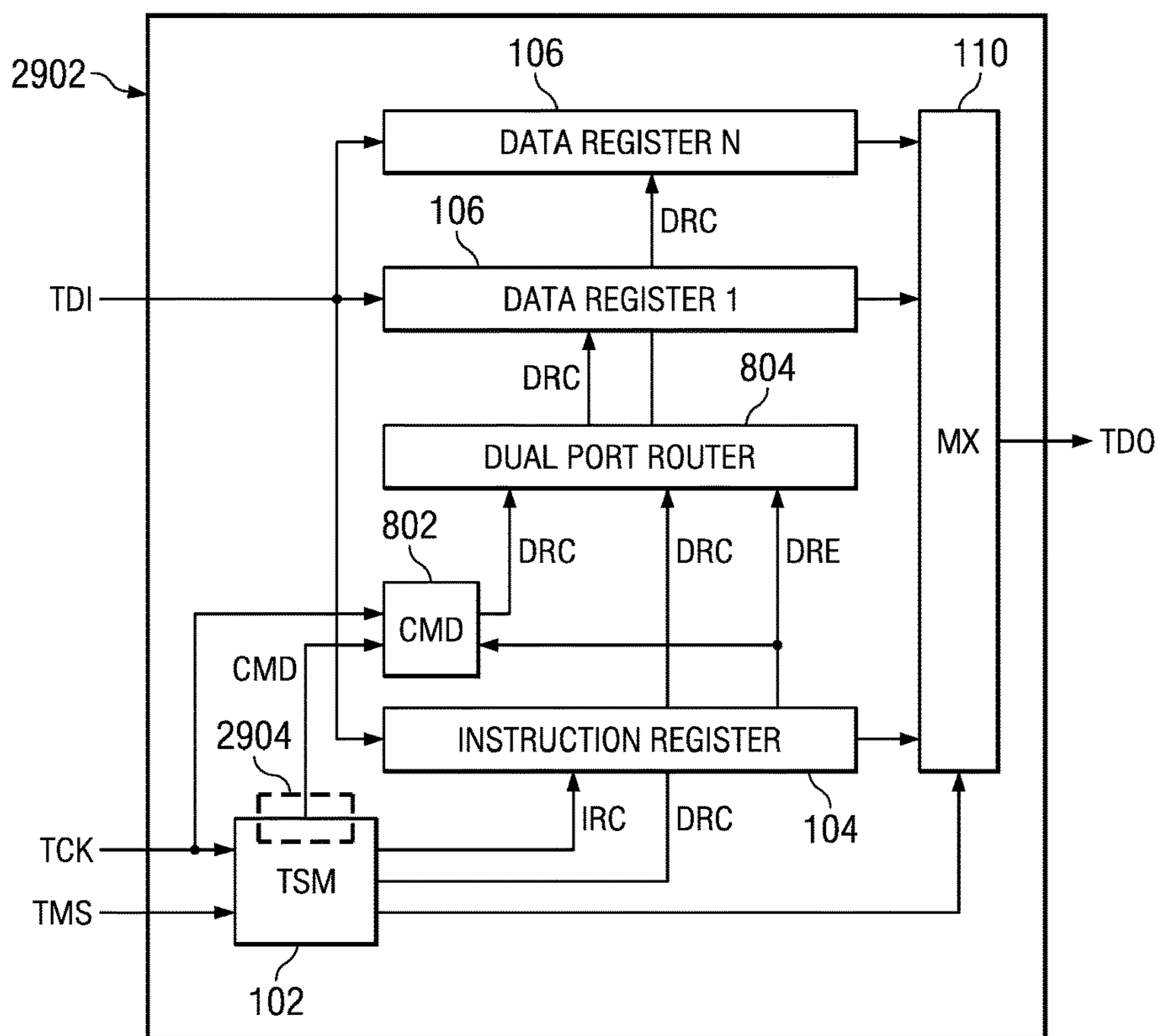
FIG. 29A
