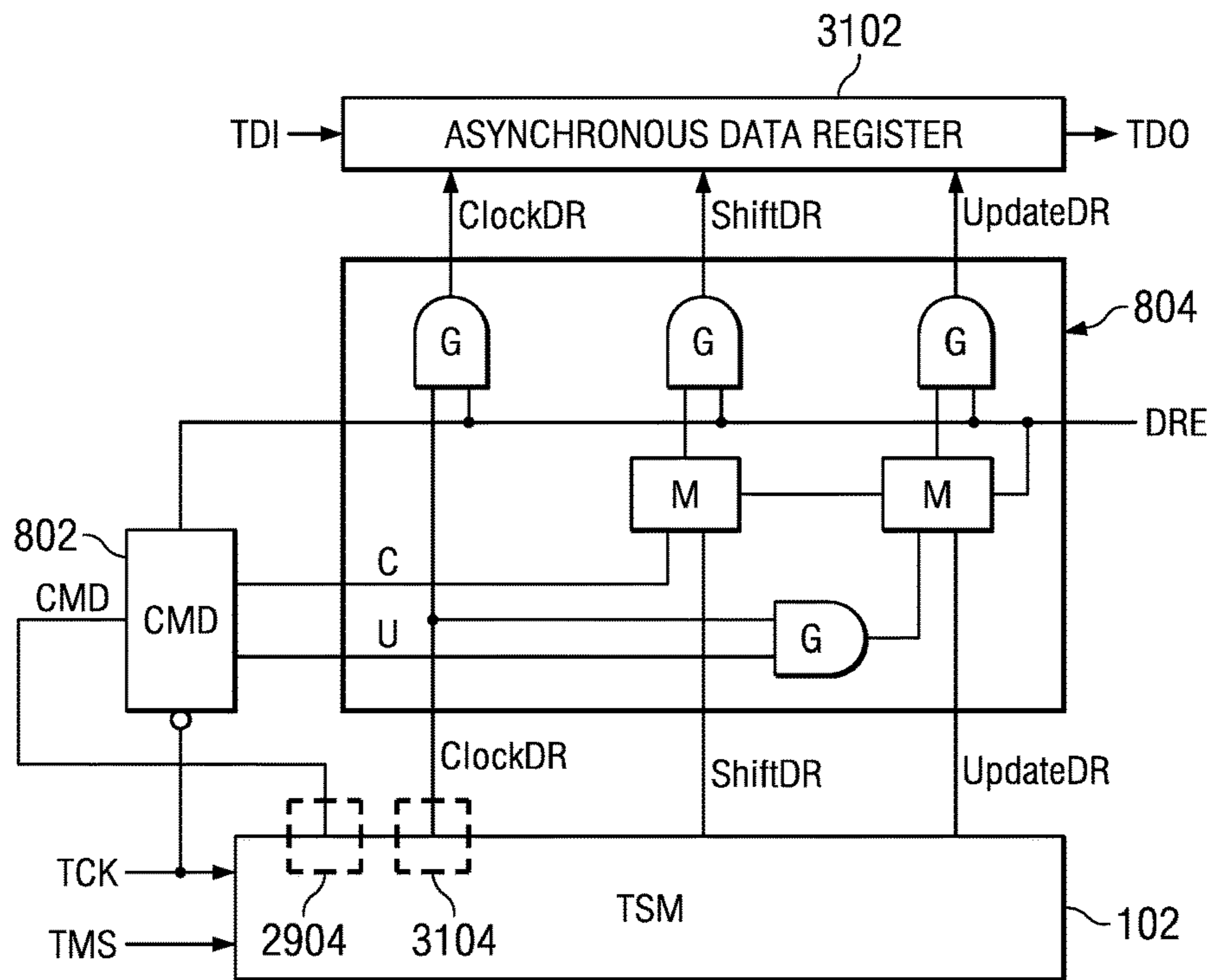
FIG. 31
