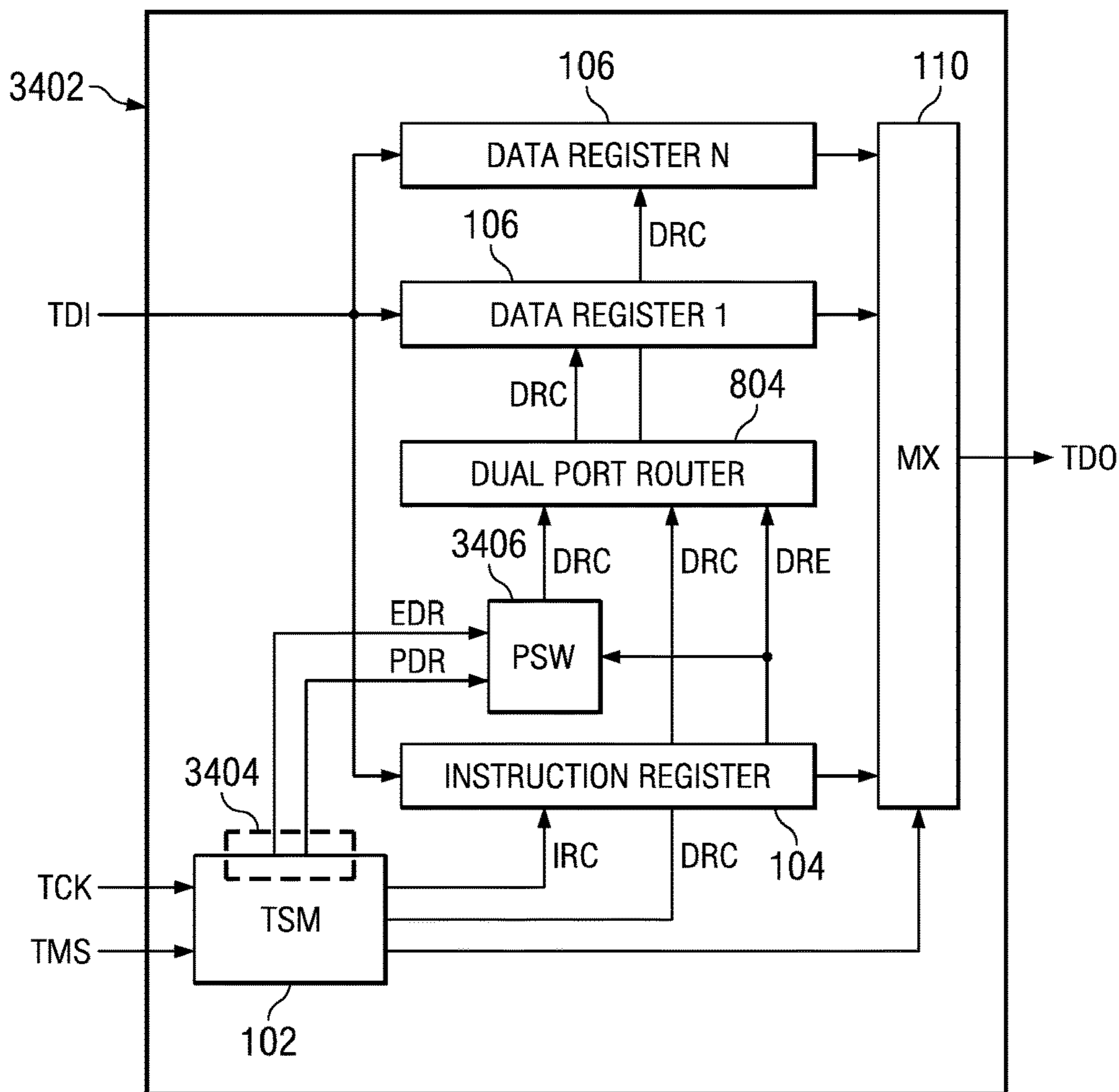
FIG. 34A
