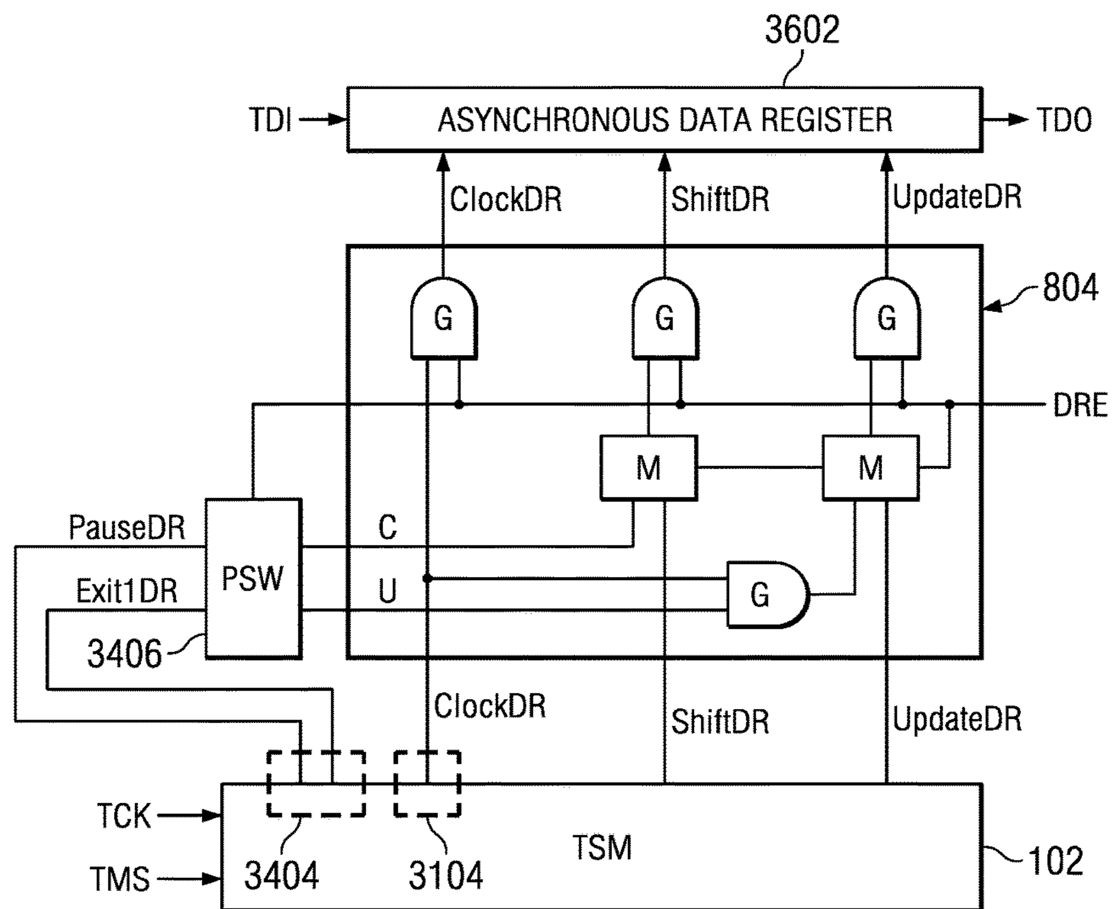
FIG. 36
