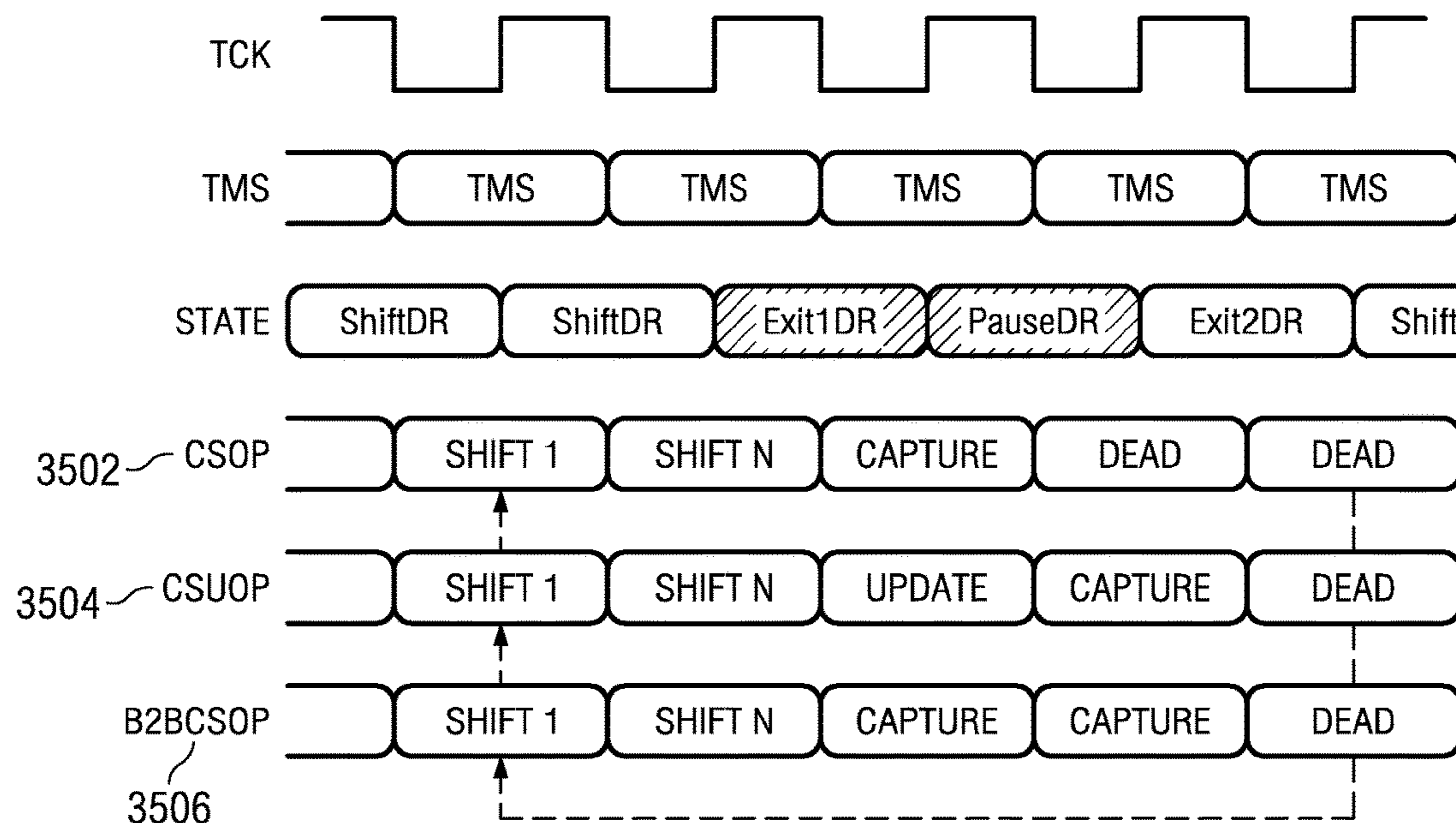
FIG. 35
