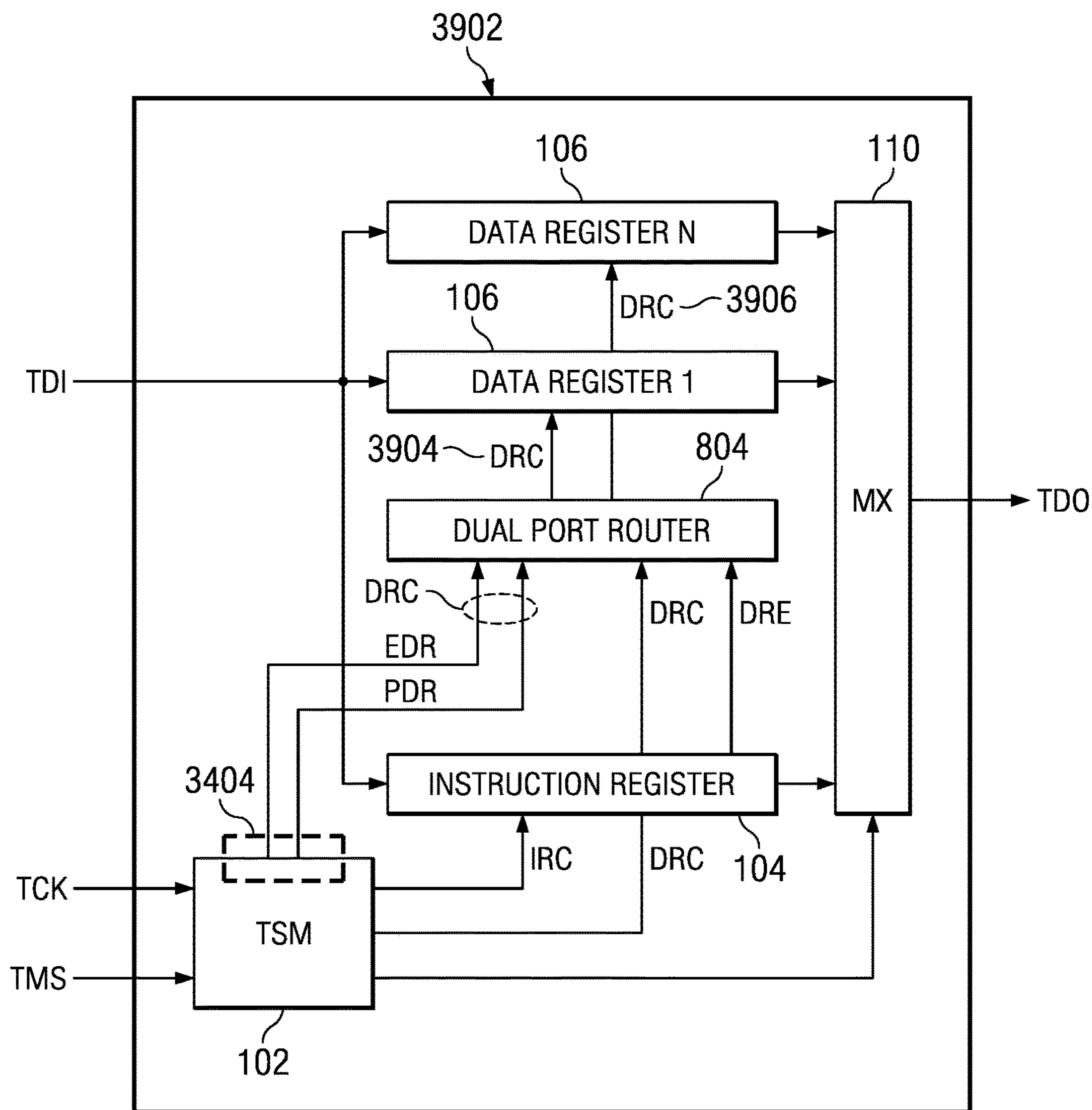
FIG. 39
