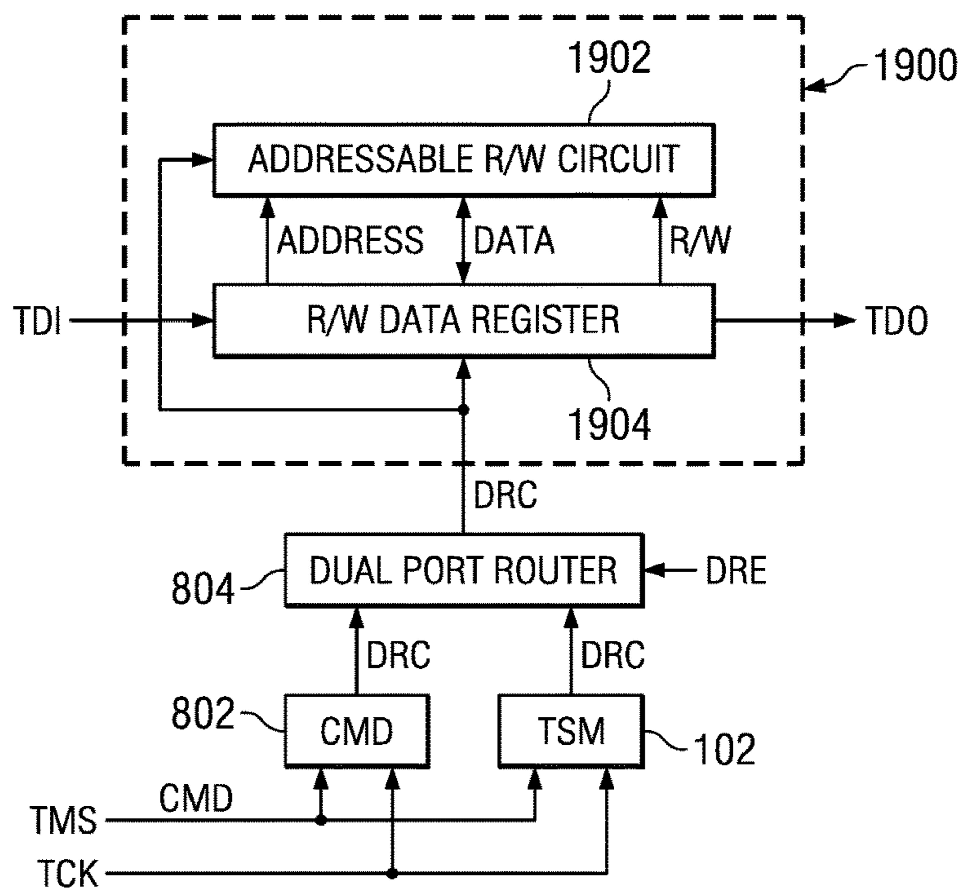
FIG. 19
