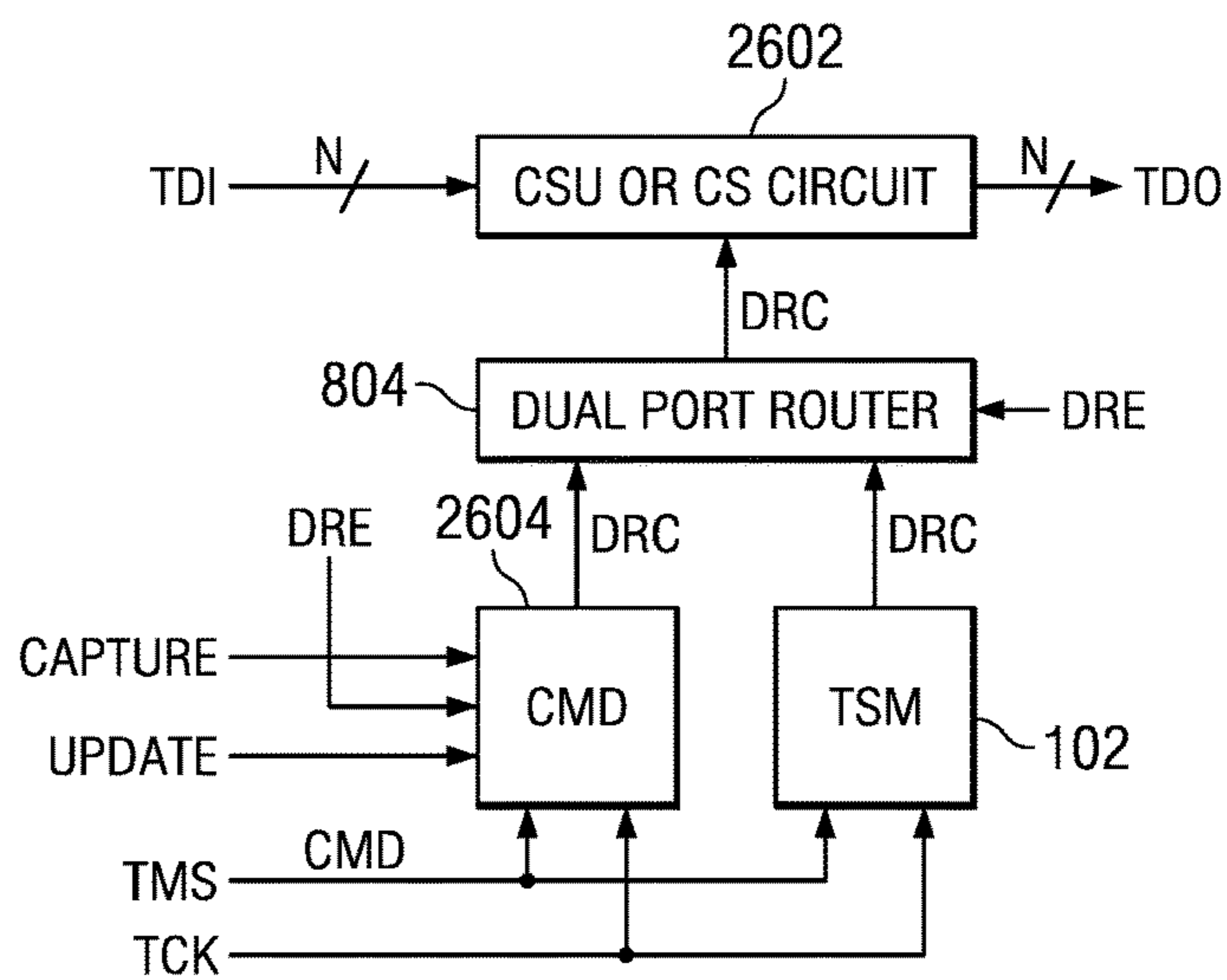
FIG. 26
