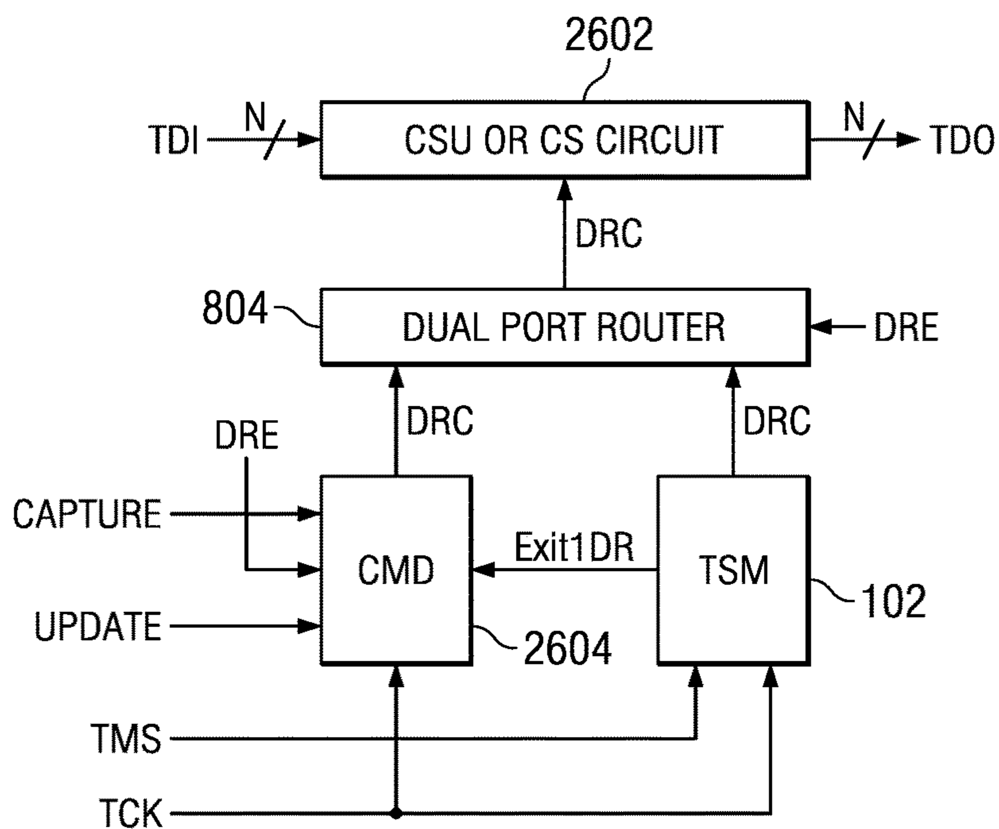
FIG. 33
