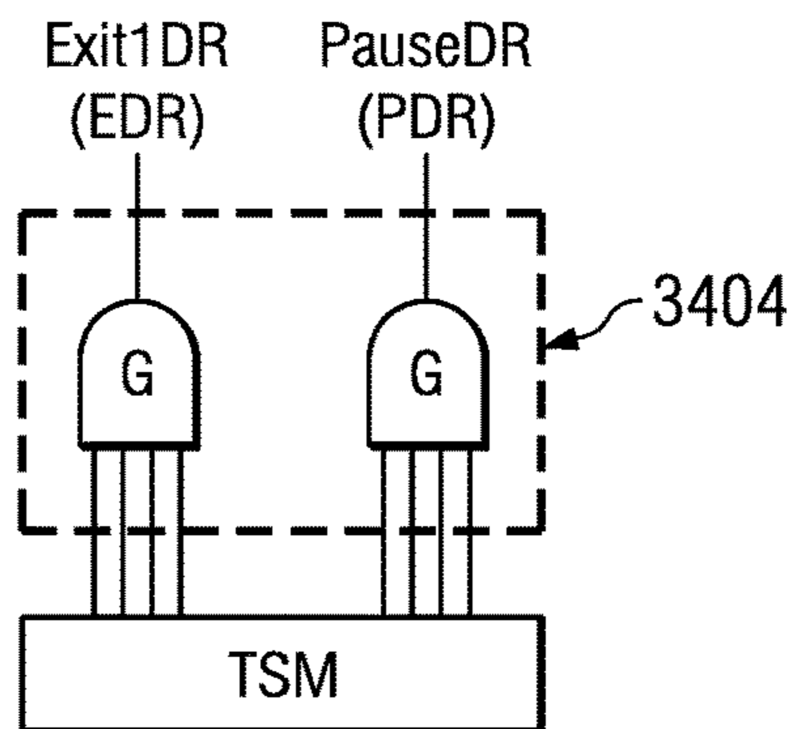
FIG. 34B
