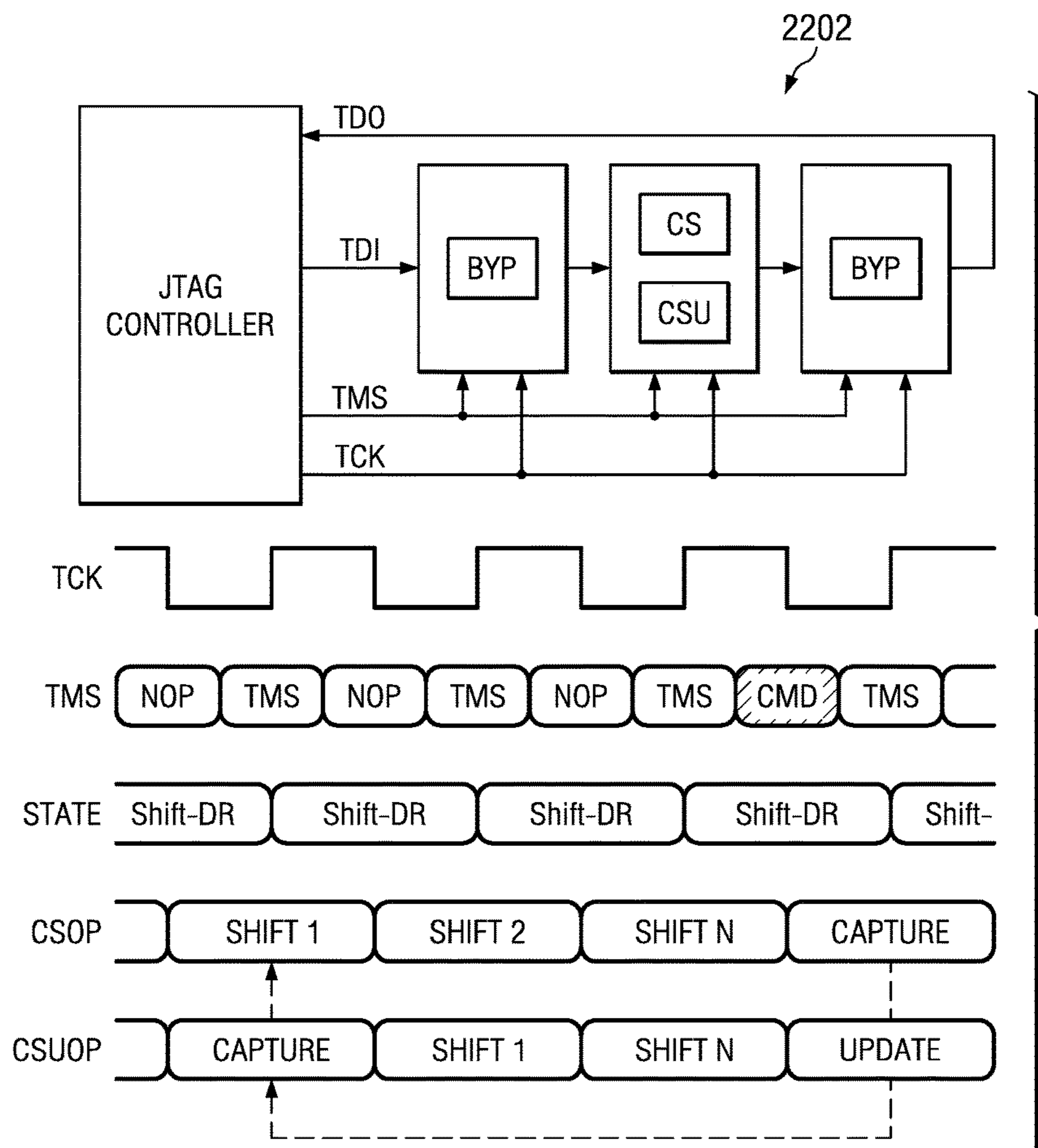
FIG. 22
