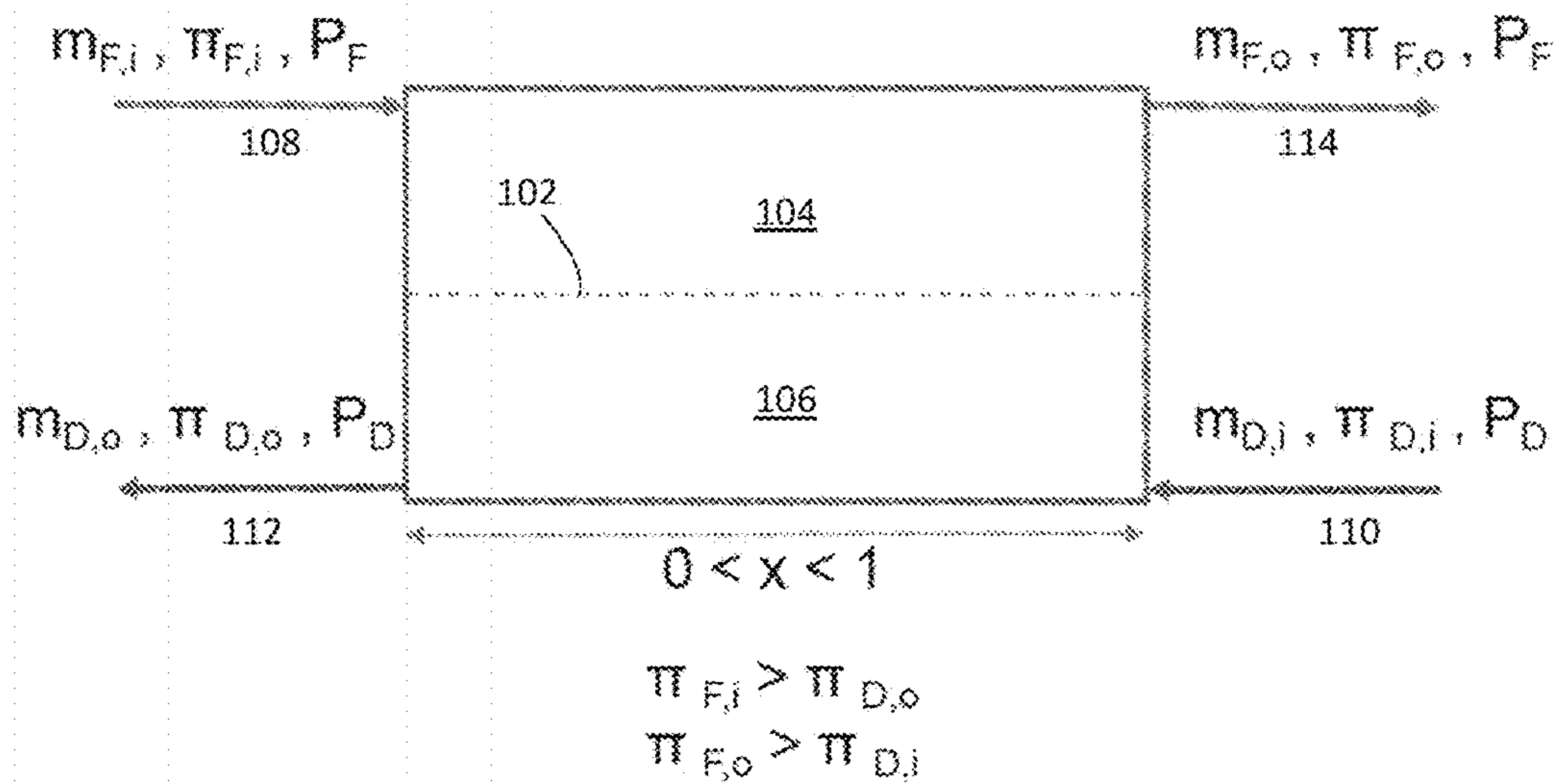
FIG. 4A
