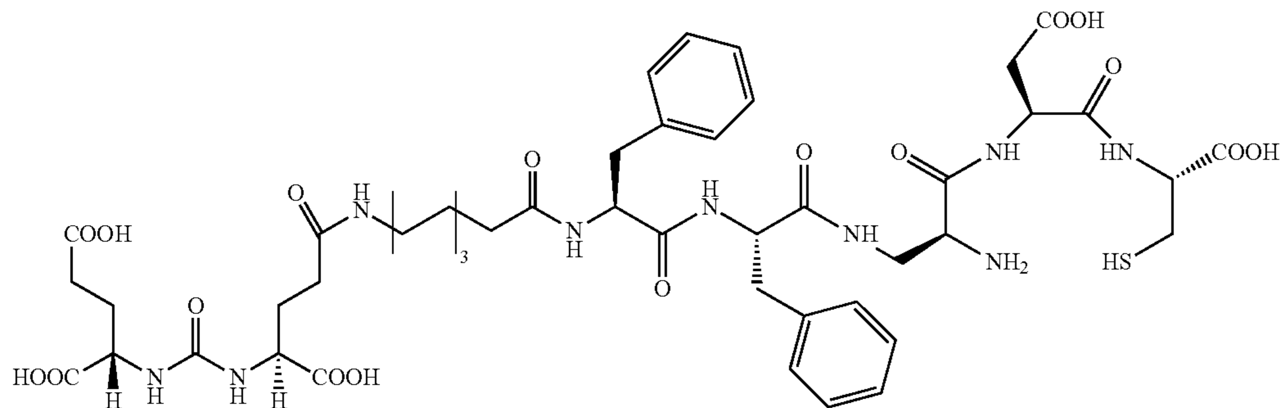
PC01SK28 \text{C}_{47}\text{H}_{65}\text{N}_9\text{O}_{17}\text{S} Mol. Wt.: 1060.13
