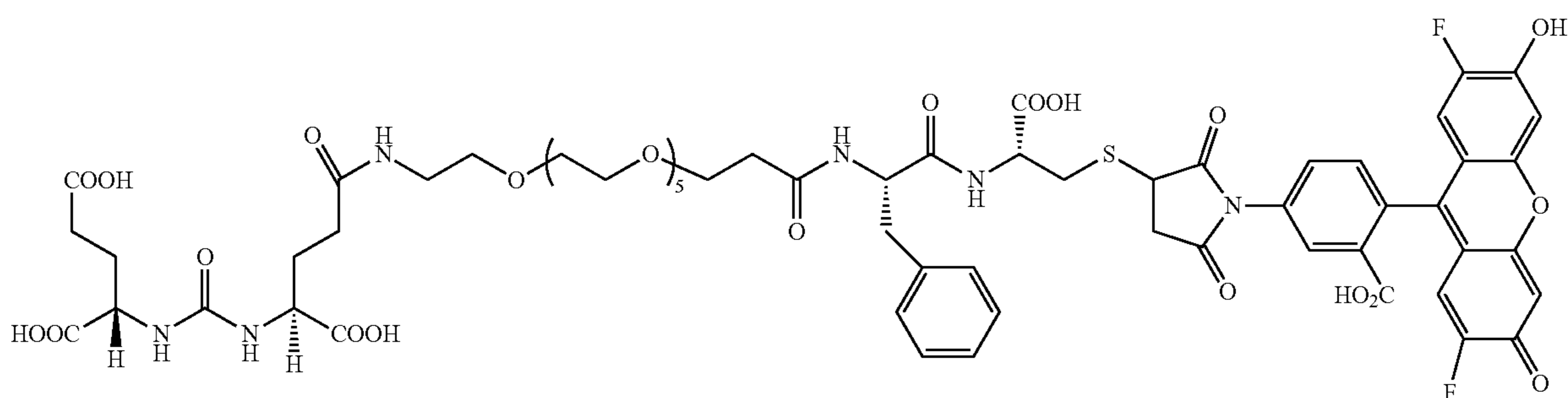
PC01SK56 C_{62}H_{70}F_2N_6O_{25}S Mol. Wt.: 1369.31
