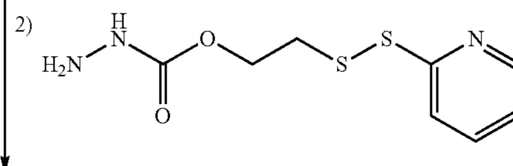
EC0311 C 8 H 11 N 3 O 2 S 2 Mol. Wt.: 245.32
