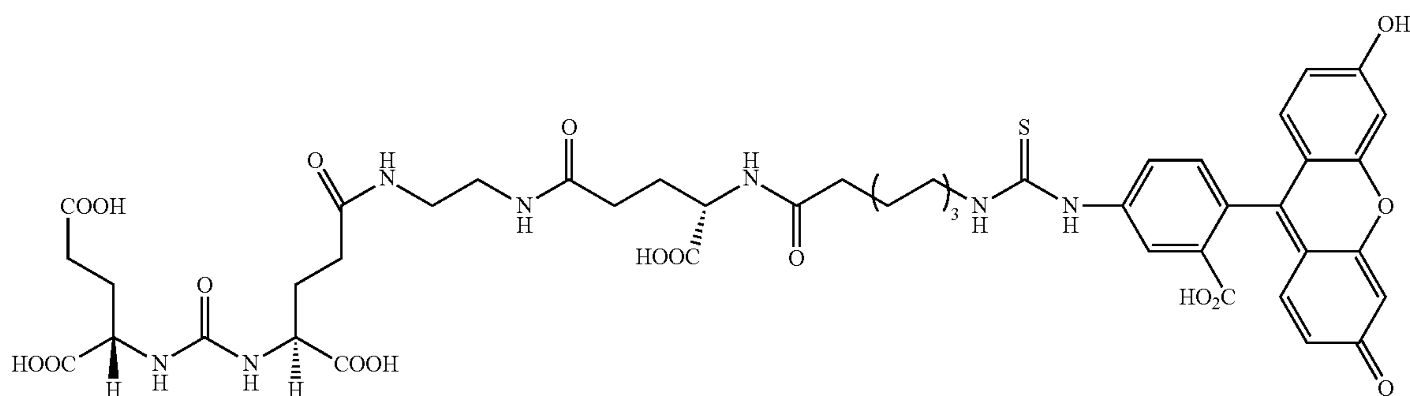
PC01SK64 C 47 H 55 N 7 O 17 S Mol. Wt.: 1022.04
