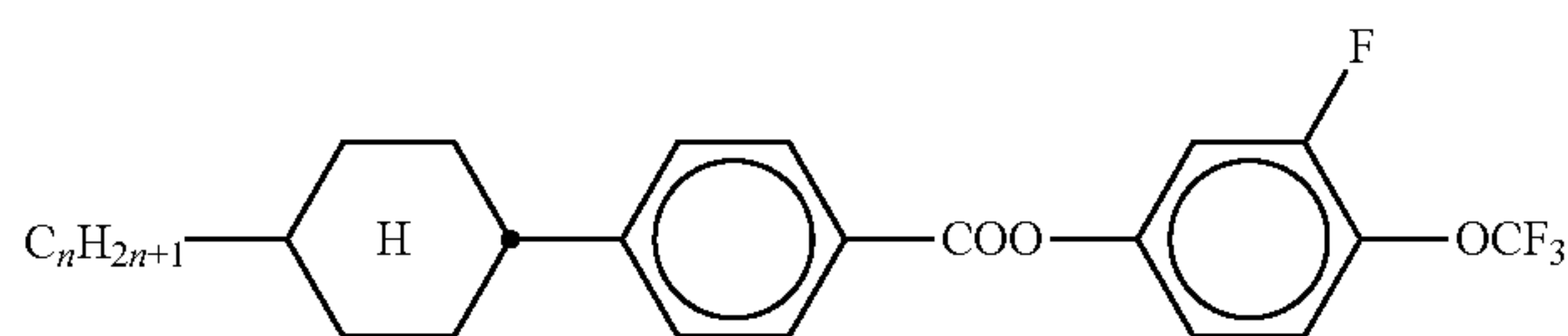
CPZG-n-OT
