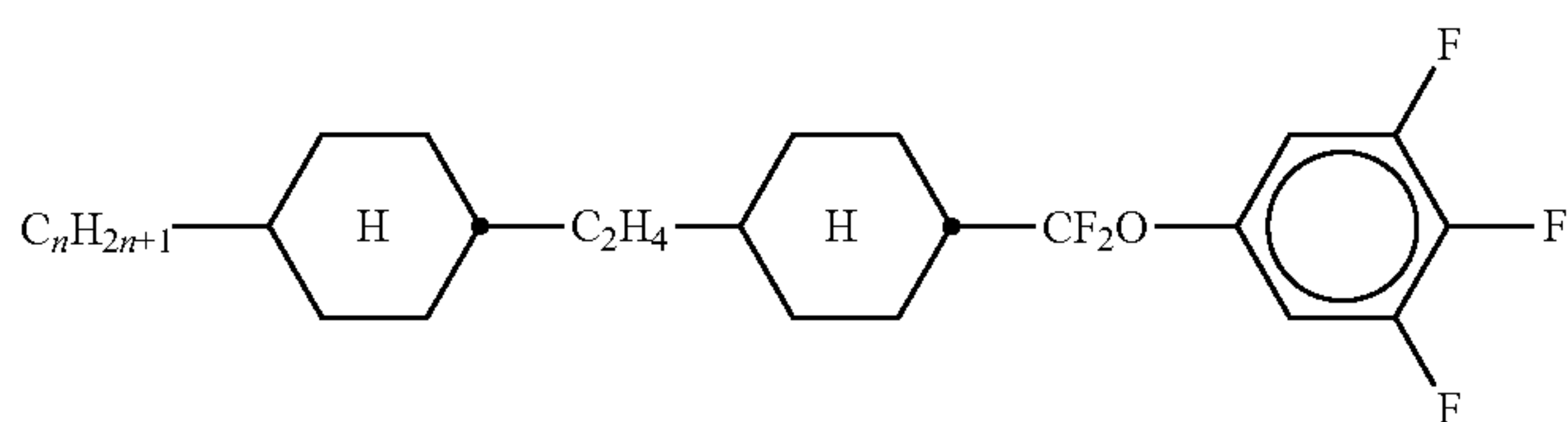
CWCQU-n-F
