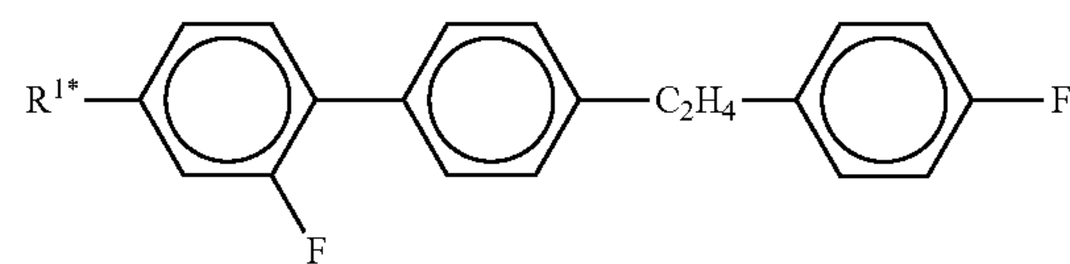
FET-nF
