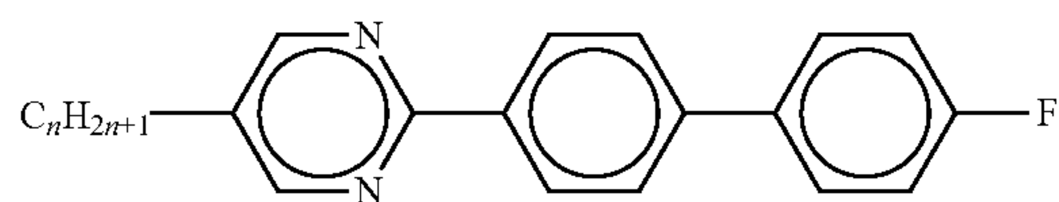
MPP-n-F
