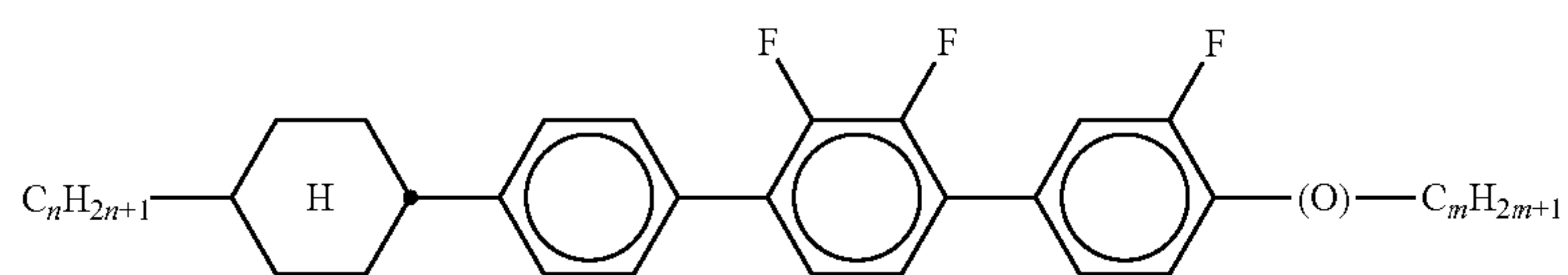
CPYG-n-(O)m
