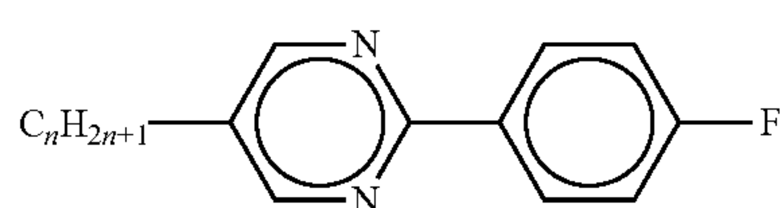
PYP-n-F
