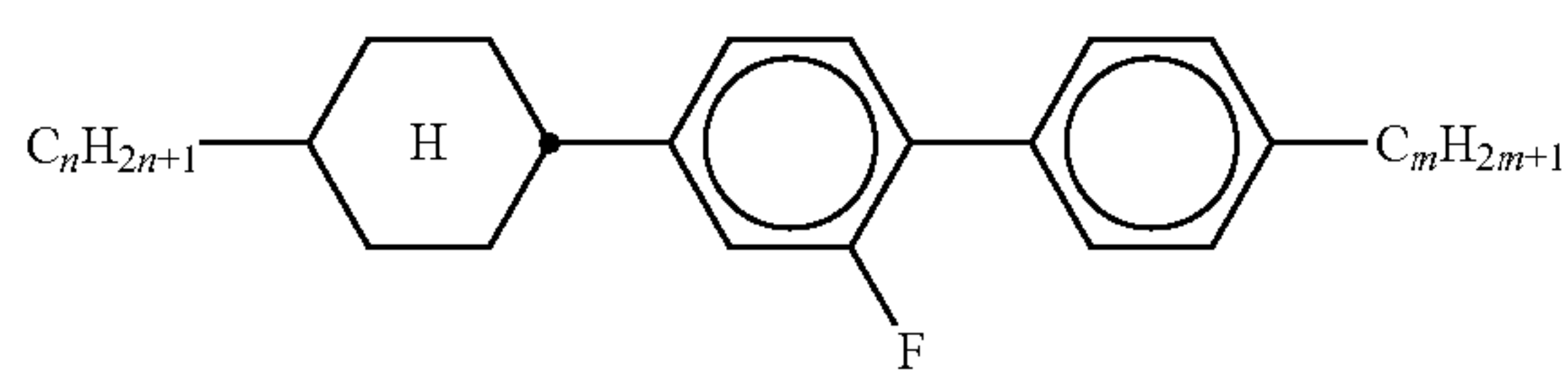
BCH-nmF
