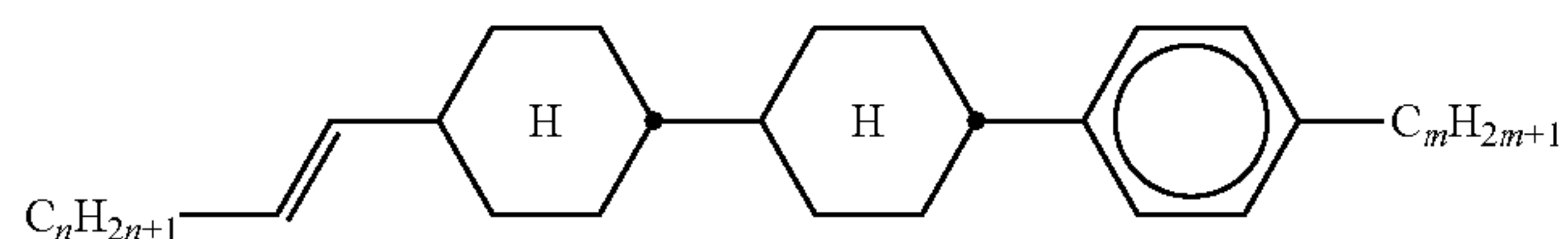
CCP-nV-m
