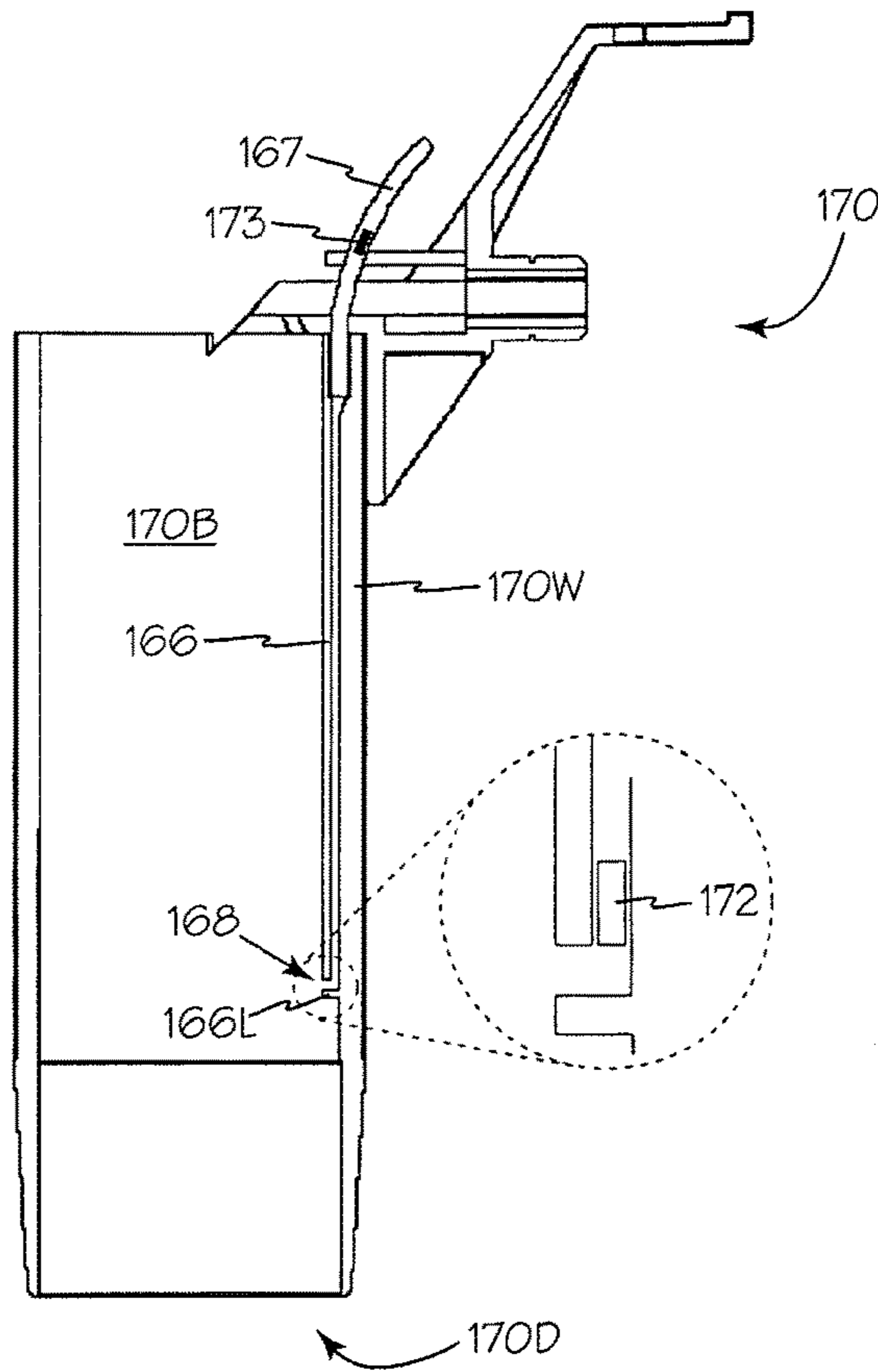
Fig. 31
