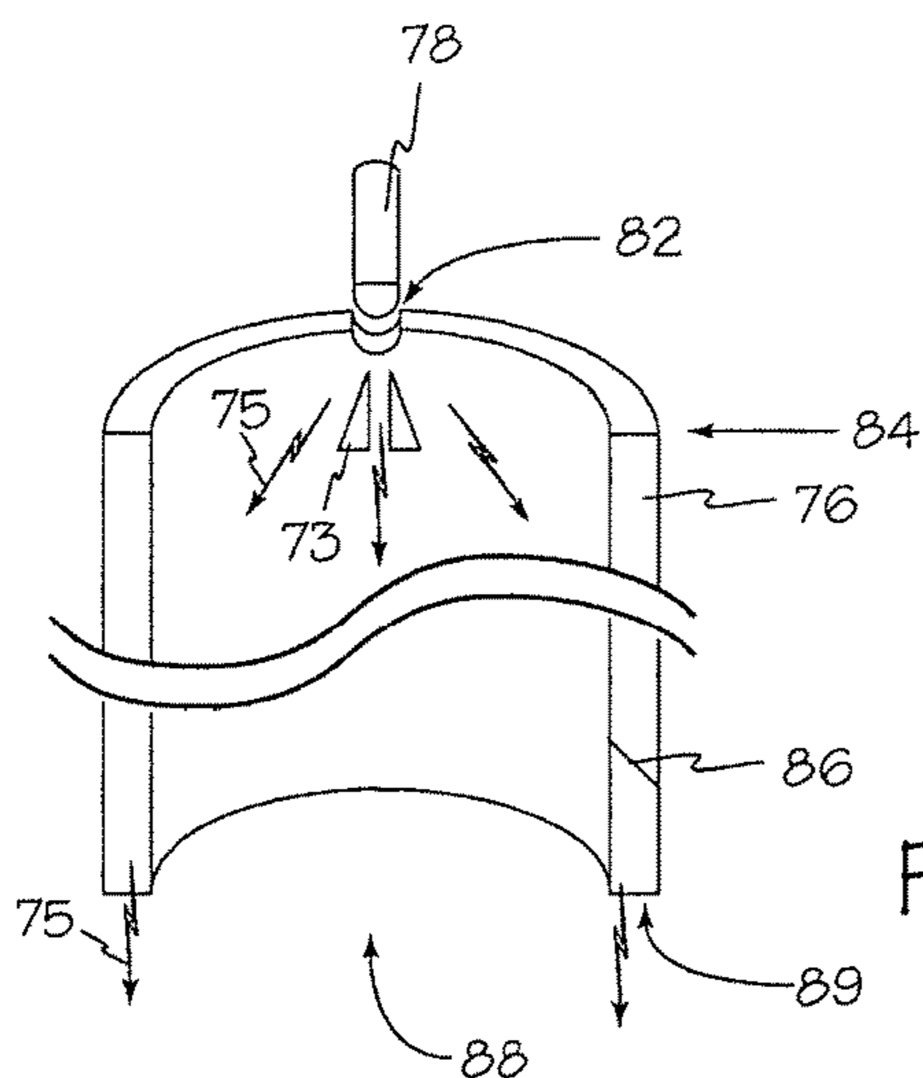
Fig. 11A
