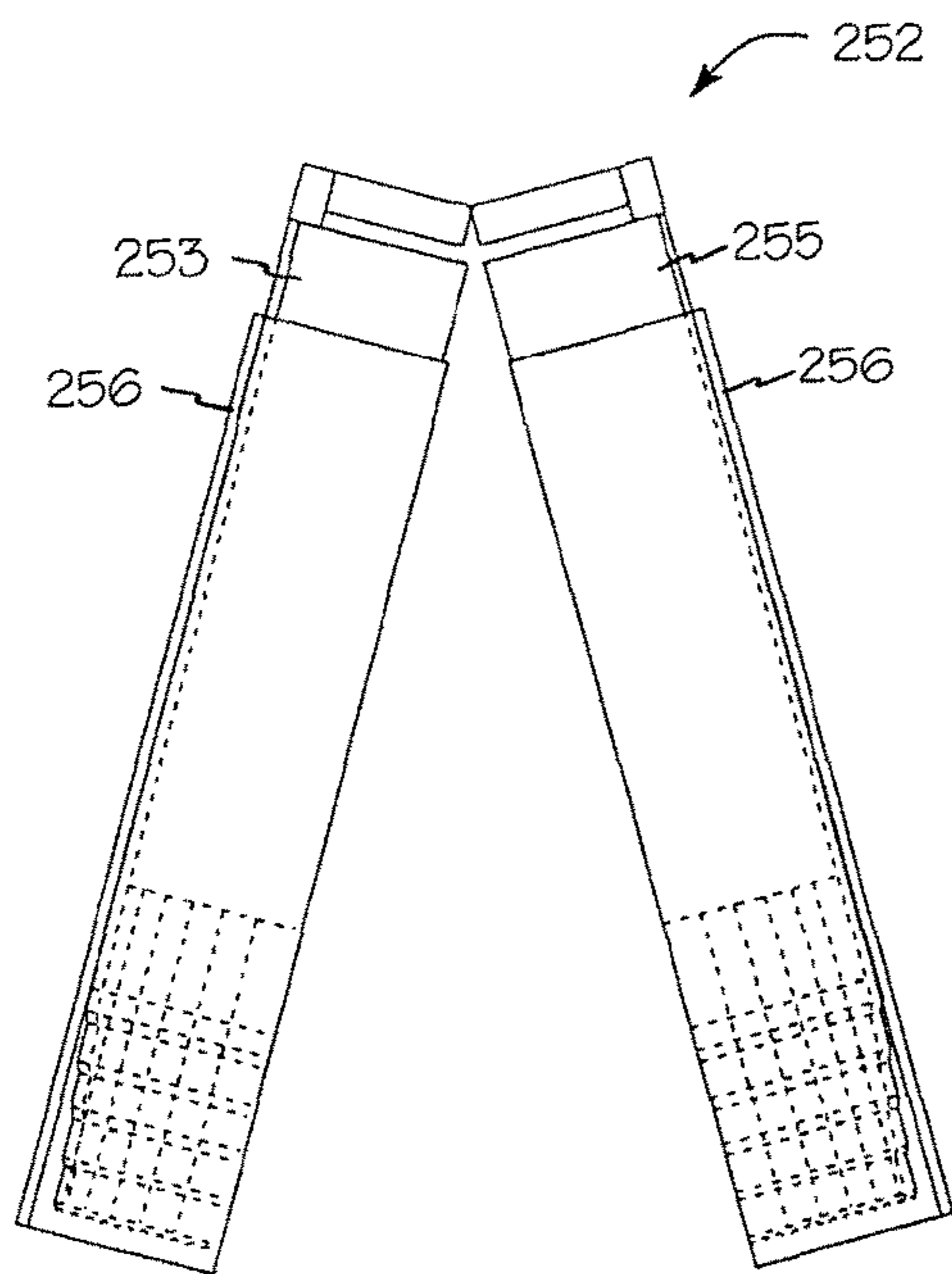
Fig. 46
