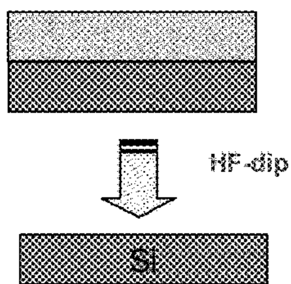
wo/ anneal
