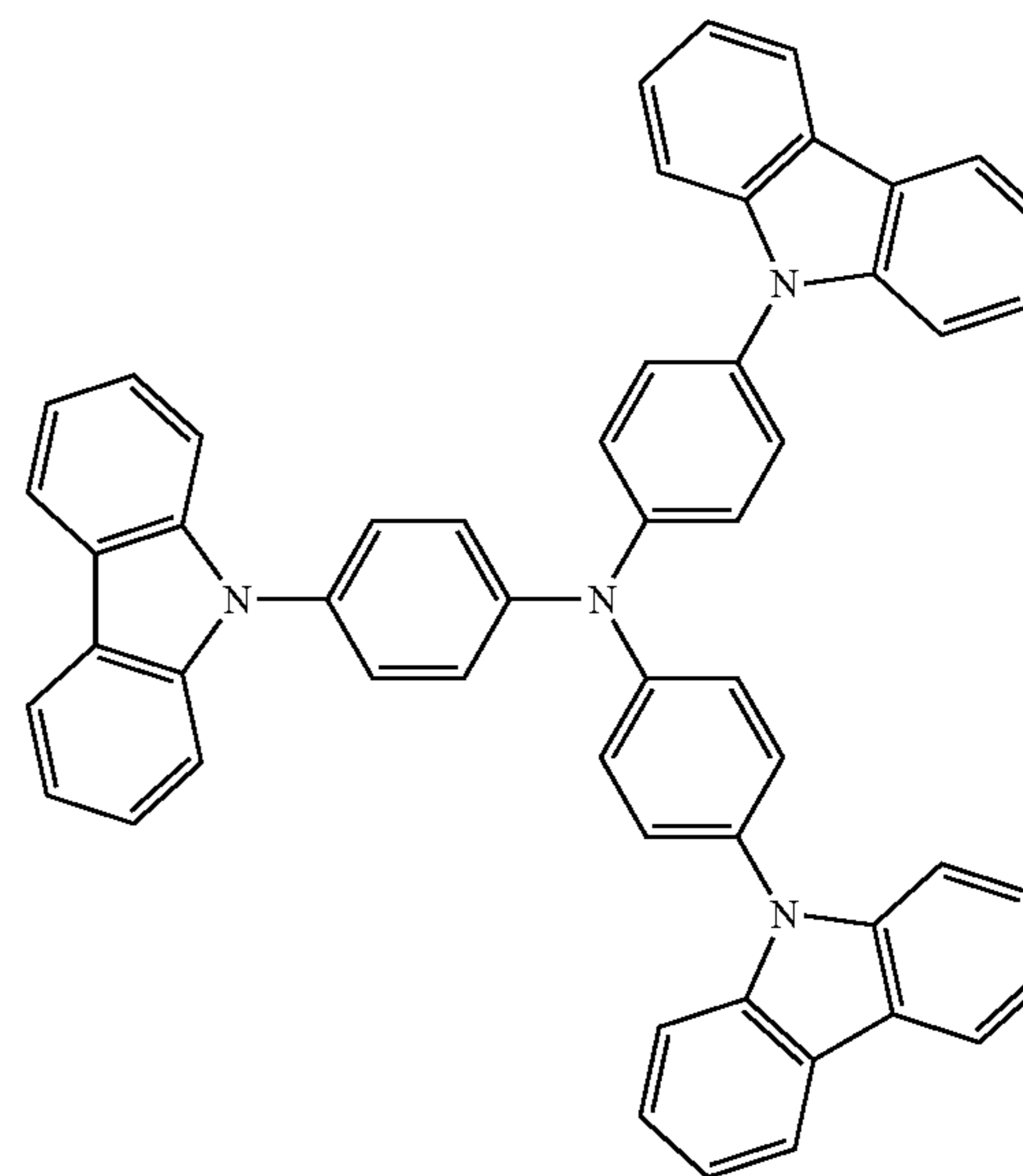
TCTA
