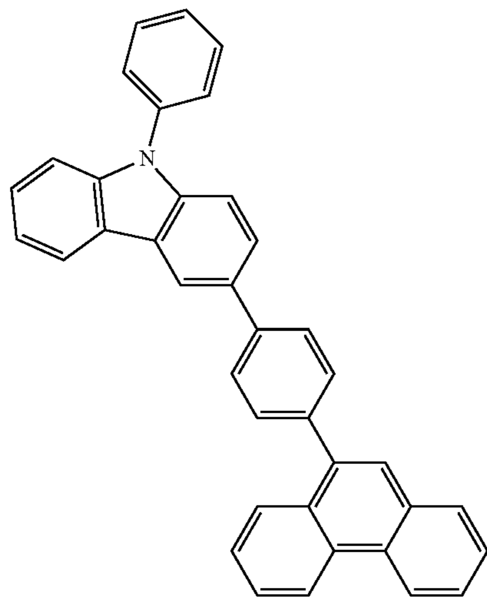
PCPPn
