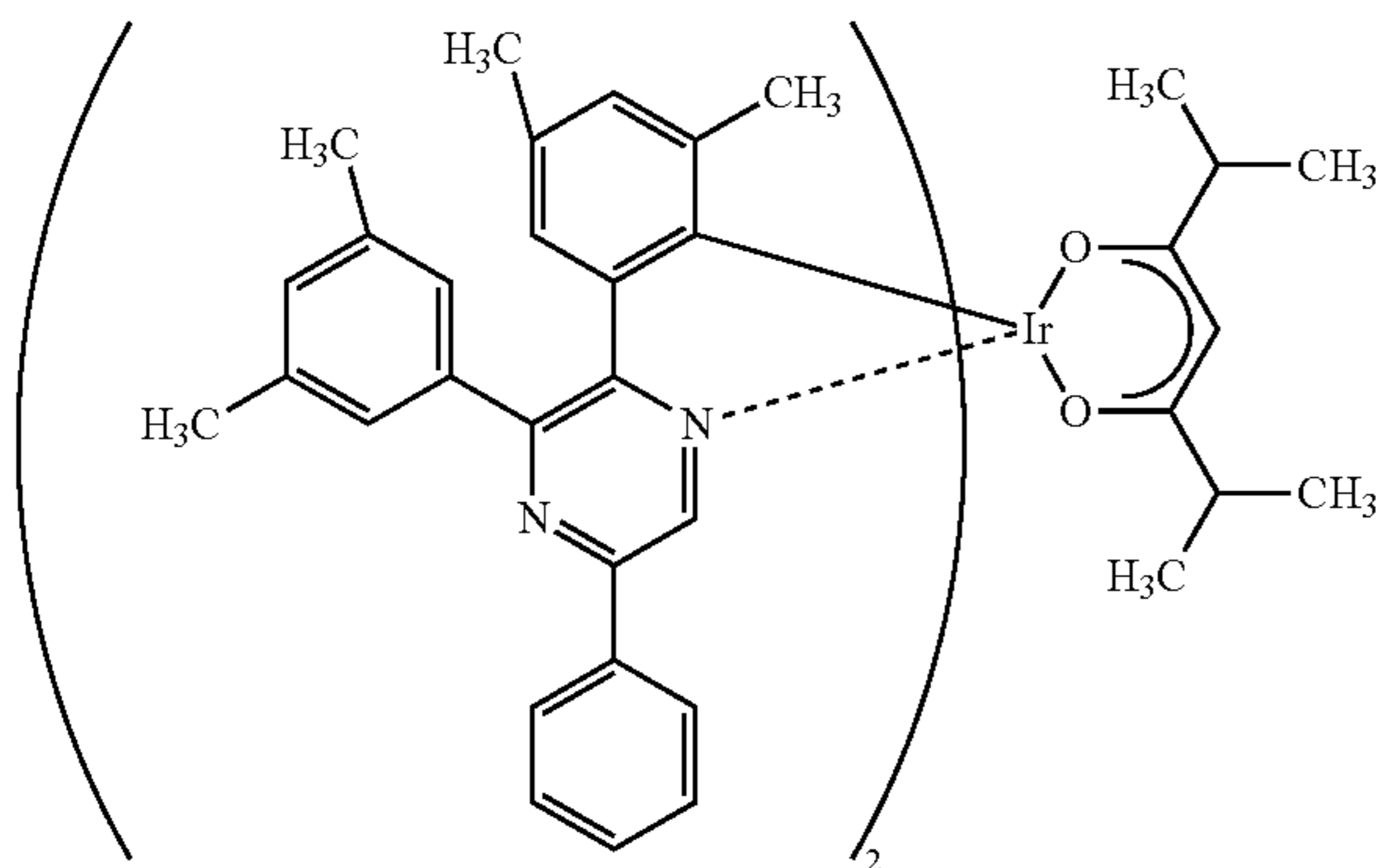
Ir(dmdppr-P) 2 (dibm)
