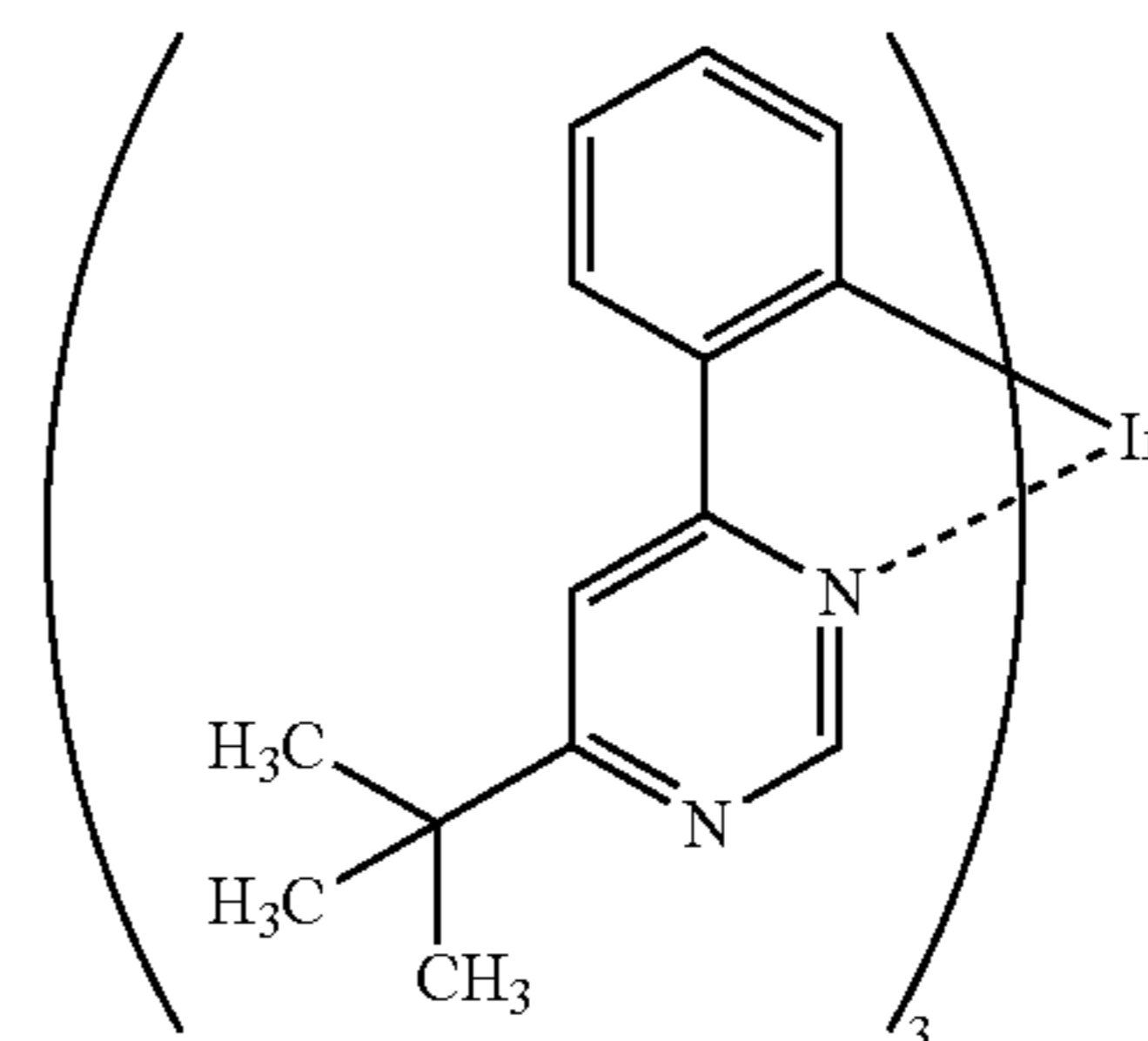
Ir(tBuppm) 3
