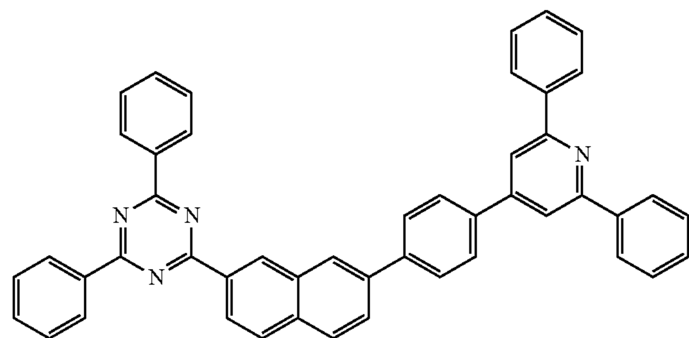
[formula 5-1-5]
