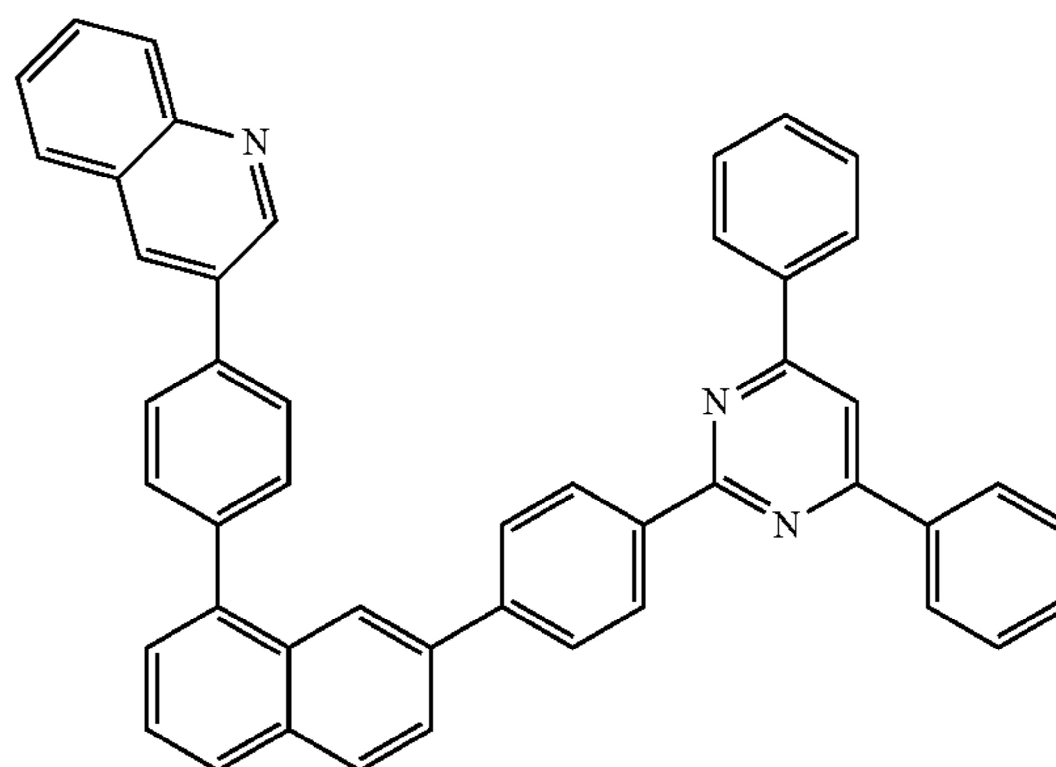
[formula 3-2-6]
