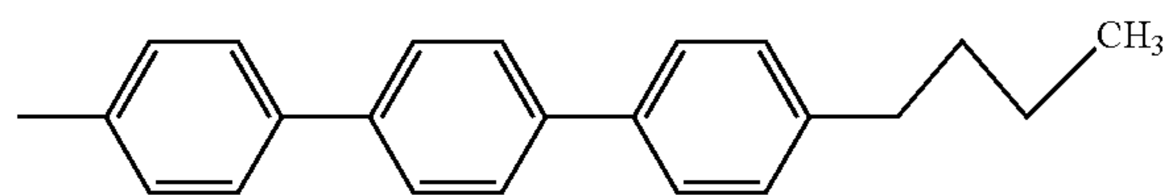
4-butyl-[1,1';4',1'']terphenyl-4-yl
