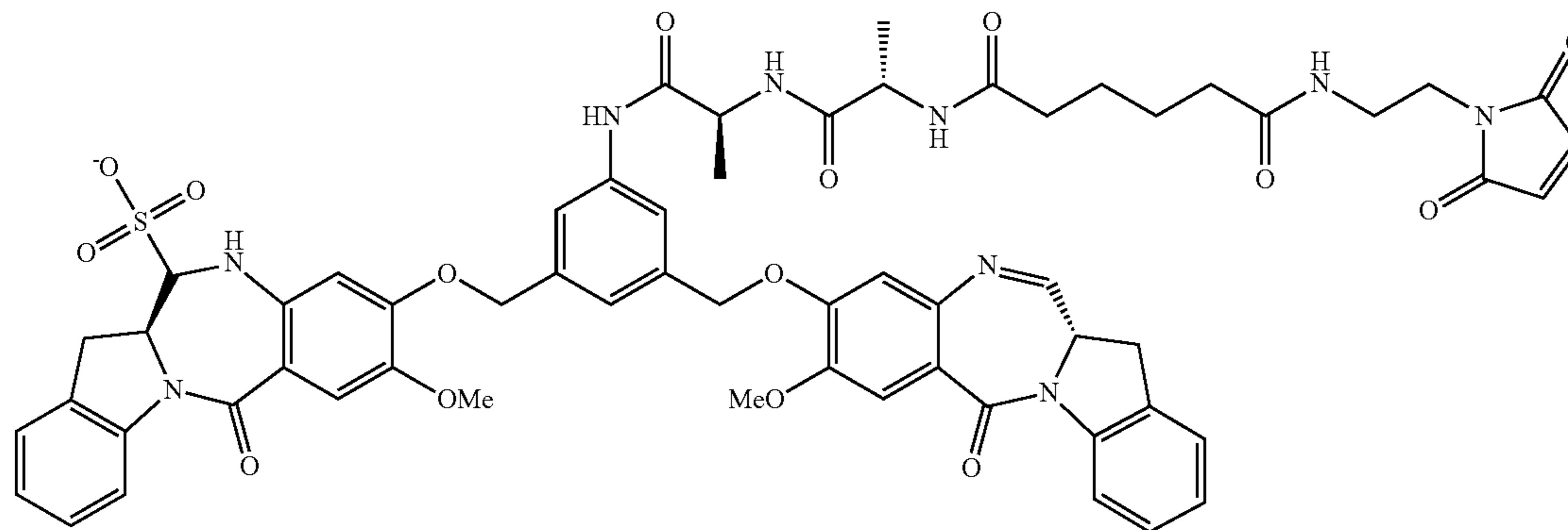
Imine di-sulfo D5
