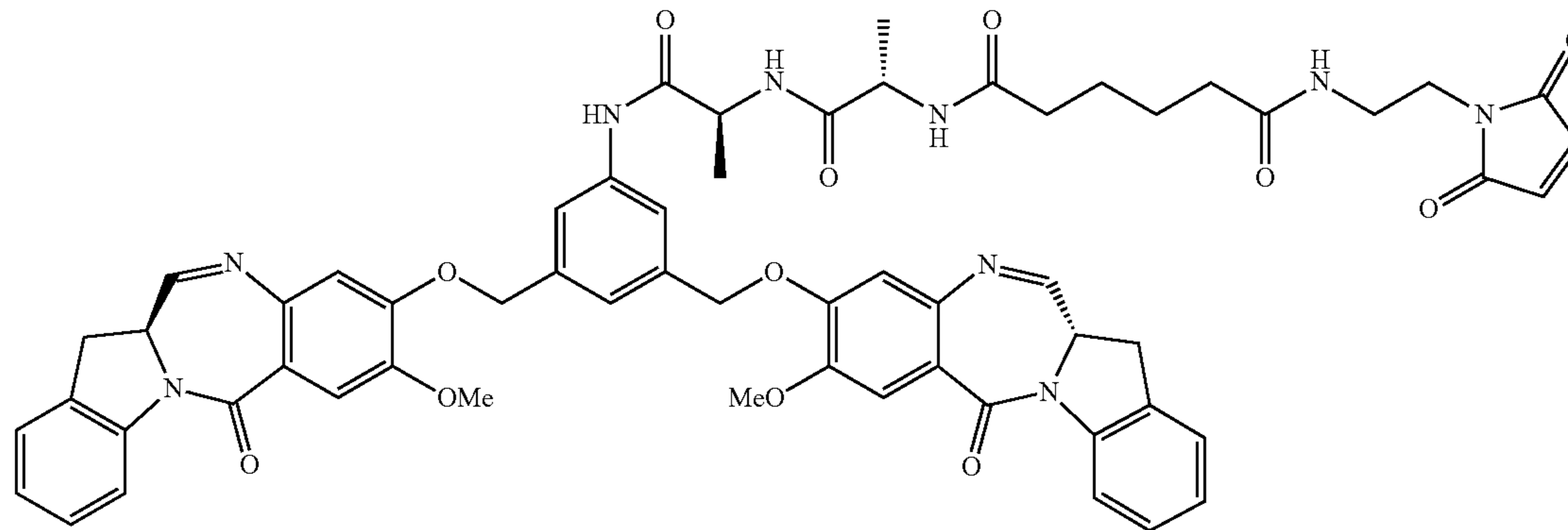
Imine mono-sulfo D5
